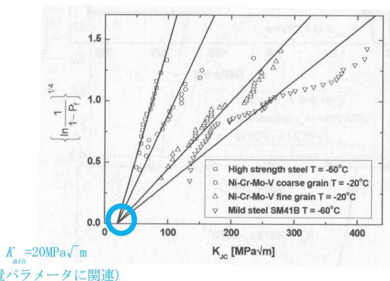
図 4. 2. 12-1 位置母数(固定：最小破壊靱性)の根拠 143
