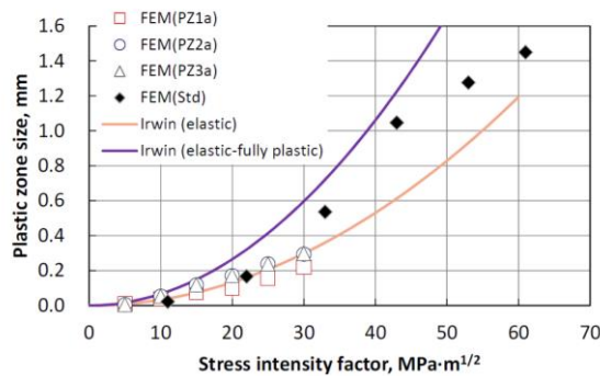
図 4.2.4-1 塑性域寸法の推移の比較 118
