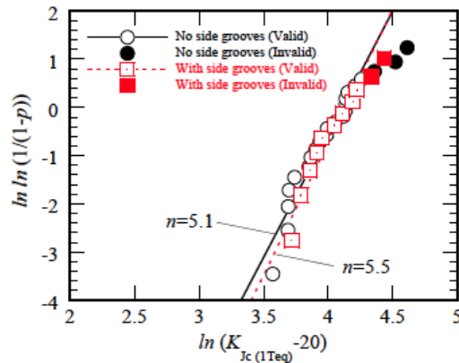
図 4.2.6-1 サイドグループ付き試験片とサイドグループのない試験片による破壊靱性分布（ワイブルプロット）の比較 122
