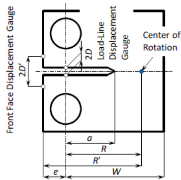
図 4. 2. 8-1 Mini-C(T) の寸法 124
