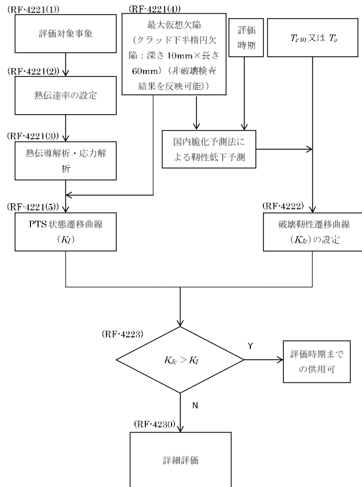
図-RF-4210-1 一般評価の評価手順
