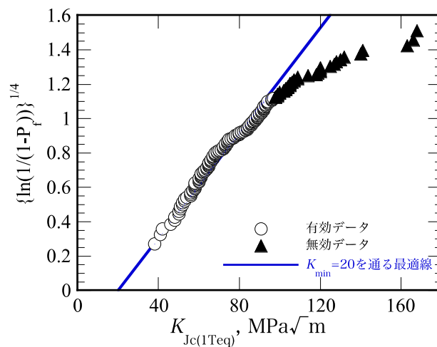
図 4.2.12-2 ロウンドロビンデータに基づく K_{min} の傾向確認 144
