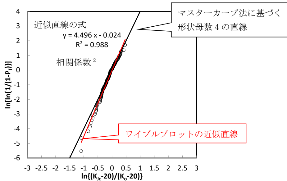
図 4.2.12-4 鍛鋼品の中性子照射後破壊靱性データのワイブルプロット(全材料) 149
