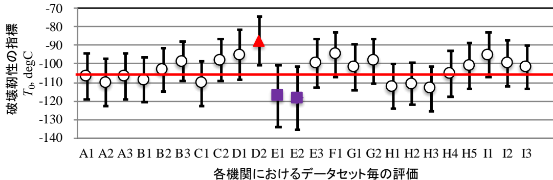
図 4.2.2-5 Mini-C(T)試験片を用いた破壊靱性評価ラウンドロビン試験結果 102
