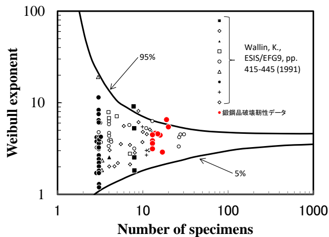
図 4.1.11-3 破壊靱性データのワイブル分布の形状母数 49
