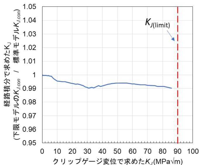
図添付 5-5 経路積分法で求めた K_{J,con} と荷重-CG 変位で求めた K_J の関係 ( \sigma_{ys}=275 MPa)
