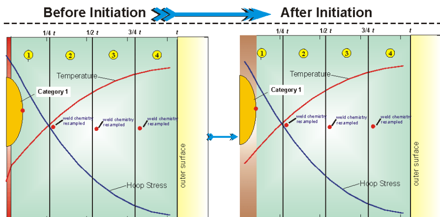
図 4.1.12-1 FAVOR における欠陥の想定例
