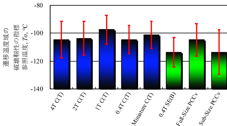
図 4.2.2-1 様々な寸法の未照射材の試験片で取得した破壊靱性データ 93
