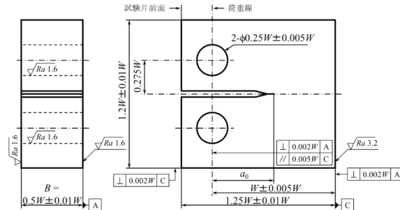
参考図 4. 1. 11-1 タイプ I 試験片の例 (ピンの外径は 0.24W_{-0.005W}^0 とする。)
