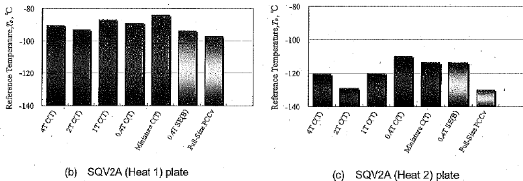
図4.2.2-3 単一温度法(sgl)及び複数試験温度法(mlt)による T_0 の評価結果
