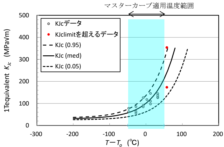
(a) 鍛鋼品 No. 1 (照射量 2.3 \times 10^{19} n/cm 2 , T_0 = -33^\circ\text{C} )
