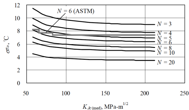
図 4.2.9-1 破壊靱性の中間値 K_{Jc}(\text{med}) と T_0 の標準偏差の関係における破壊靱性確認方法 2016 と ASTM E1921 の比較 137
