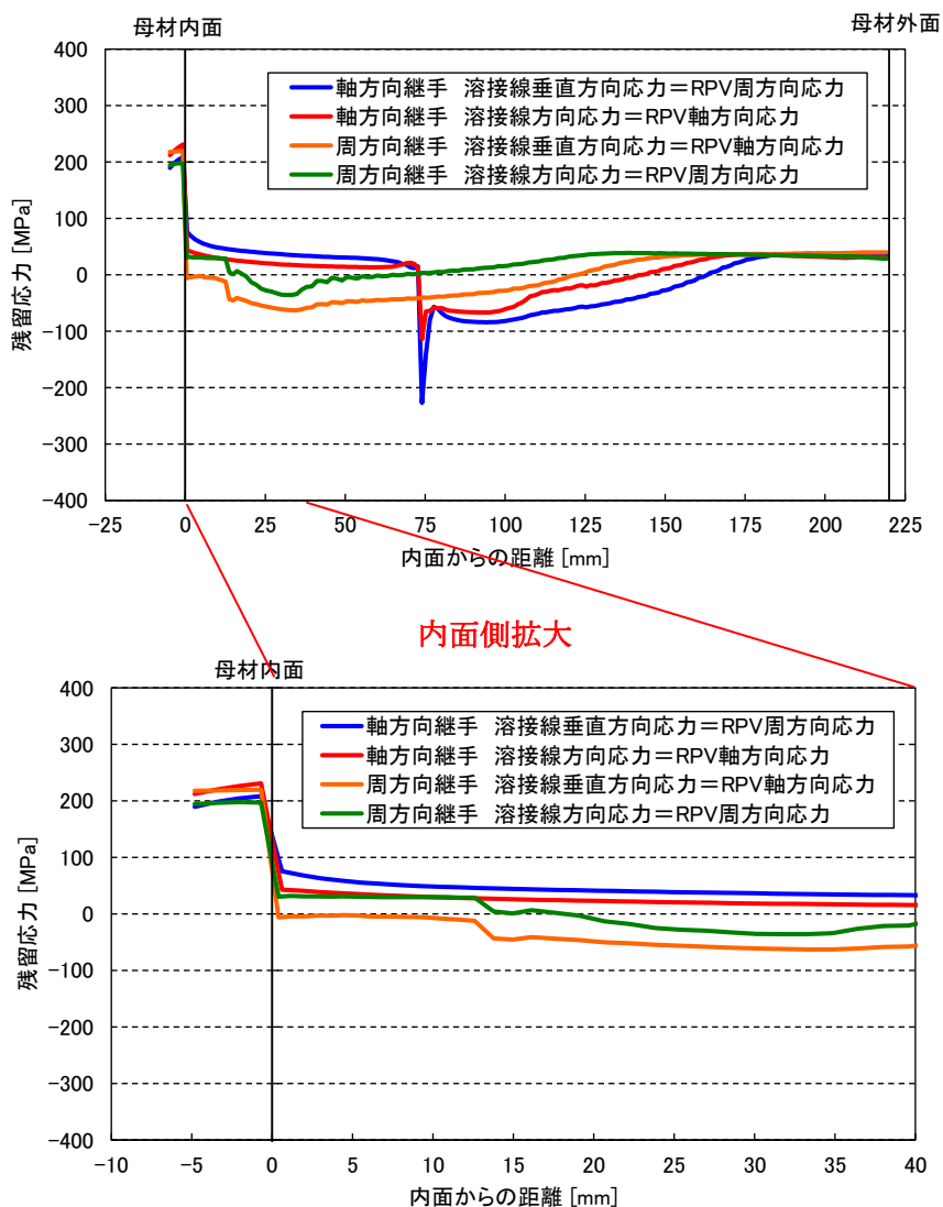
図 4-9-1 軸方向継手と周方向継手の溶接残留応力の比較(運転条件負荷後、室温) 13
