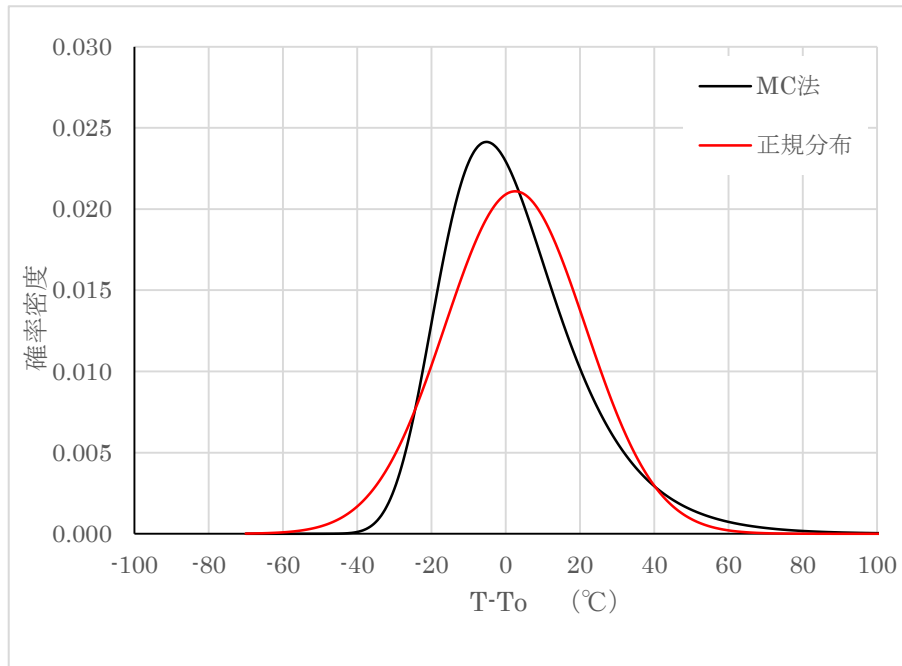
図 4. 1. 11-4 T-To のマスターカーブ法及び置き換えた正規分布の確率密度分布 ( K_{Jc}=100\text{MPa}\sqrt{\text{m}} 、中央値 =-0.22^\circ\text{C} 、 \mu=2.56^\circ\text{C} 、 \sigma=18.91^\circ\text{C} )
