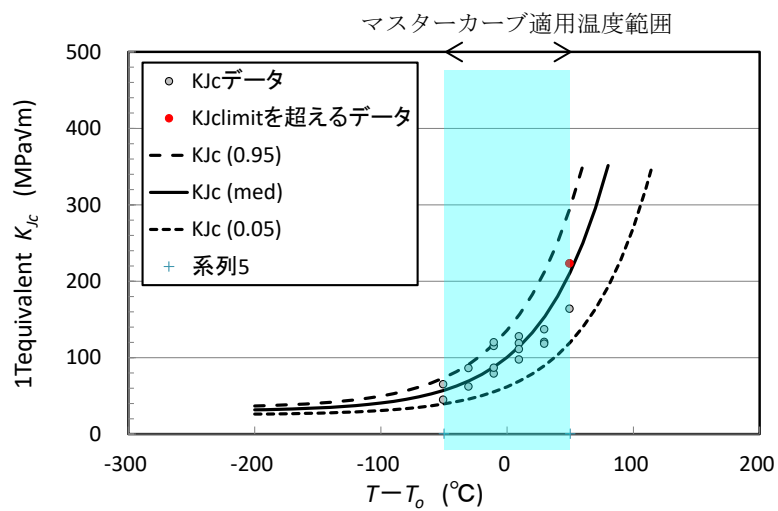
(b) 鍛鋼品 No. 2 (照射量 2.6 \times 10^{19} n/cm 2 , T_0 = -49^\circ\text{C} )
