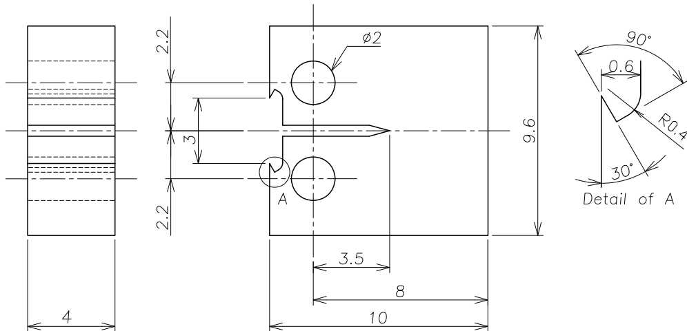
図 4. 2. 3-2 クリップゲージ取付用切欠き部の詳細を記載した Mini-C(T) 試験片形状 115
