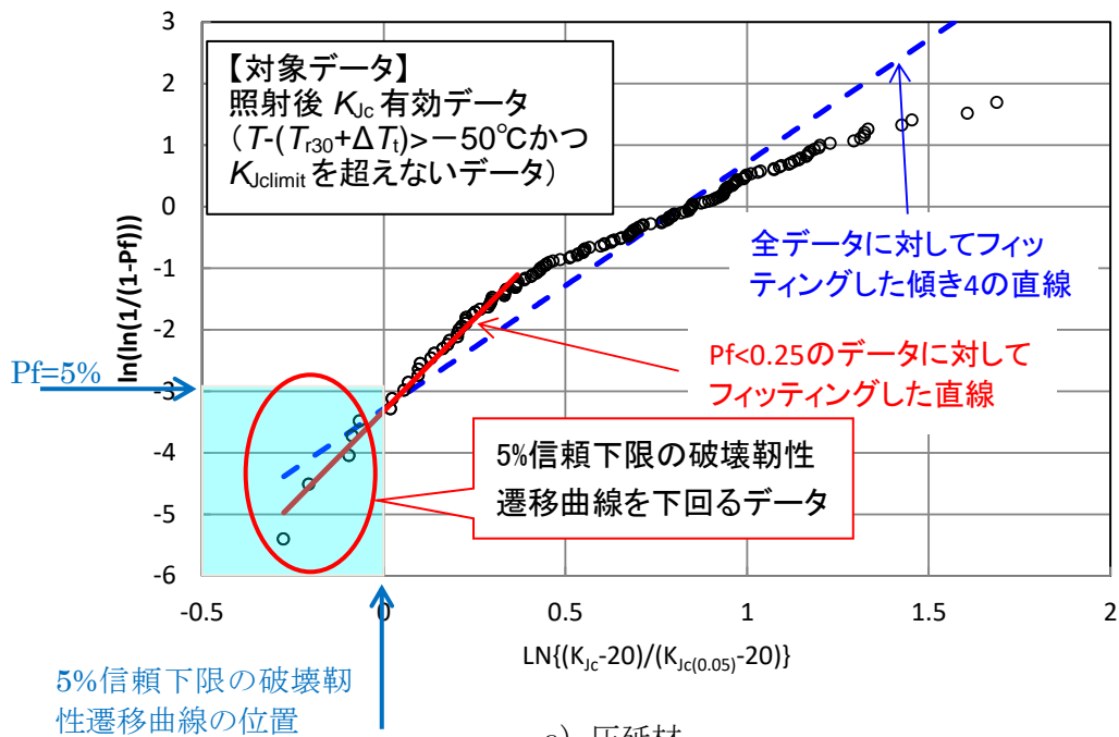
図 4.1.11-6(1/2) 中性子照射後破壊靭性データ（圧延材、鍛鋼品、溶接金属）のワイブルプロット 65
