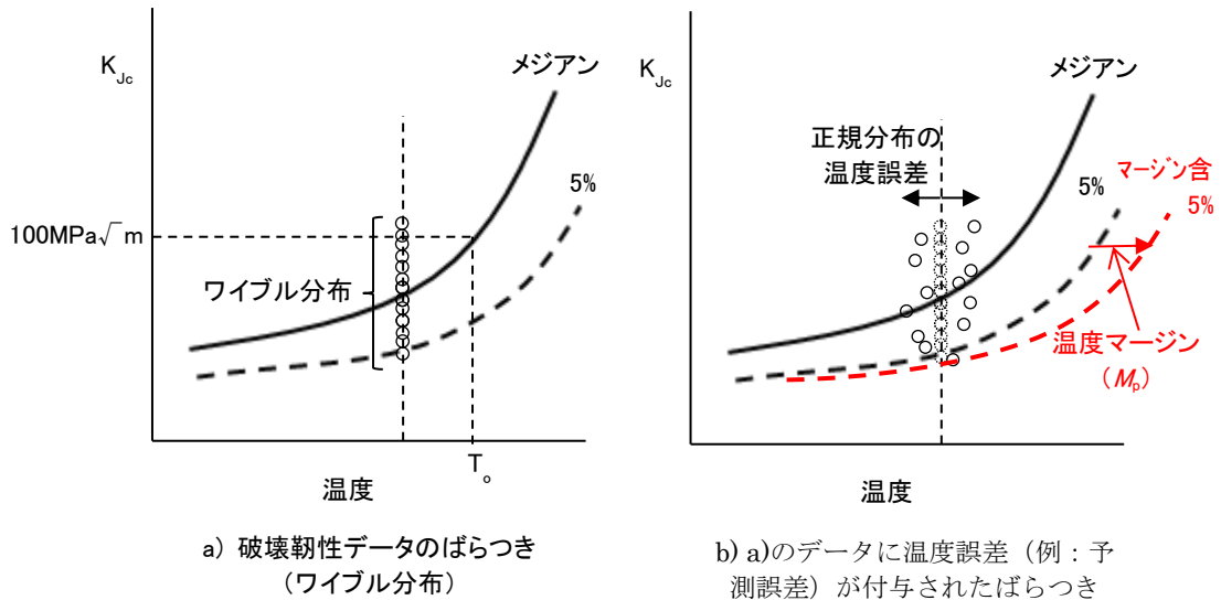
図 4.1.11-5 脆化予測による予測誤差を考慮したマージン ( M_k ) 63
