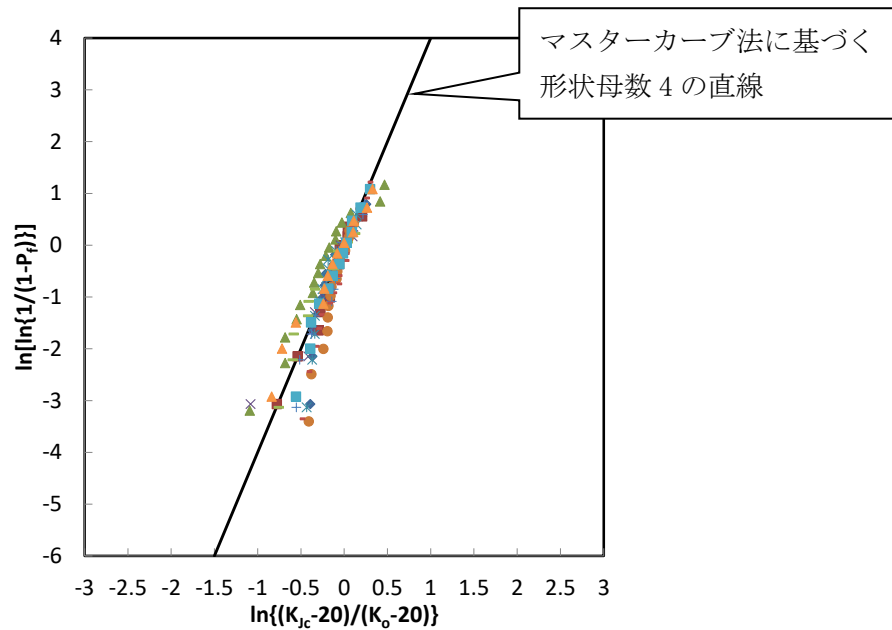
図 4. 2. 12-3 鍛鋼品の中性子照射後破壊靱性データのワイブルプロット (材料毎) 148
