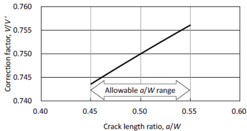
図 4. 2. 8-2 a/W と V/V' の関係 125
