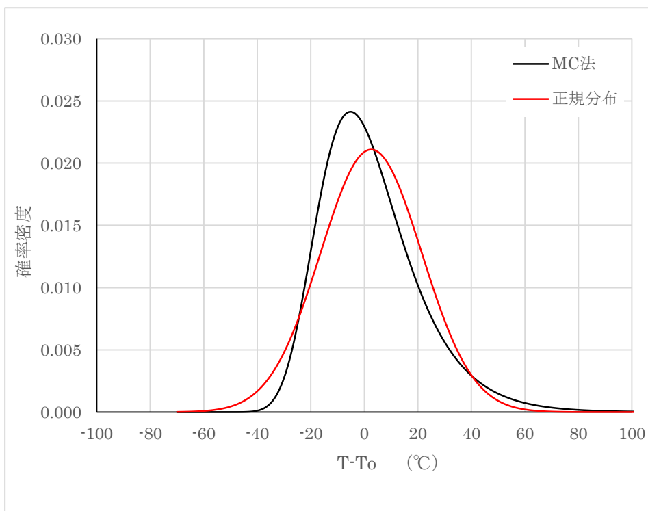
図添付 4-1 T-To のマスターカーブ法及び置き換えた正規分布の確率密度分布 ( K_{Jc}=100\text{MPa}\sqrt{\text{m}} 、中央値 =-0.22^\circ\text{C} 、 \mu=2.56^\circ\text{C} 、 \sigma=18.91^\circ\text{C} )
