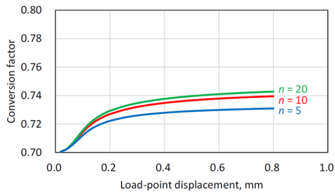
図 4.2.8-4 解析的に得られた換算定数の推移 128
