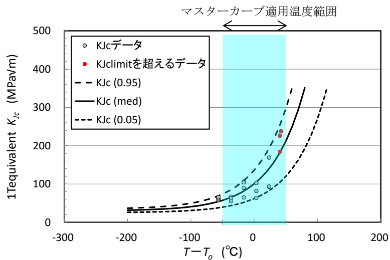
(i) 鍛鋼品 No. 9 (照射量 5.3 \times 10^{19} n/cm 2 , T_0 = -24^\circ\text{C} )
