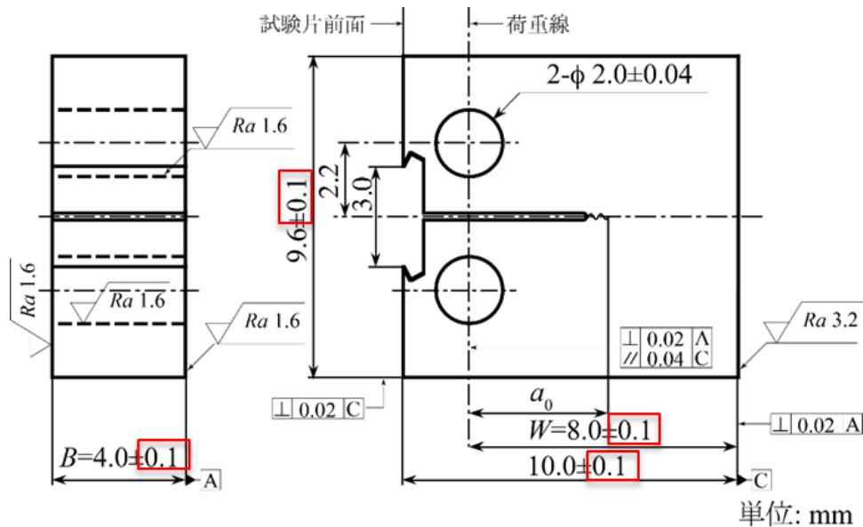
図 4.2.3-1 Mini-C(T)試験片の寸法及び形状 112
