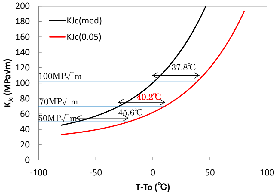
図 4.1.11-9 マスターカーブの K_{Jc(\text{med})} と K_{Jc(0.05)} の温度差 71
