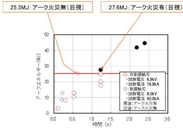
図 5-1 M/C 試験結果
