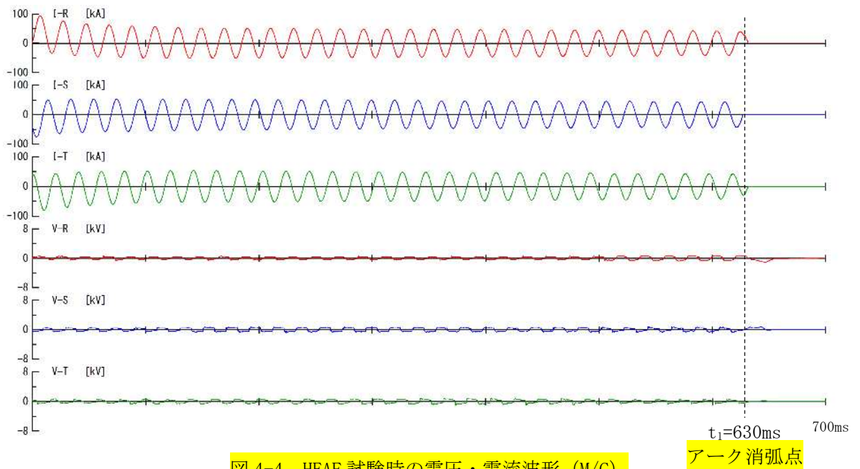
図 4-4 HEAF 試験時の電圧・電流波形 (M/C)
