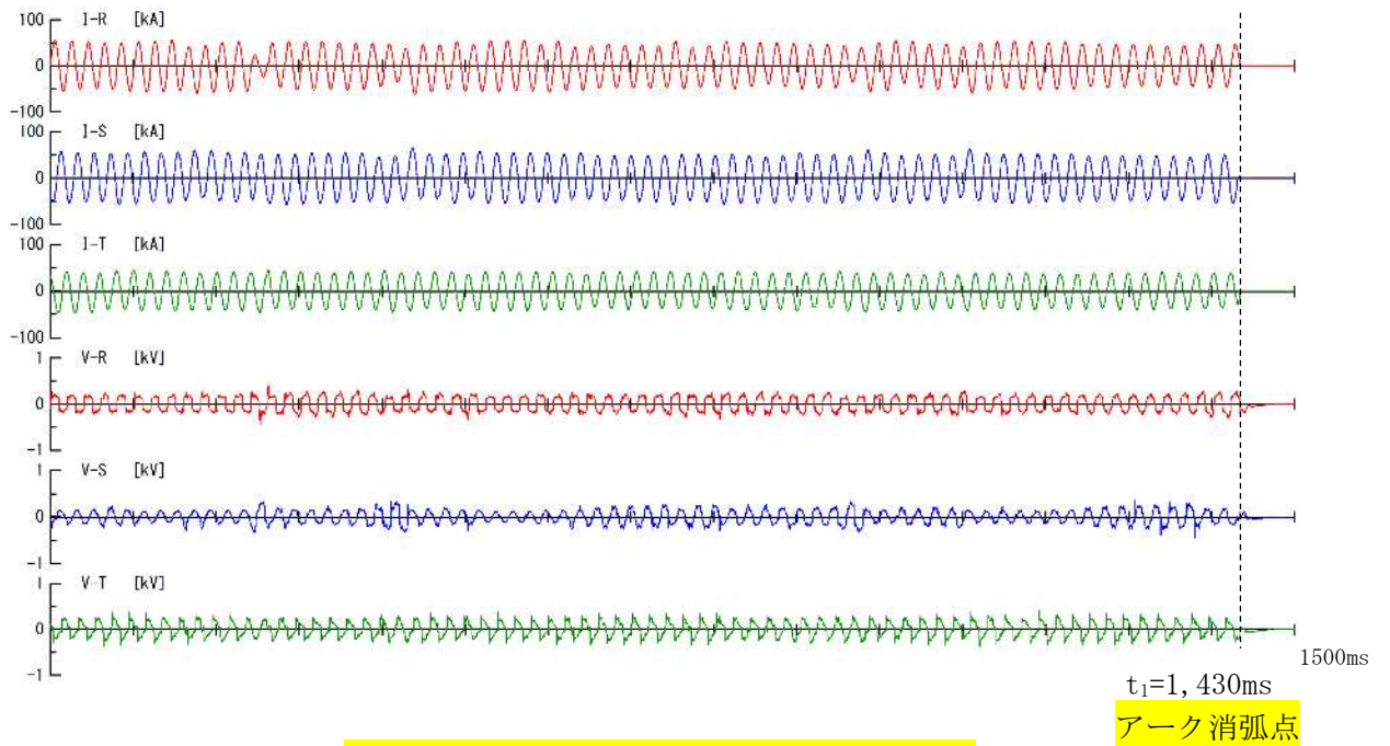
図 4-5 HEAF 試験時の電圧・電流波形 (P/C)
