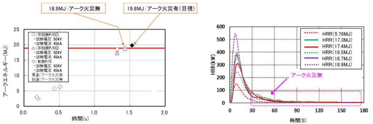
図 5-2 P/C 試験結果
