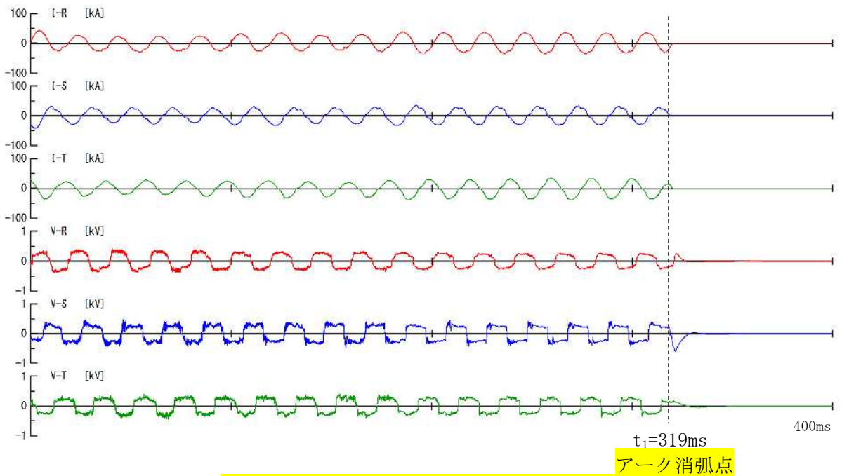
図 4-6 HEAF 試験時の電圧・電流波形 (MCC)
