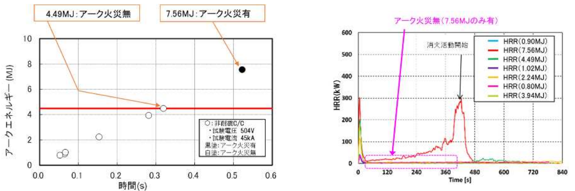
図 5-3 MCC 試験結果
