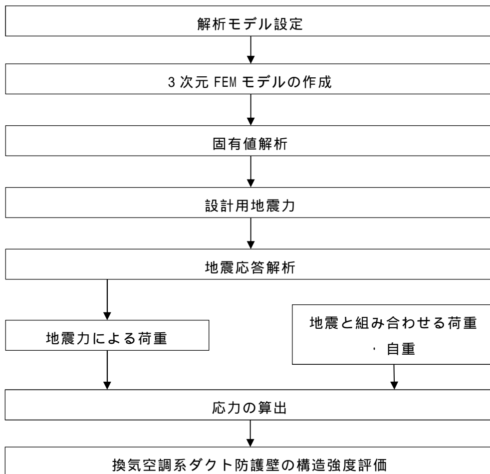
図2-2 換気空調系ダクト防護壁 (No.9) の耐震評価フロー
