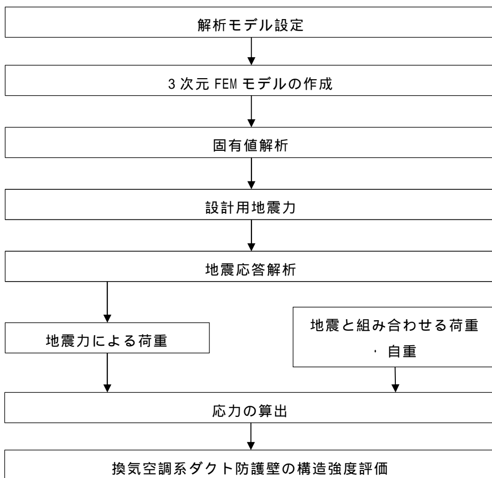
図2-2 換気空調系ダクト防護壁の耐震評価フロー
