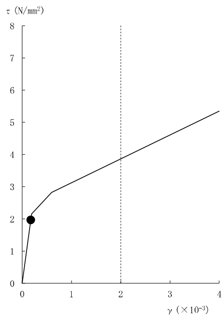
(NS 方向, S s -2, ケース 5, 1F)
