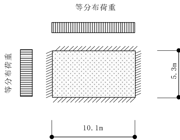
(d) 床スラブ② (四辺固定版)
