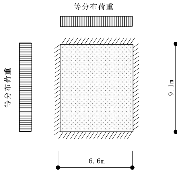
(c) 床スラブ① (四辺固定版)
