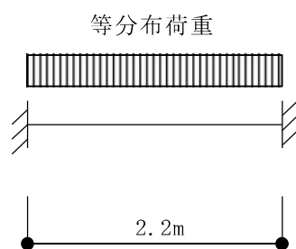
(a) 天井スラブ①（両端固定はり）
