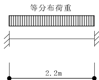
(a) 天井スラブ①（両端固定はり）
