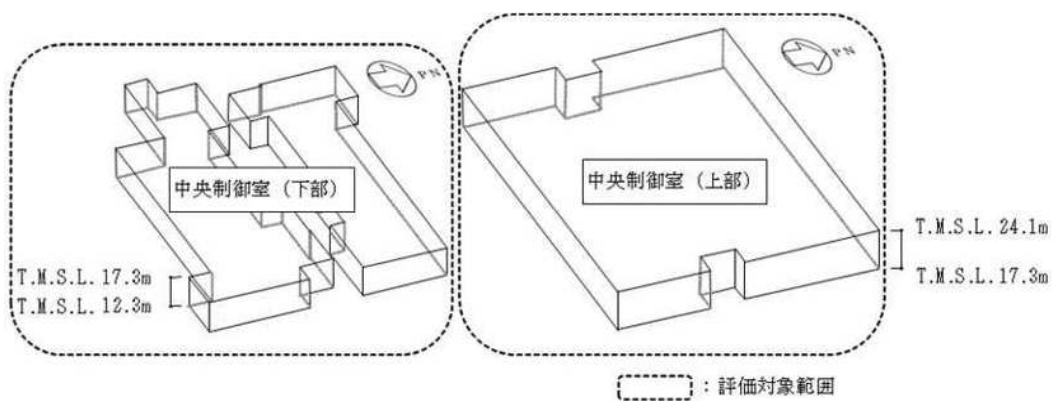
(b) 中央制御室バウンダリの概要
