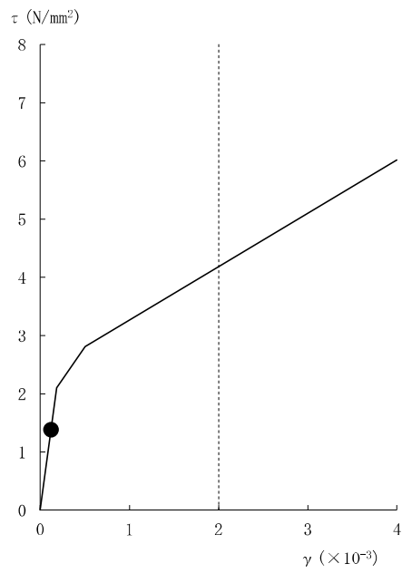
(EW 方向, S s -1, ケース 5, 2F)
