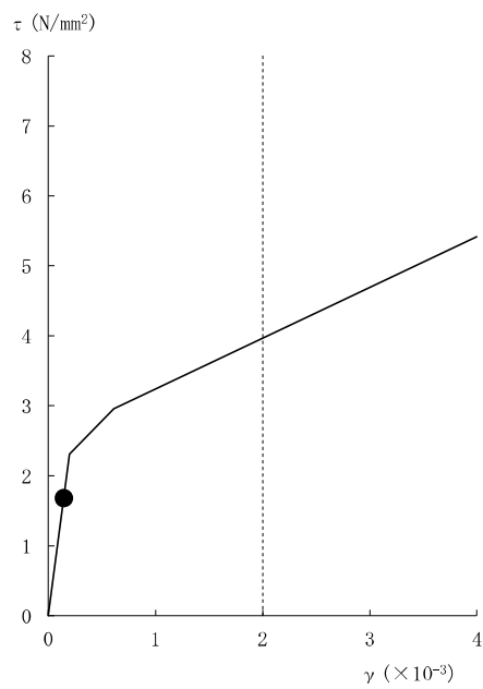
(EW 方向, S s -1, ケース 3, 1F)
