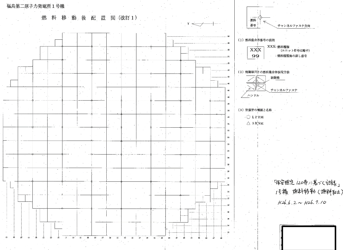
1号炉 燃料集合体炉内装荷配置図
