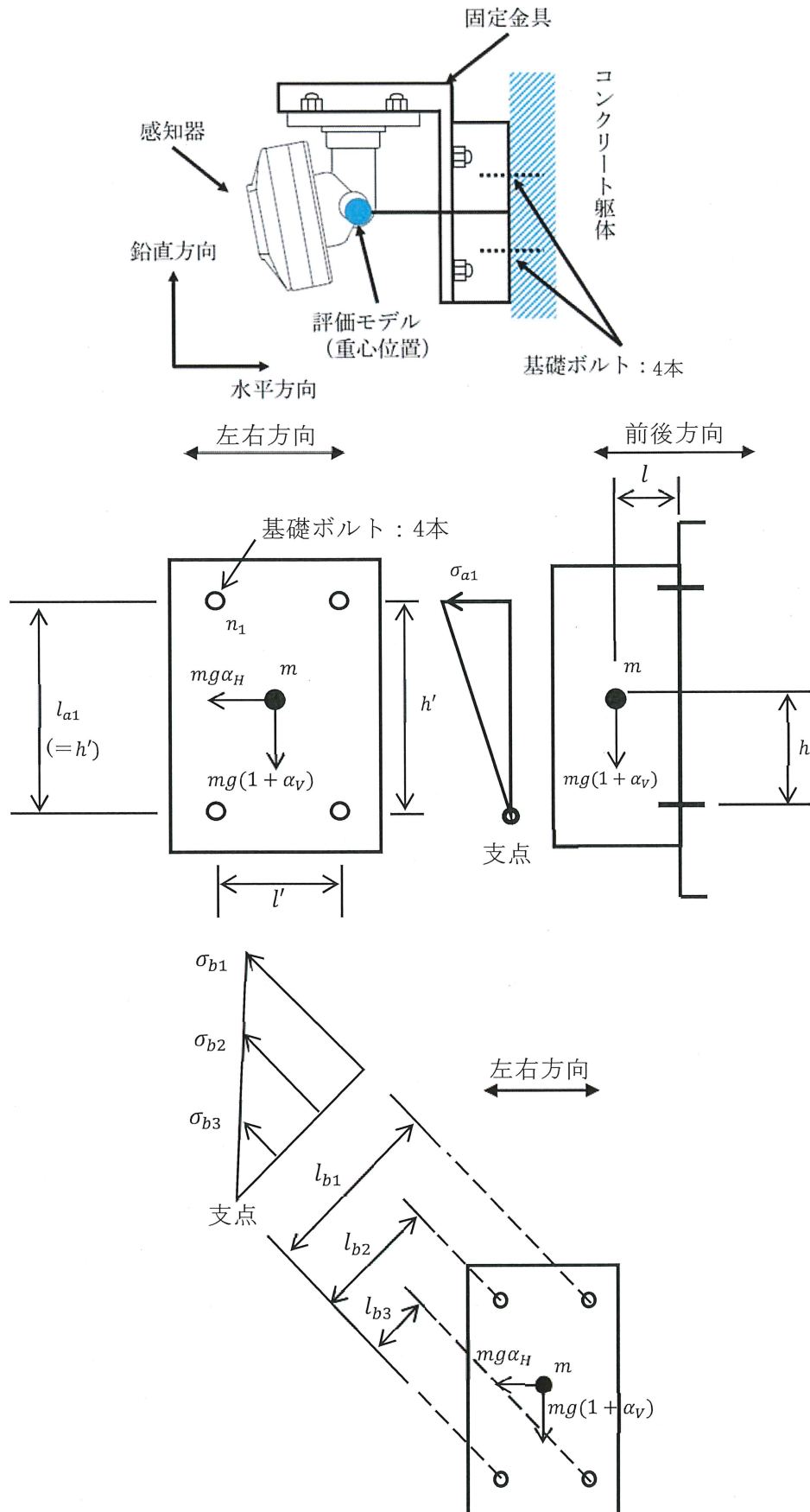
第5-3図 四点固定型（壁掛け型）の応力評価モデル（左右方向）
