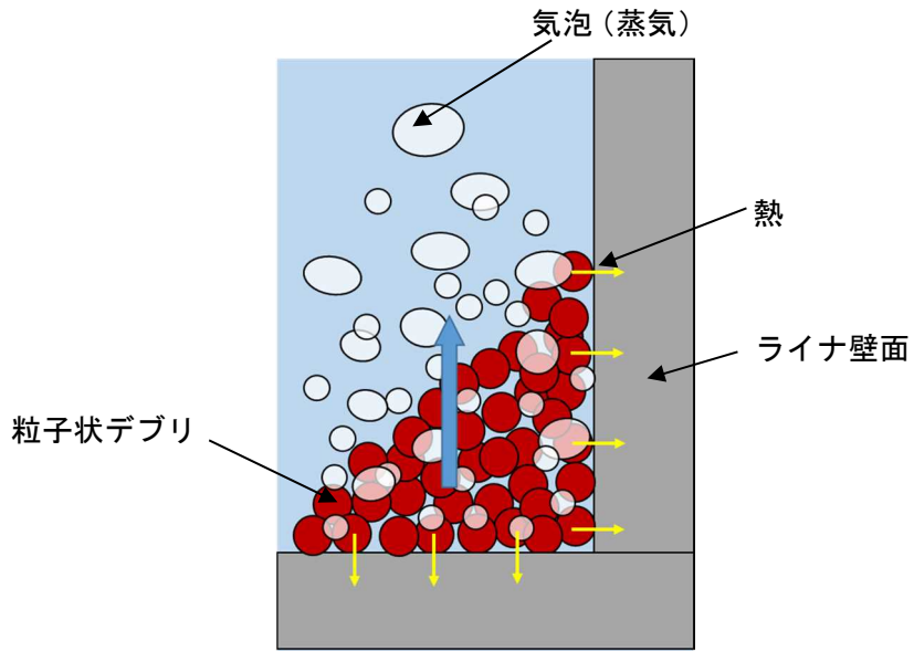
(a) 粒子堆積状デブリのライナ壁面との接触
