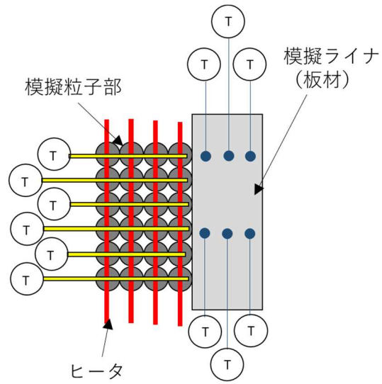
(a) 粒子状デブリの壁面接触実験
