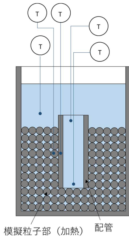
(b) 粒子状デブリの配管接触実験
