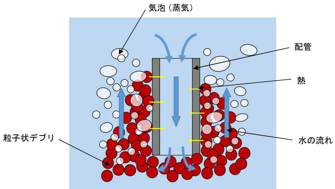
(b) 粒子堆積状デブリの配管との接触
