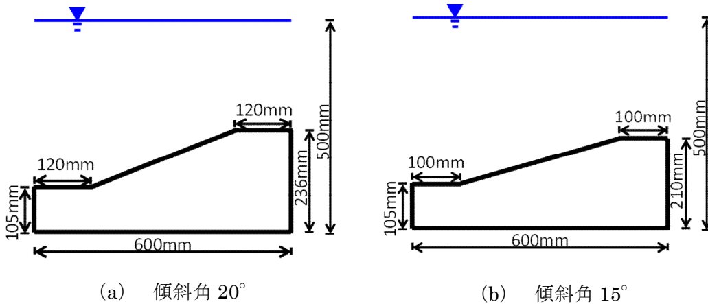
図1 模型地盤の形状 (案)
