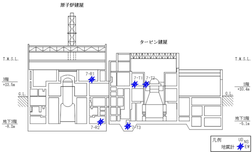
図 3-1 地震計配置図 (7号機)
