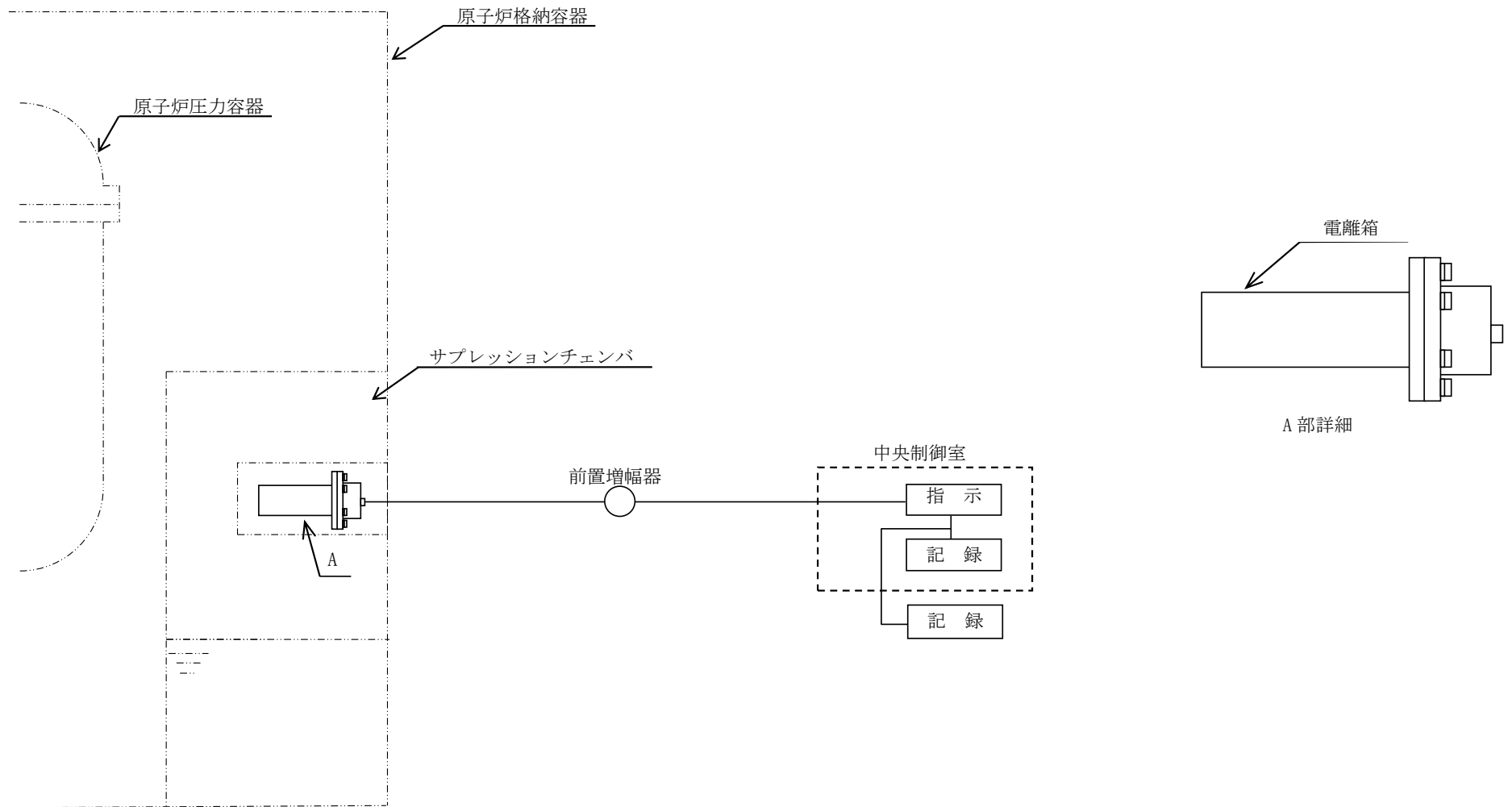
図3-4 検出器の構造図（格納容器内雰囲気放射線モニタ（S/C））
