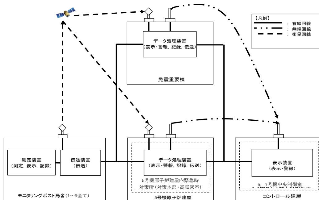
図3-20 固定式周辺モニタリング設備の概略構成図
