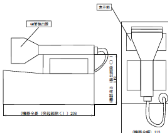
図3-30 検出器の構造図（GM汚染サーベイメータ）
