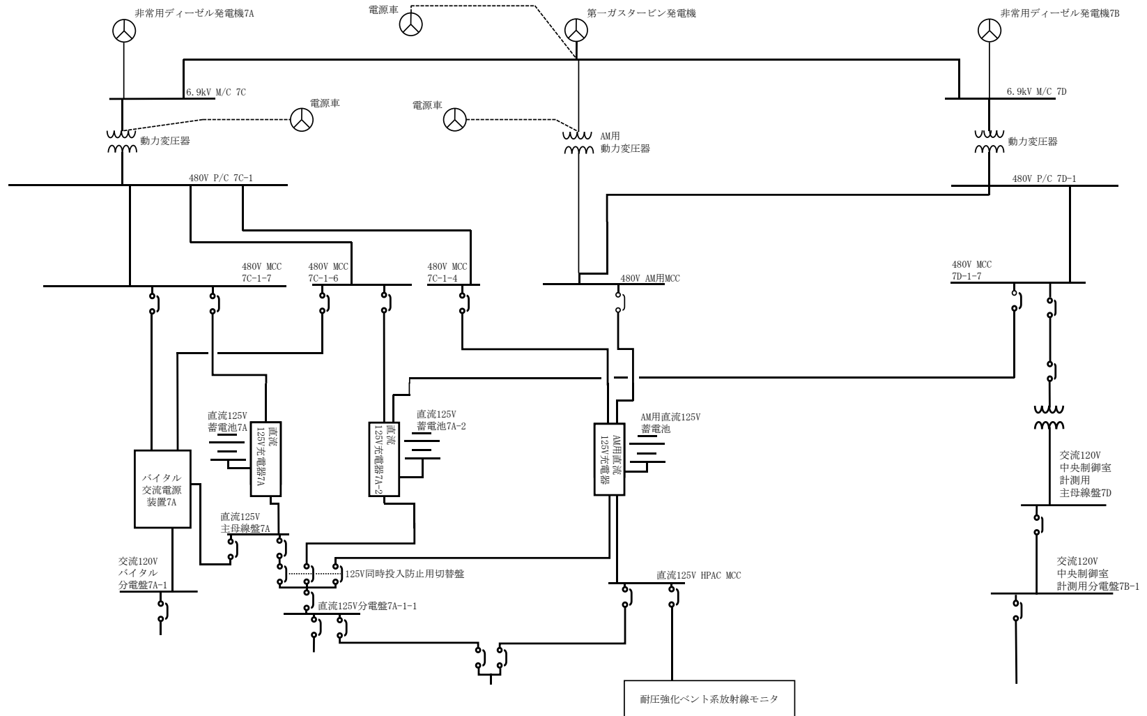
図3-11 耐圧強化ベント系放射線モニタの概略電源系統図（直流電源）
