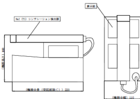
図3-28 検出器の構造図（NaIシンチレーションサーベイメータ）
