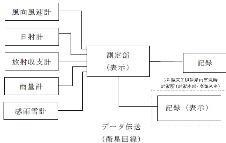
図3-33 可搬型気象観測装置の概略構成図
