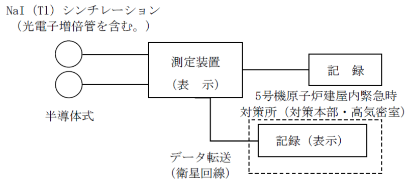
図3-14 5号機原子炉建屋内緊急時対策所（対策本部・高気密室）近傍に設置する可搬型モニタリングポストの概略構成図
