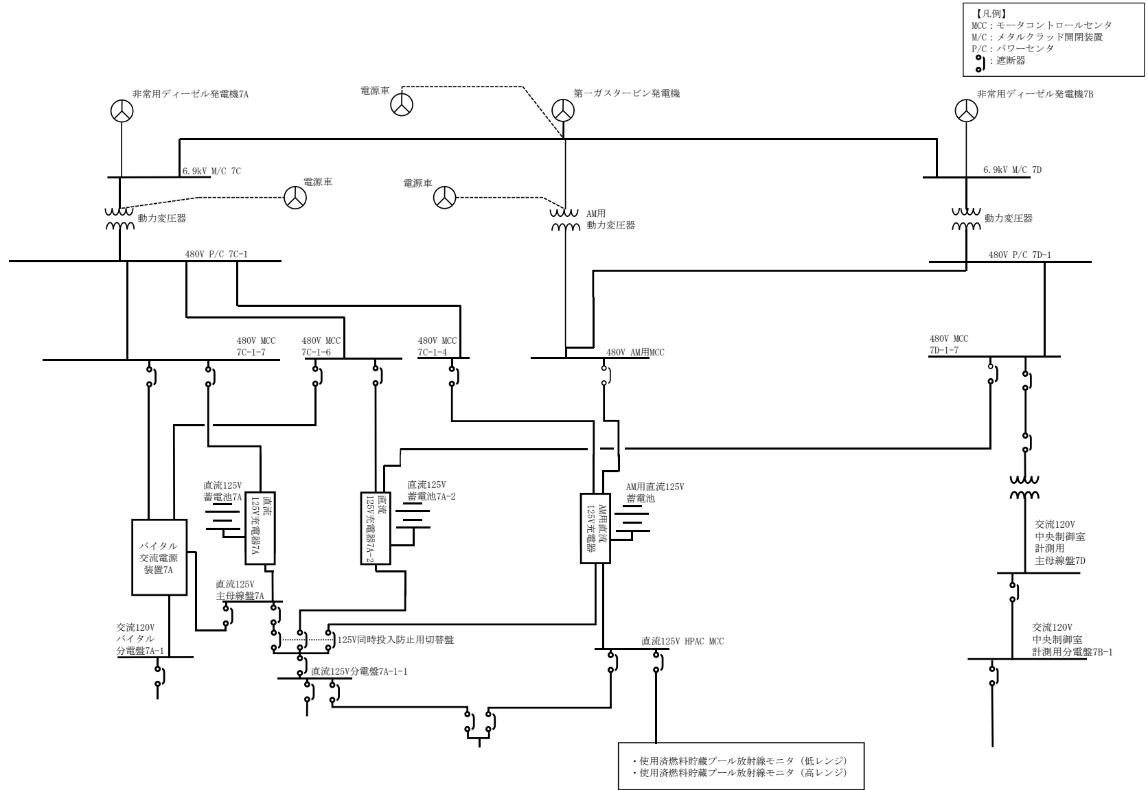
図3-19 使用済燃料貯蔵プール放射線モニタ（低レンジ）（高レンジ）の概略電源系統図（直流電源）
