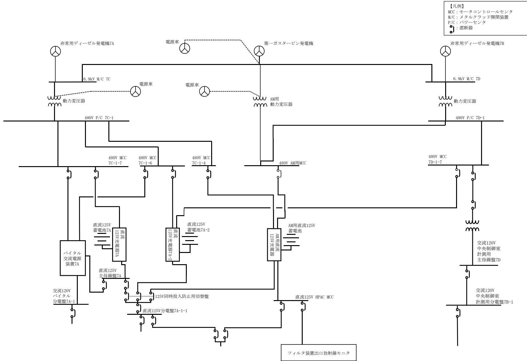
図3-8 フィルタ装置出口放射線モニタの概略電源系統図（直流電源）
