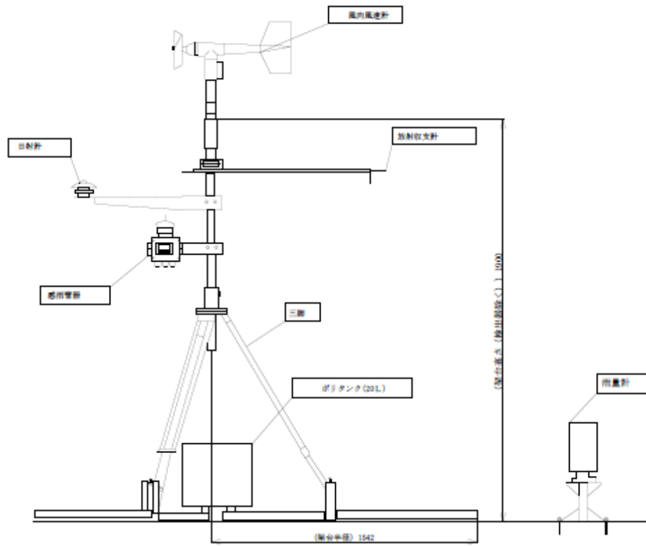
図3-35 「可搬型気象観測装置の構造図」
