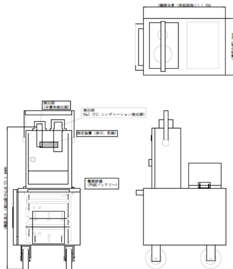
図3-24 検出器の構造図 (可搬型モニタリングポスト)
