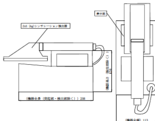
図3-32 検出器の構造図（ZnSシンチレーションサーベイメータ）
