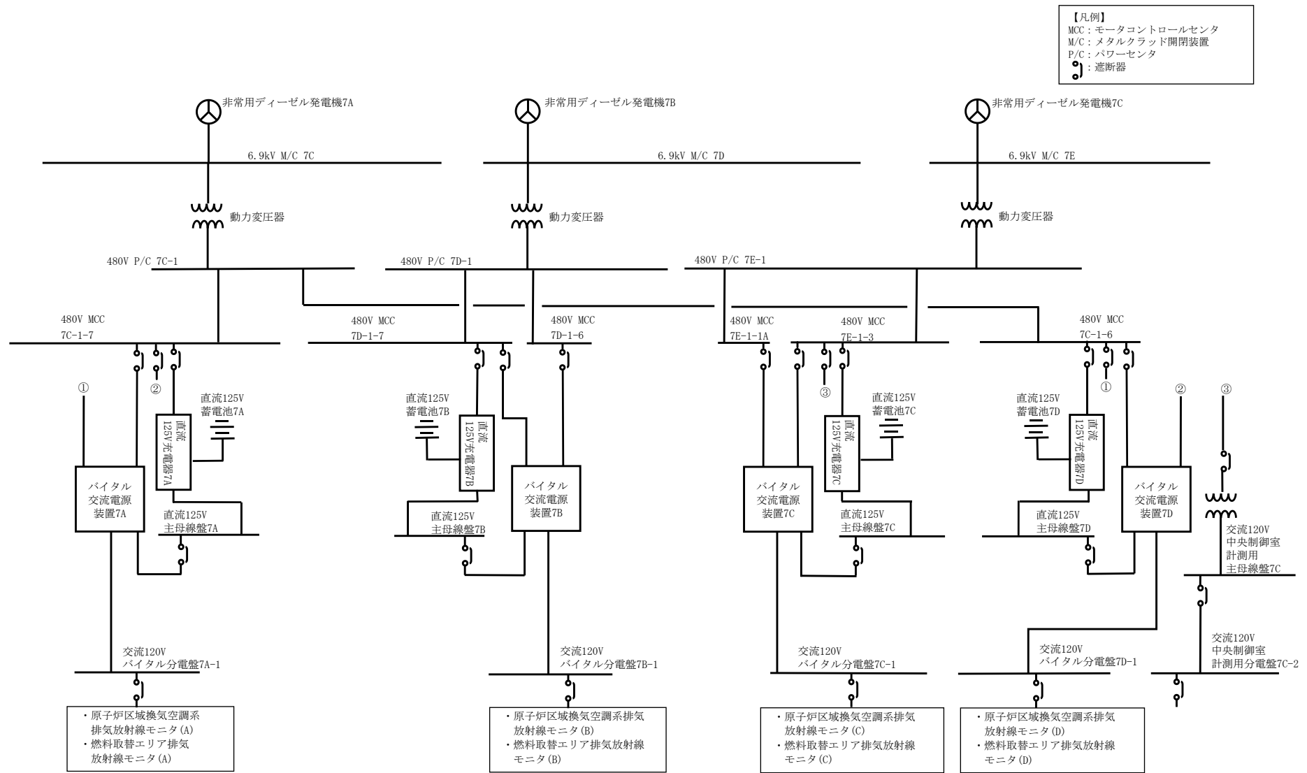
図3-5 燃料取替エリア排気放射線モニタ及び原子炉区域換気空調系排気放射線モニタの概略電源系統図（交流電源）
