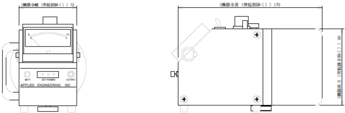
図3-26 検出器の構造図（電離箱サーベイメータ）
