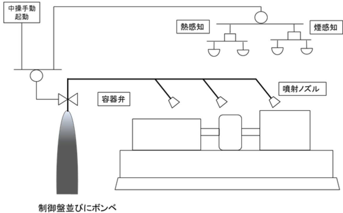
図 5-3 SLC ポンプ・CRD ポンプ局所消火設備 設置概要図
