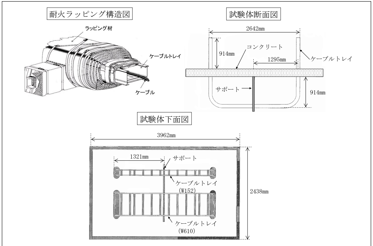
図 6-7 耐火ラッピングの耐火試験体
