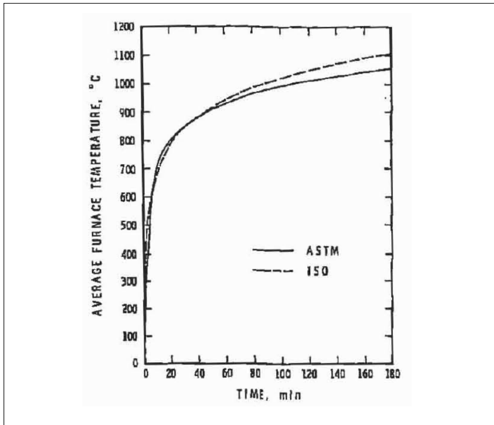
圖 6-6 A S T M E 1 1 9 加熱曲線
