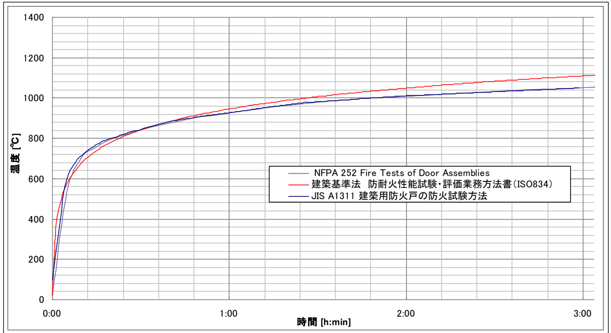
図 6-1 建築基準法 (ISO 834) 加熱曲線
