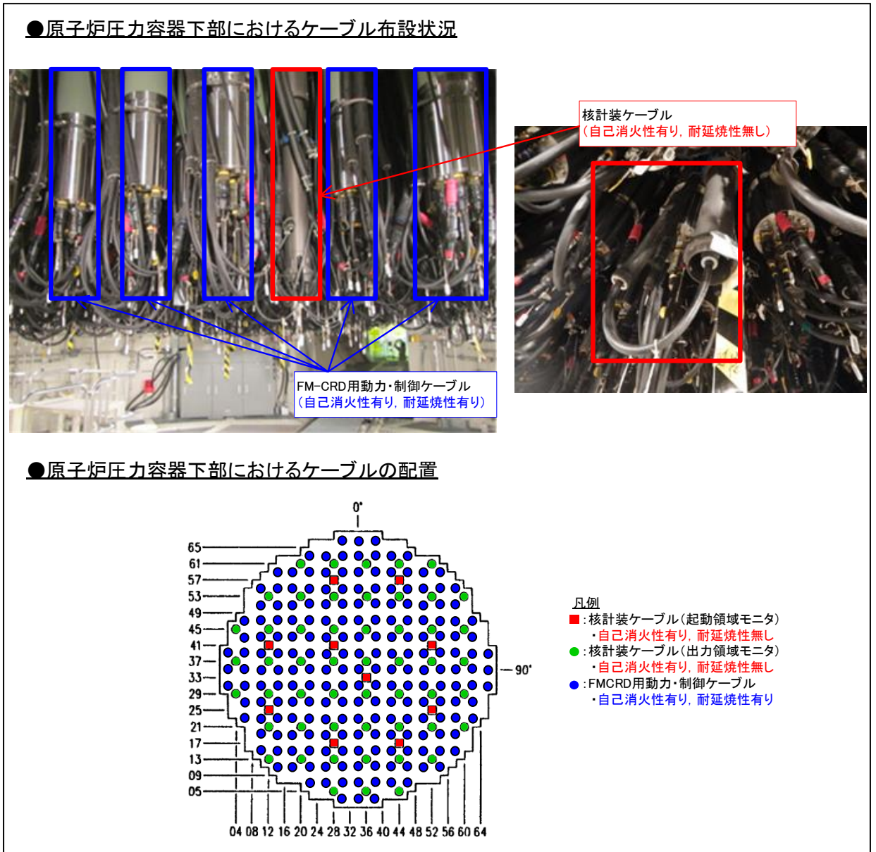
図 6-8 ケーブル敷設状況及び起動領域モニタの位置的分散
