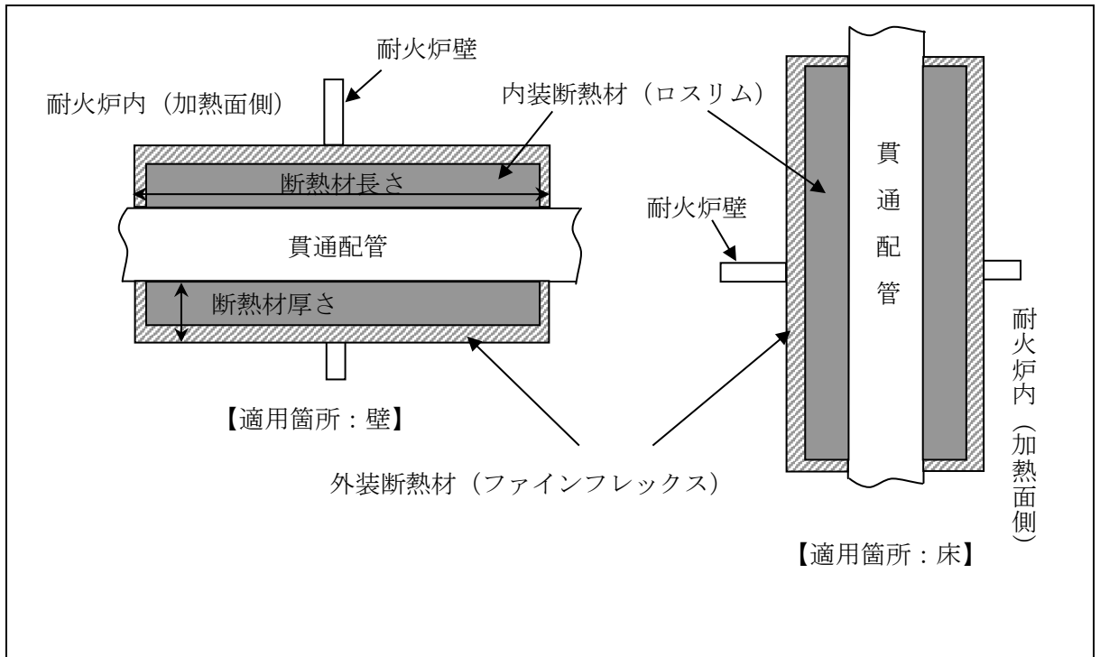
図 6-2 貫通部シール (配管貫通部) の耐火試験体
