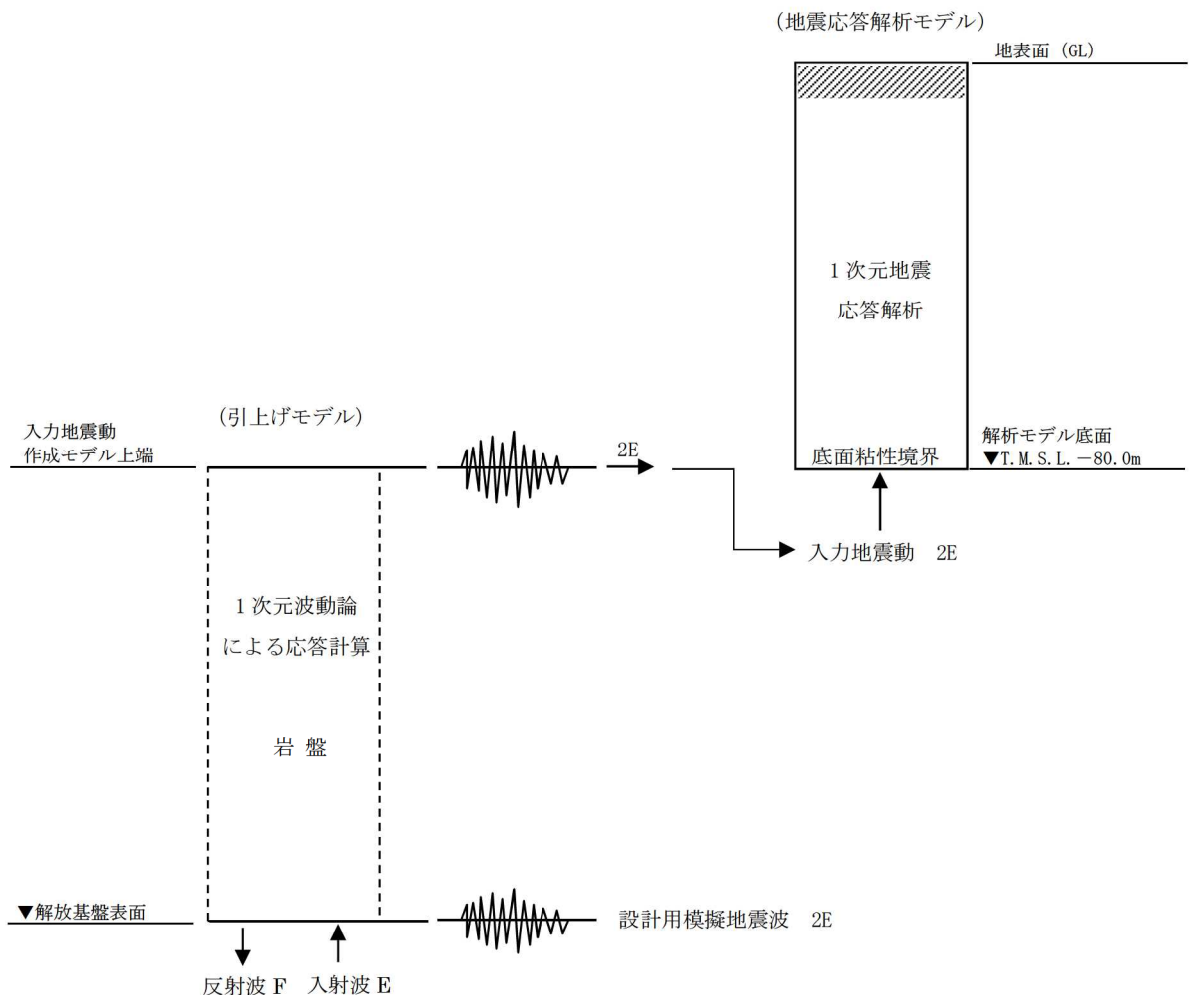
図2-15 モデル下端の入力地震動算定の考え方
