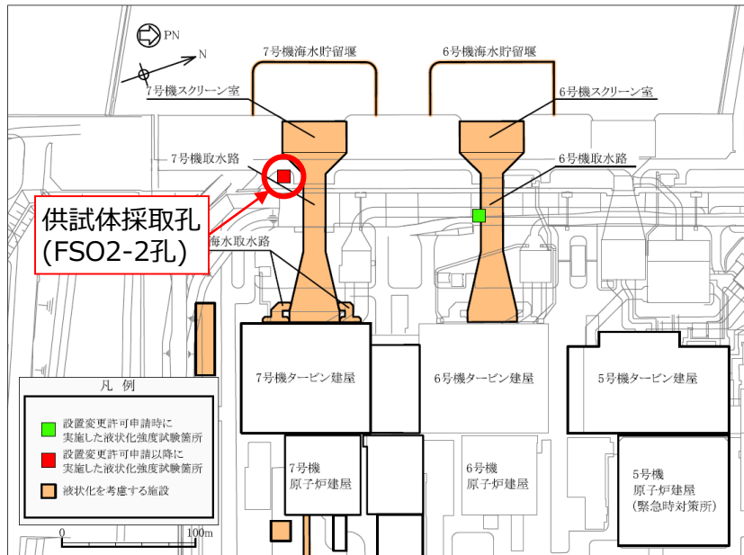
A2s層の液状化強度試験供試体の採取位置
