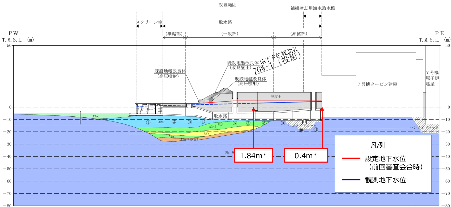
施設の設置区間の地下水位設定と観測地下水水位との関係（前回審査会合時）
