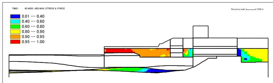
過剰間隙水圧比の分布（北断面）
