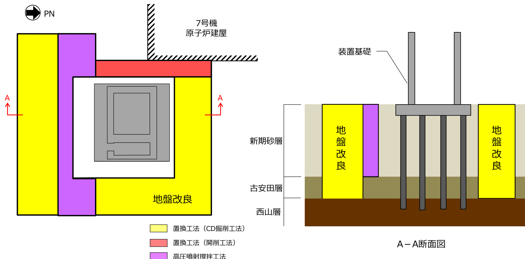
地盤改良範囲図
