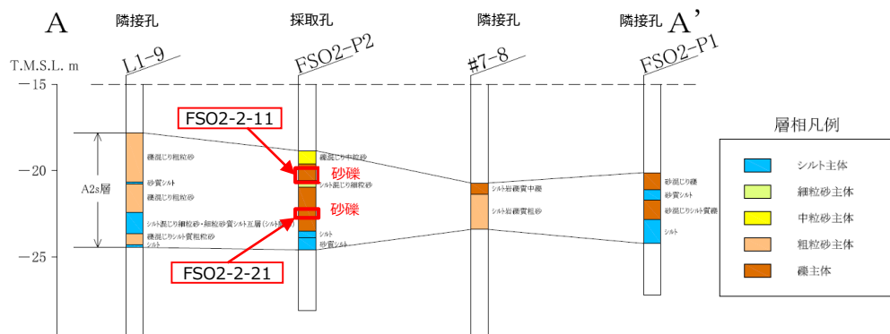
ボーリング柱状図
