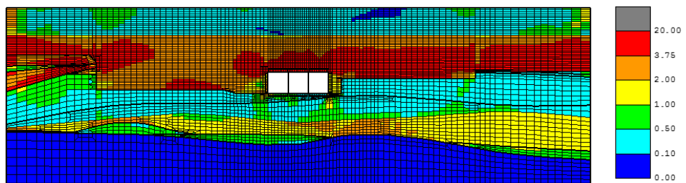
最大せん断ひずみ分布図 (下限値ケース)
