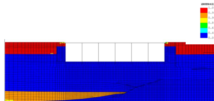
地震終了時の過剰間隙水圧比分布 (曲げ軸力照査値最大となる解析ケース①・地震動 S_s -3---)
