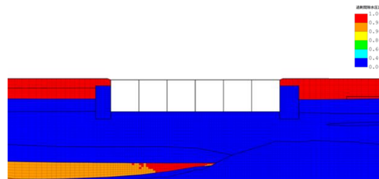
最大過剰間隙水圧比分布 (曲げ軸力照査値最大となる解析ケース①・地震動 S_s -3---)
