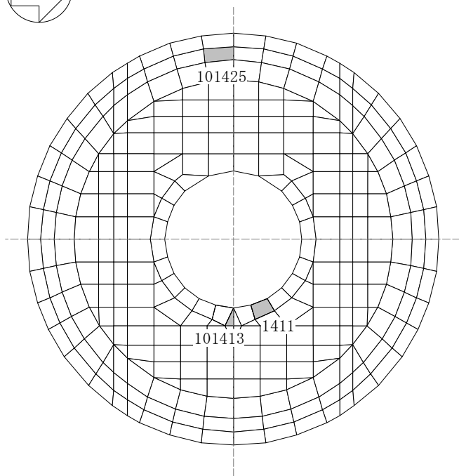
(b) トップスラブ部
