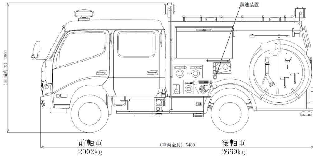
図 2-14 可搬型代替注水ポンプ（A-2 級）の仕様
