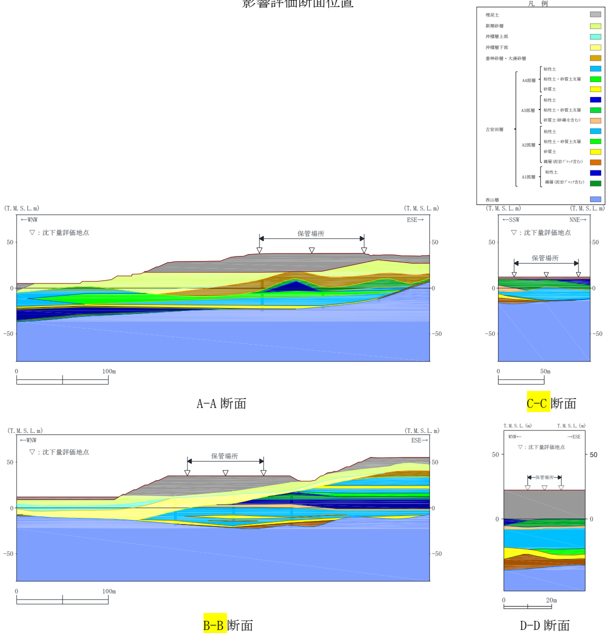
図 2-9 液状化及び揺すり込みによる不等沈下に対する影響評価断面位置図及び断面図
