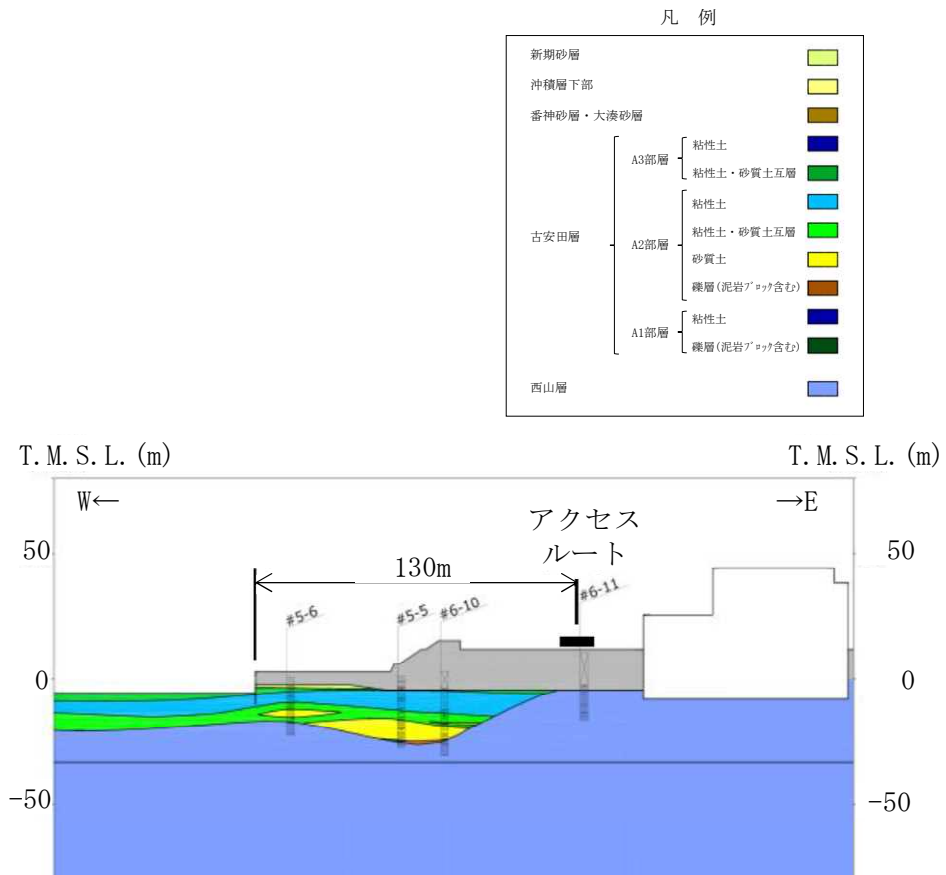
地質断面図
