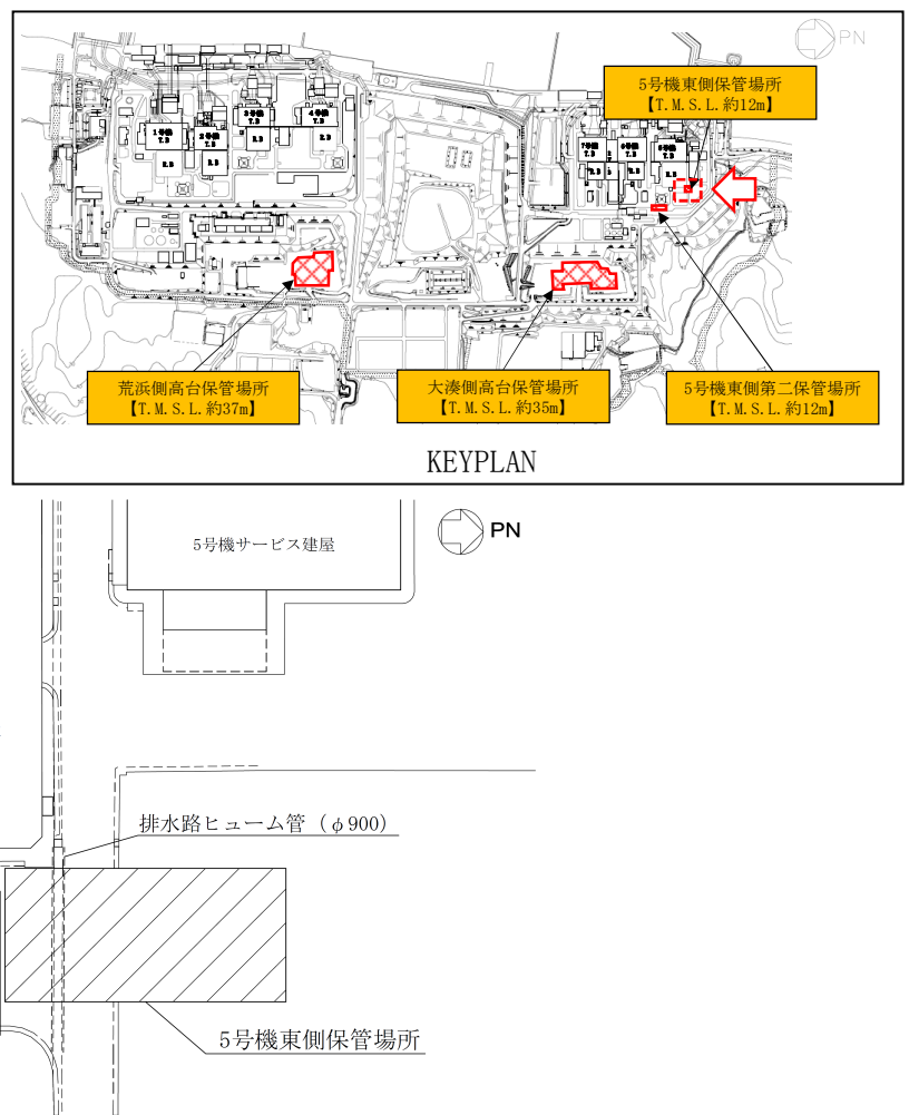
図2-10 保管場所を横断する地中埋設構造物位置図（5号機東側保管場所）
