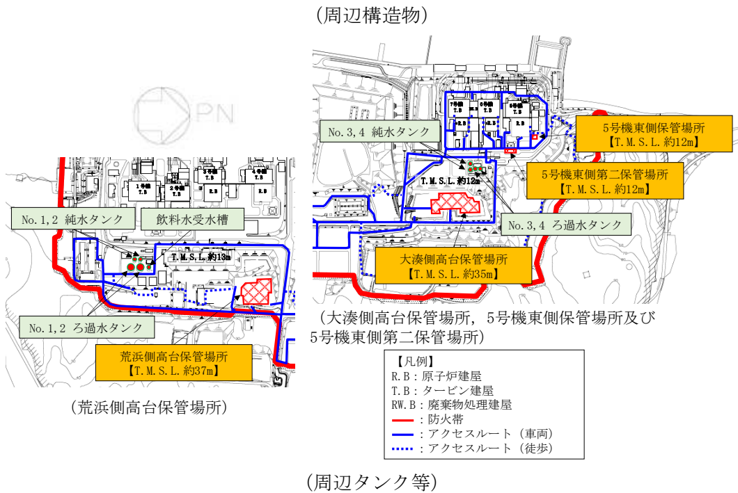
図 2-3 周辺構造物及び周辺タンク等の配置図
