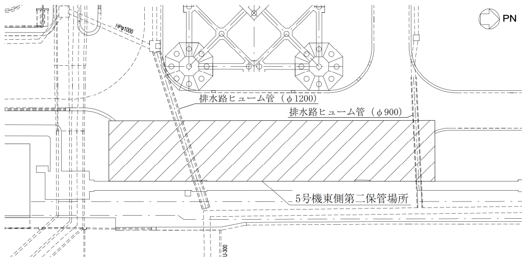
図 2-11 保管場所を横断する地中埋設構造物位置図 (5号機東側第二保管場所)
