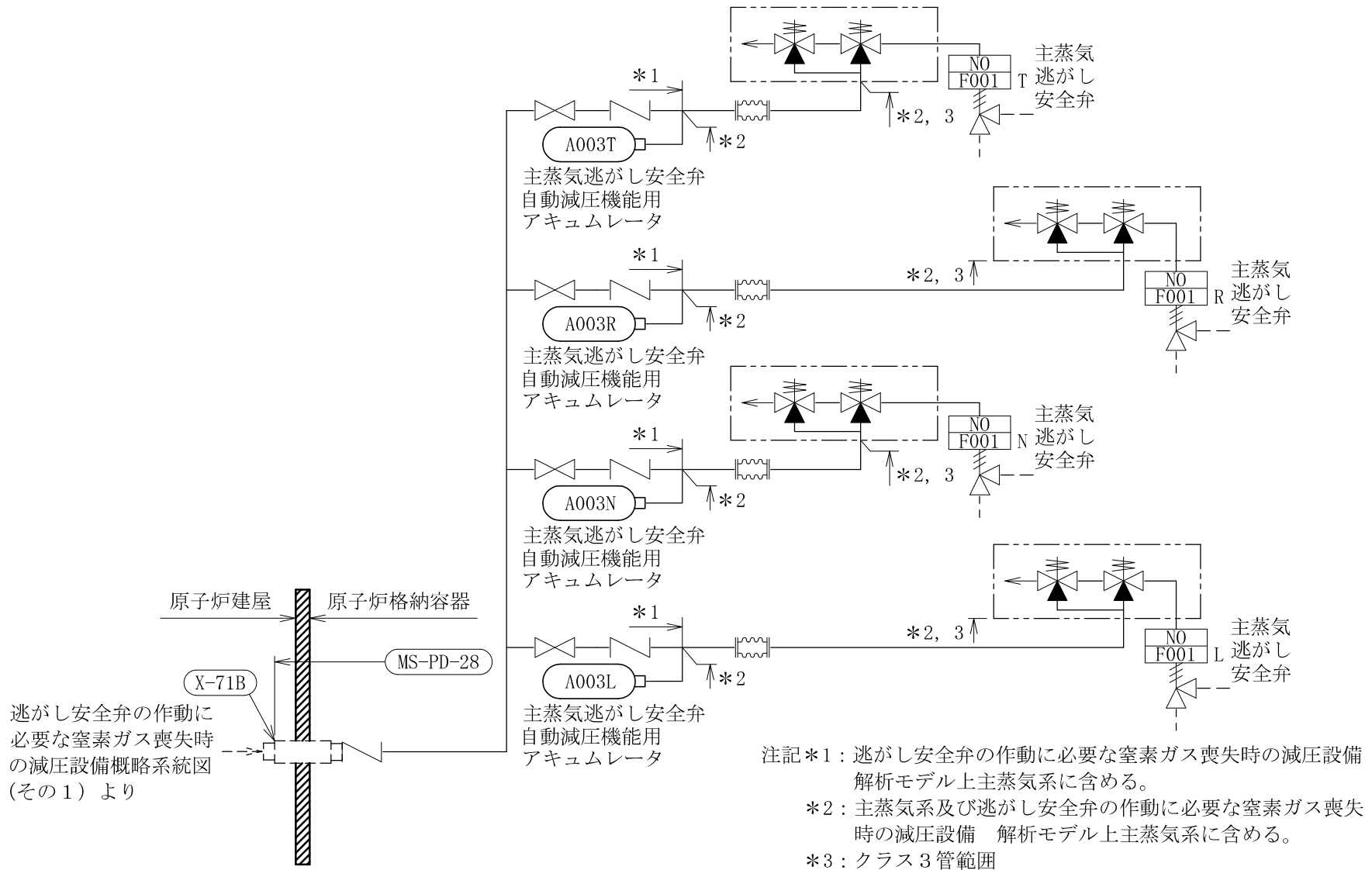
逃がし安全弁の作動に必要な窒素ガス喪失時の減圧設備概略系統図 (その5)
