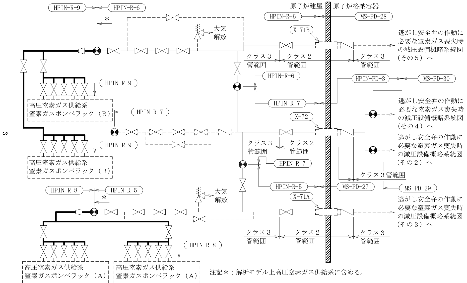
逃がし安全弁の作動に必要な窒素ガス喪失時の減圧設備概略系統図 (その 1)
