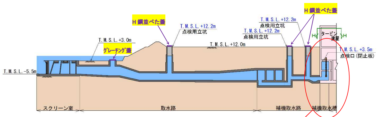
図 3.2-参 1-1 7号機取水路 (断面)
