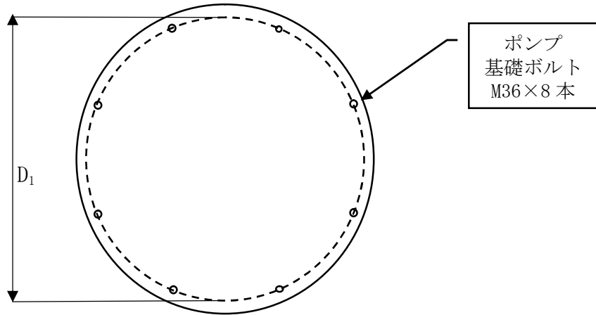
図 3.2-2 原子炉補機冷却海水ポンプ、ポンプ基礎ボルト配置
