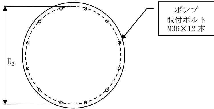
図 3.2-3 原子炉補機冷却海水ポンプ，ポンプ取付ボルト配置
