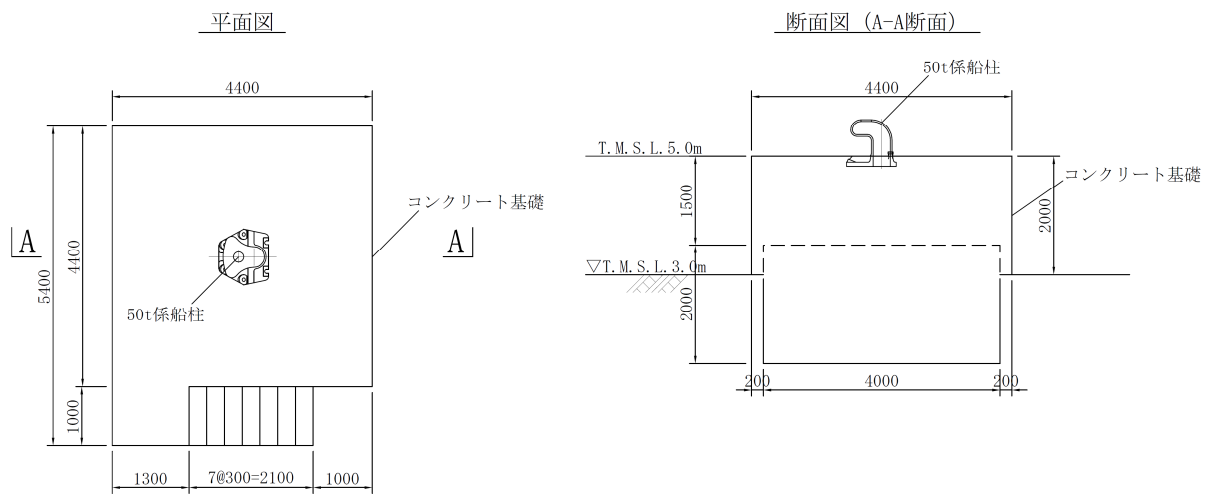
(4) 50t 係船柱コンクリート基礎図
