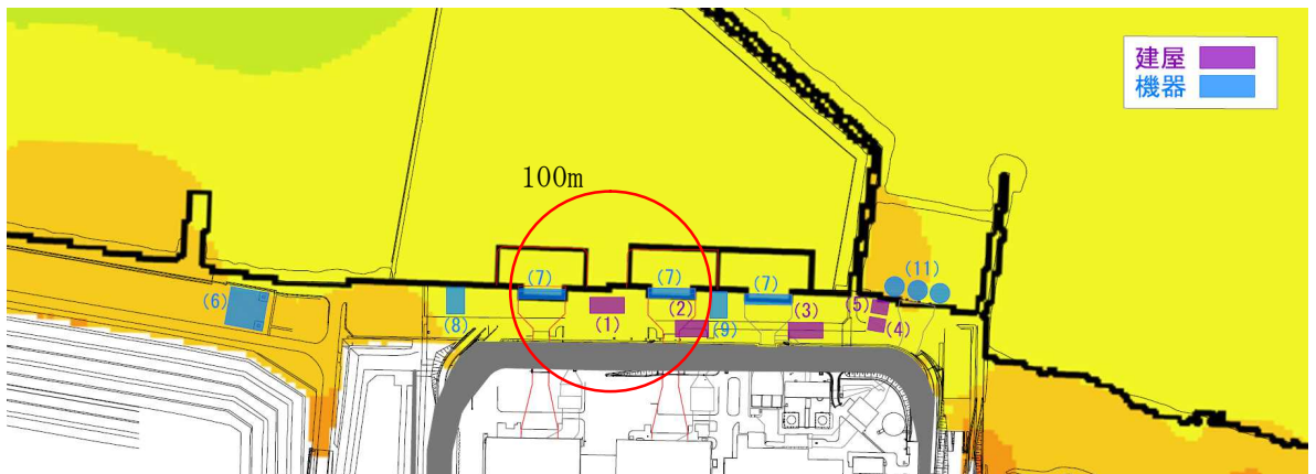
図4.2-24-2 検討対象とする鉄筋コンクリート建屋の抽出範囲
