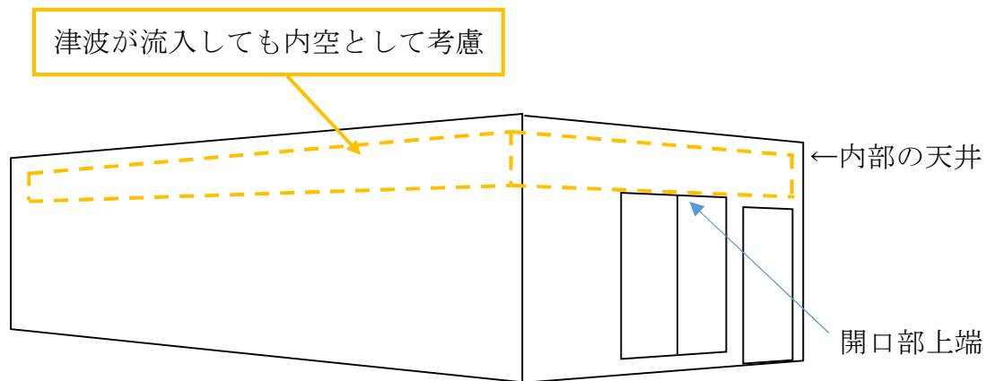
図 4.2-24-3 開口部から鉄筋コンクリート建屋内部に津波が流入しても 内空として考慮する空間のイメージ図
