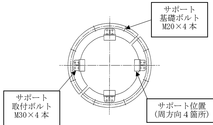
図 3.2-5 コラムパイプサポート部平面図
