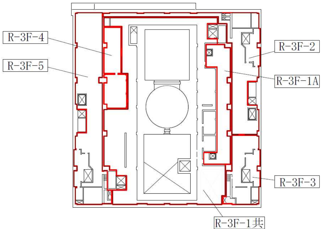
原子炉建屋 T. M. S. L. +23500
