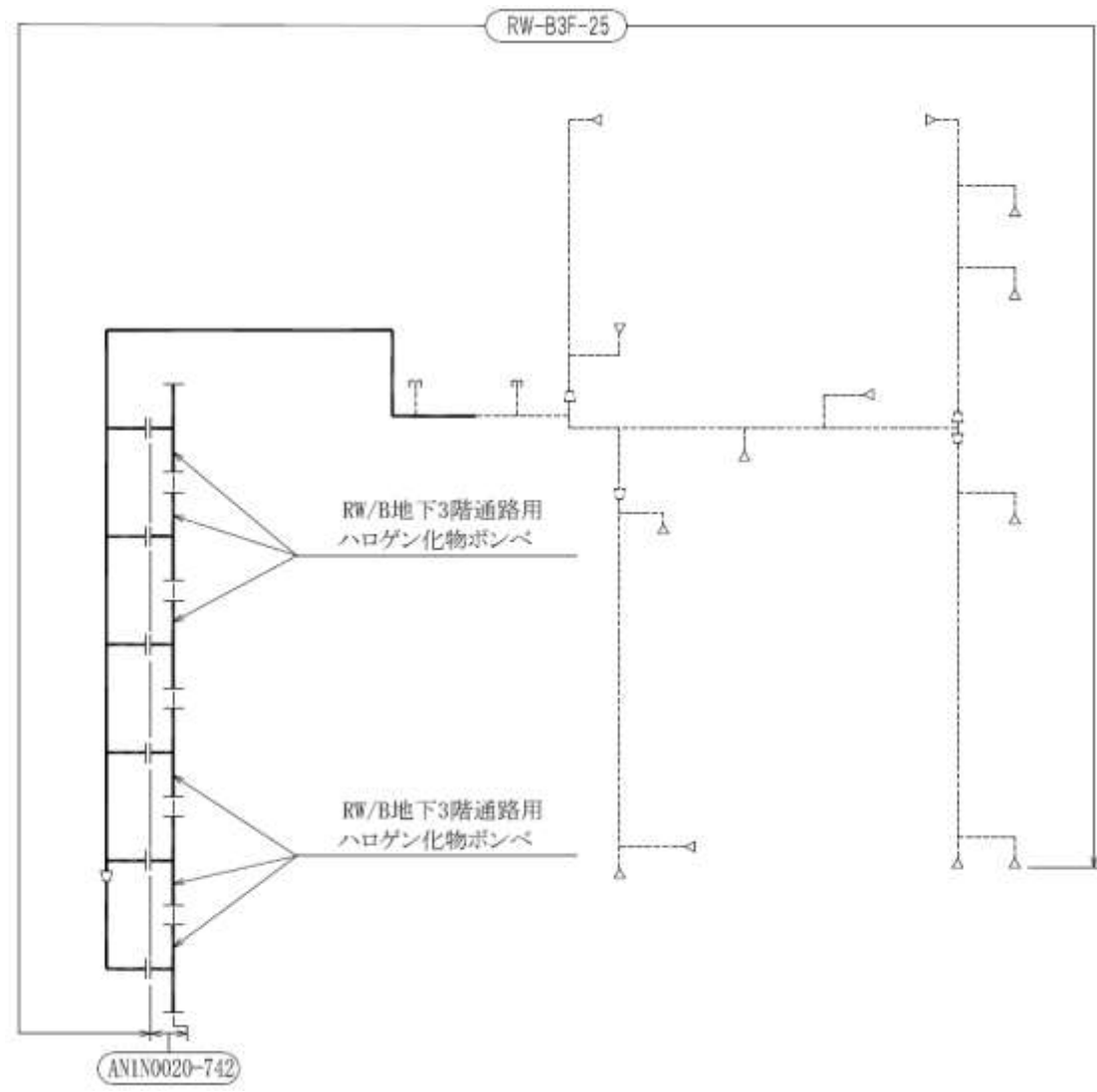
小空間固定式消火設備概略系統図 (その 80)
