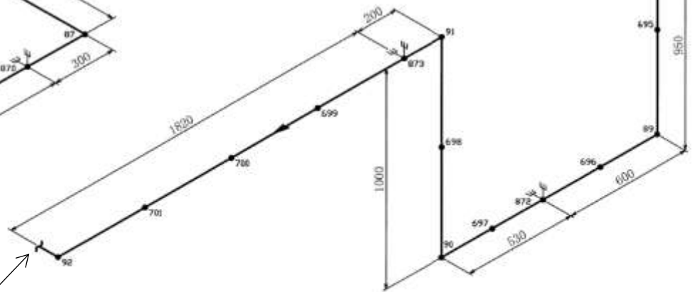
鳥瞰図 中央制御室床下フリーアクセスフロア(10/13)に接続
