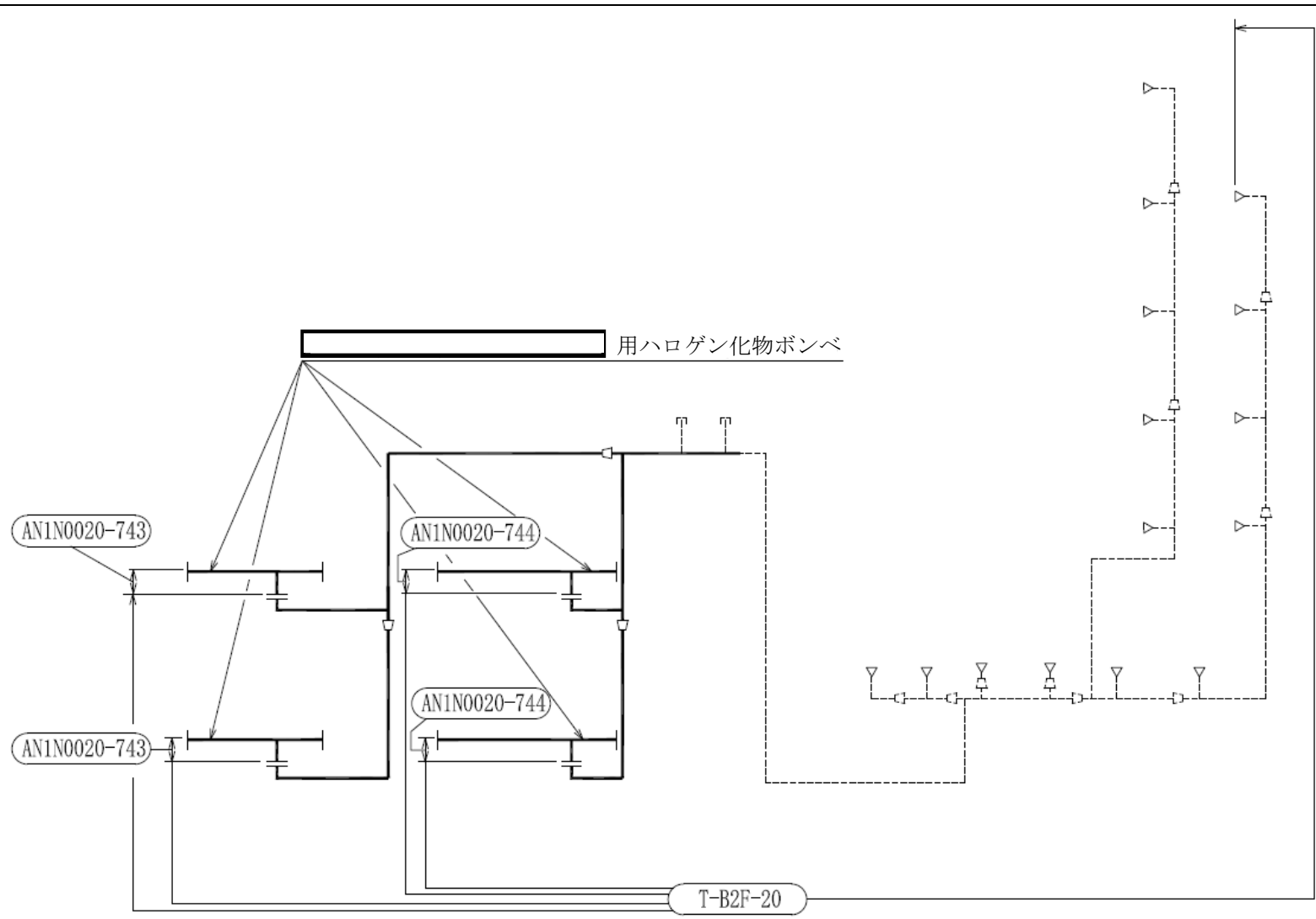
小空間固定式消火設備概略系統図 (その 54)
