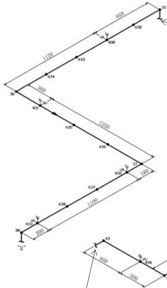
鳥瞰図 中央制御室床下フリーアクセスフロア (7/13)に接続
