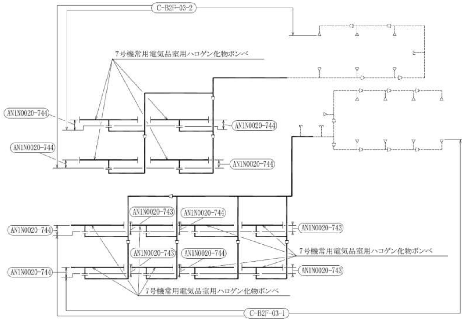
小空間固定式消火設備概略系統図 (その 67)
