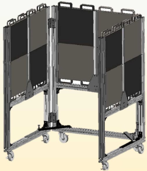
可搬式の遮蔽体を製作。遮蔽プレートをフレームに必要な数セット(最大24枚)することで、周辺BGの影響を低減できる。
