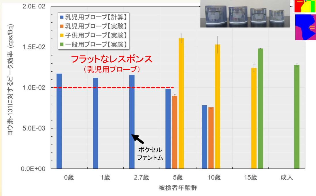
年齢別ファントムに対する 131 Iのピーク効率
