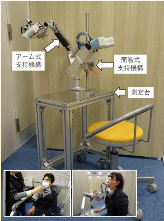
研修会受講生及び研究評価委員のコメントを踏まえ、測定者の負担を軽減するためのモニタ支持機構を製作。
