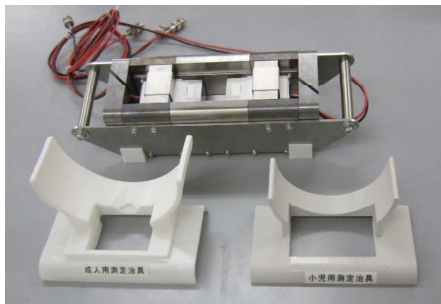
成人用 測定治具
