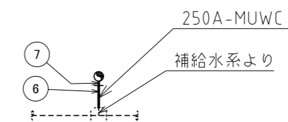
A~A矢視図
