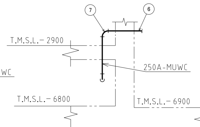
E~E矢視図
