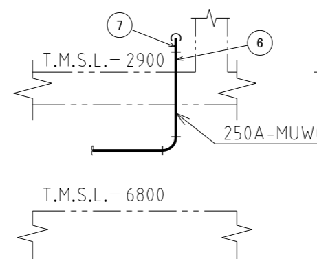
D~D矢視図
