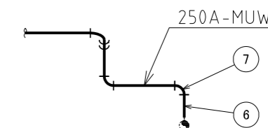
C~C矢視図
