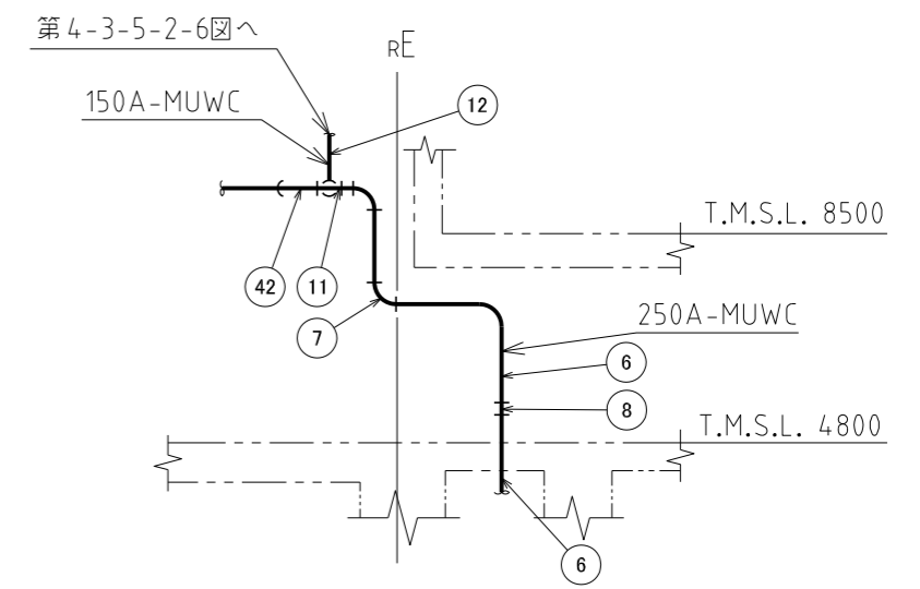
A~A矢視図
