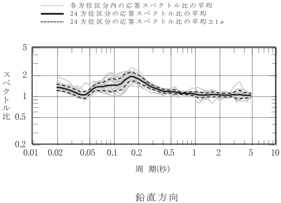
図 5-6(1) 鉛直アレイ観測記録の応答スペクトル比
