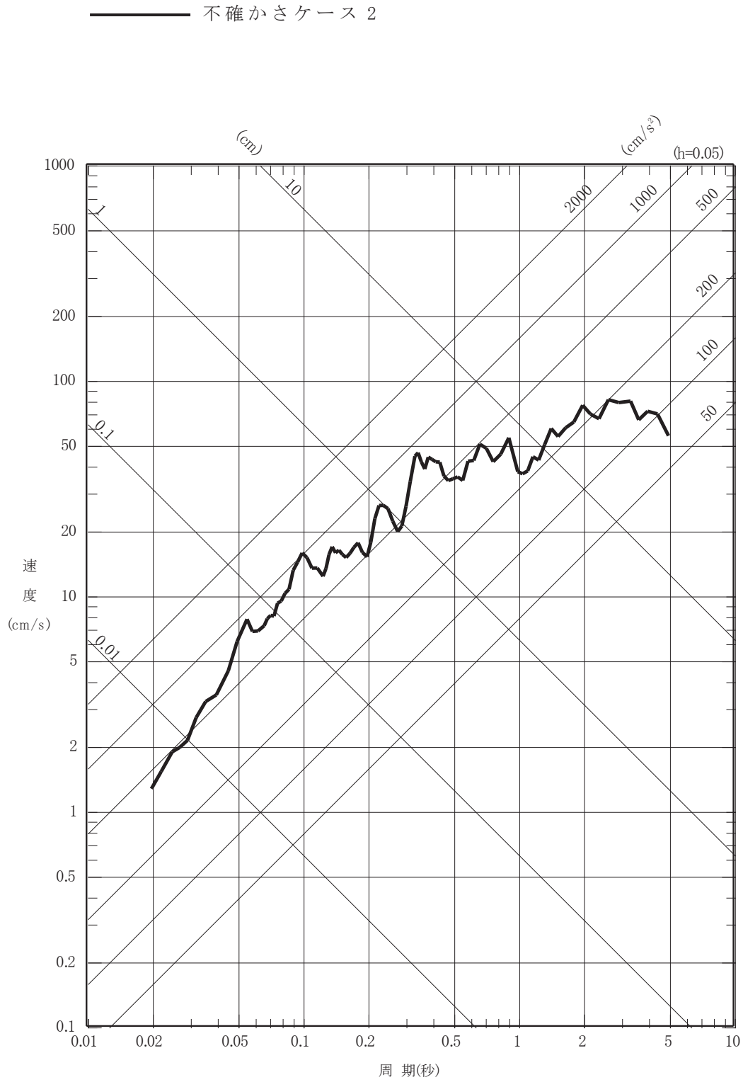
図 6-10(2) 2011 年東北地方太平洋沖型地震の断層モデルを用いた手法による地震動評価 不確かさケース 2 (鉛直方向)
