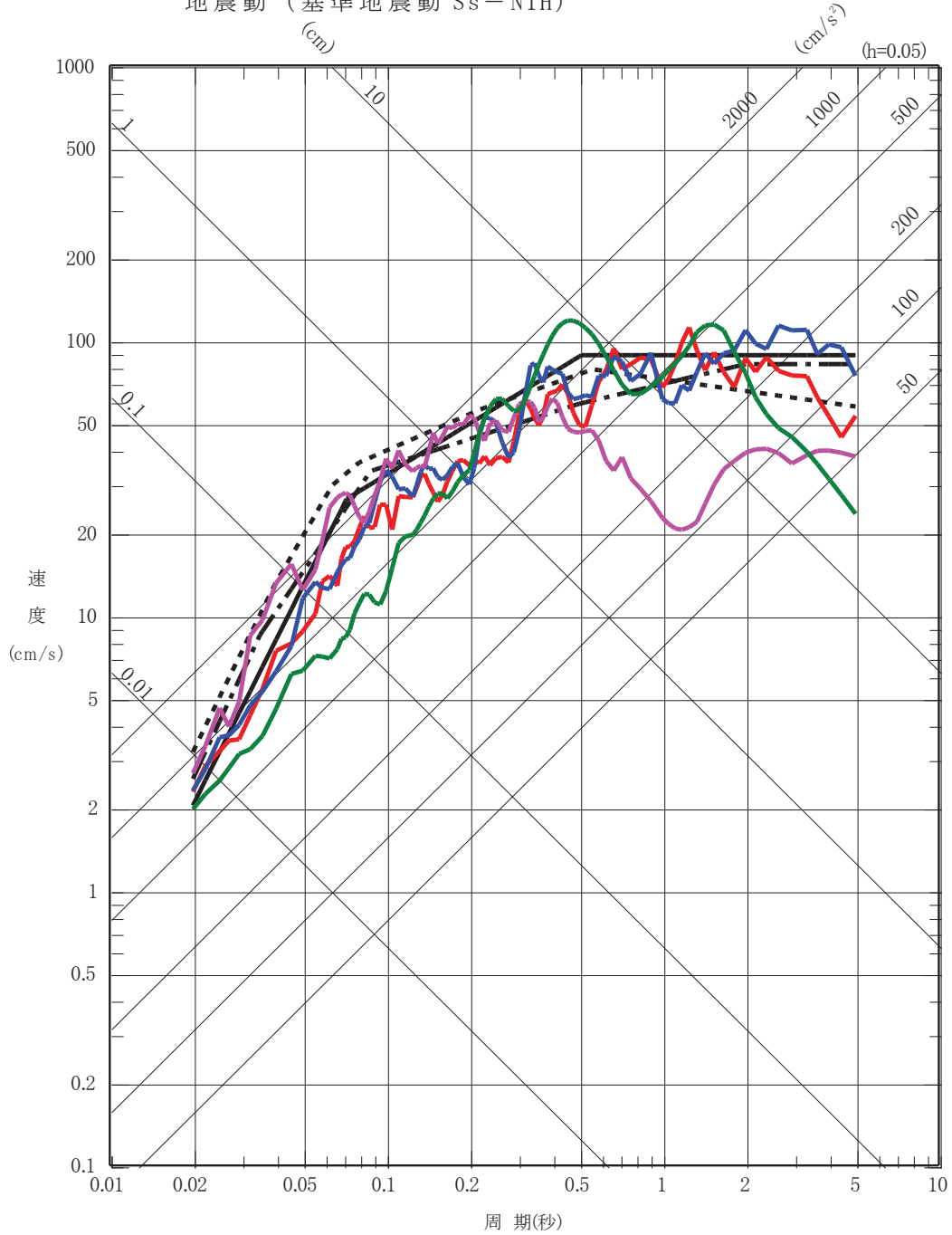
図 6-45(1) 「震源を特定せず策定する地震動」に基づく 基準地震動 S s (水平方向)
