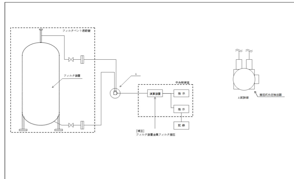
図 3-67 検出器の構造図 (フィルタ装置水位)
