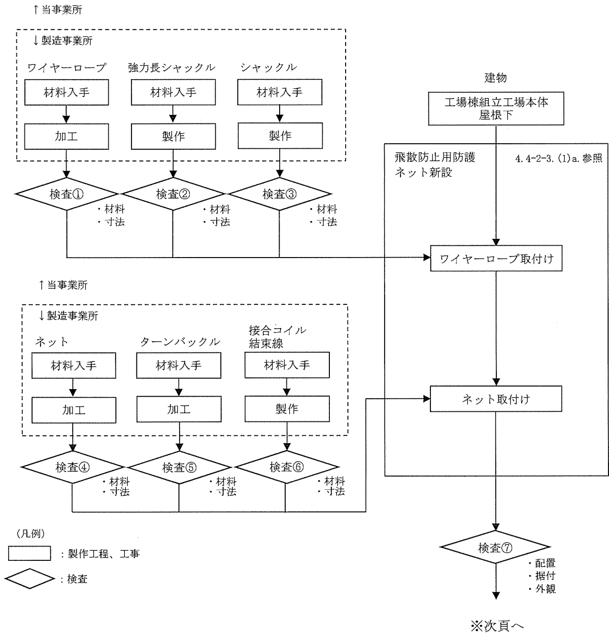
図リ 4-2-3 工場棟組立工場 緊急対策設備(2)飛散防止用防護ネット新設 の手順フロー図 (1/2)
