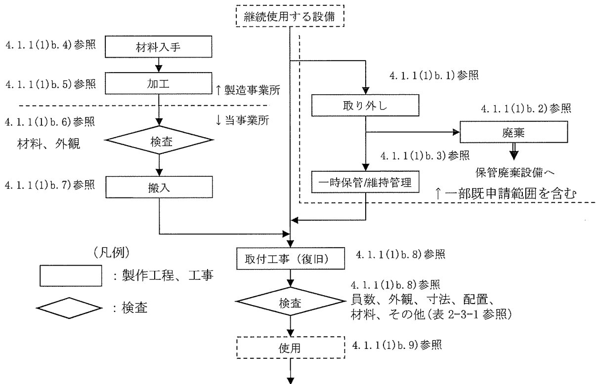
工場棟転換工場 (図イ 2-1)
