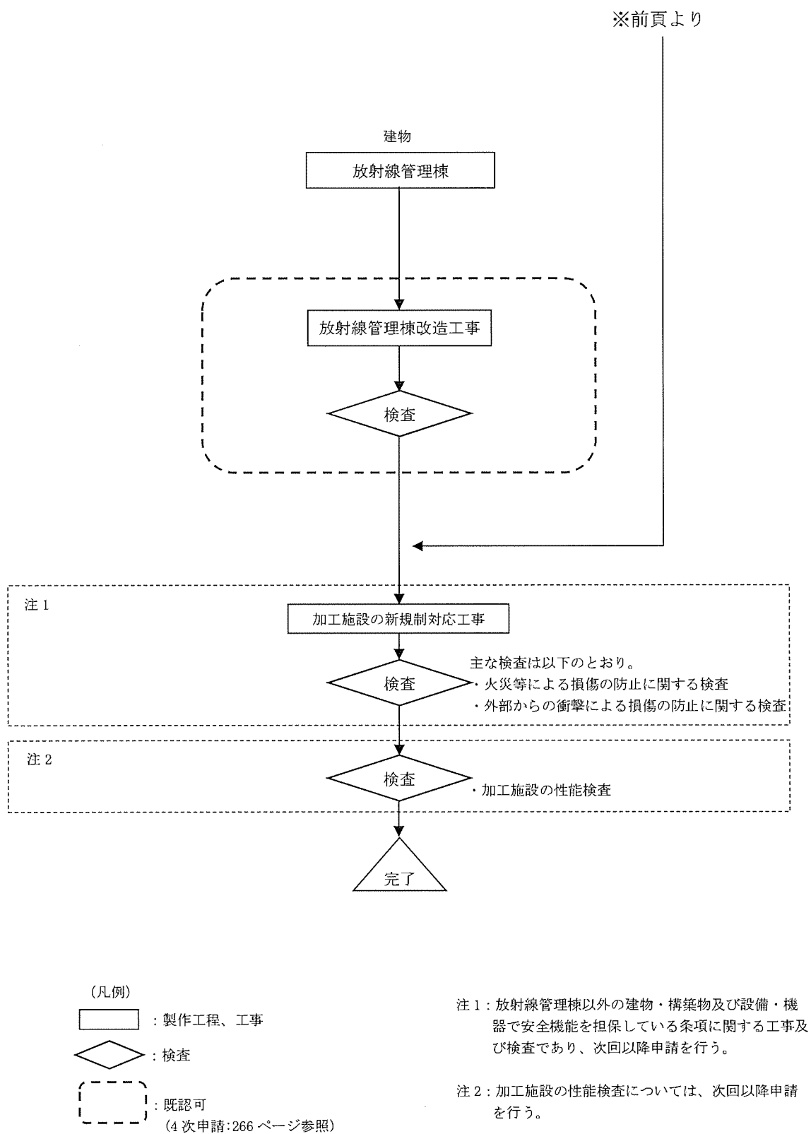
図リ 4-2-5 放射線管理棟 緊急対策設備(2)飛散防止用防護ネット新設の手順フロー図 (2/2)
