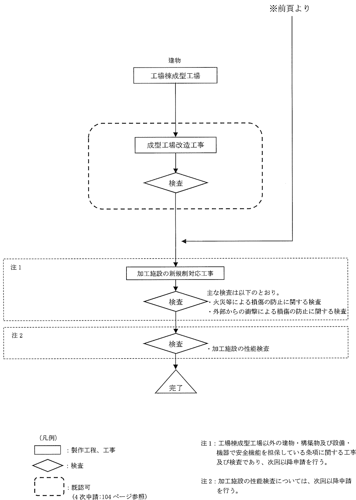
図リ 4-2-2 工場棟成型工場 緊急対策設備(2)飛散防止用防護ネット新設の手順フロー図 (2/2)
