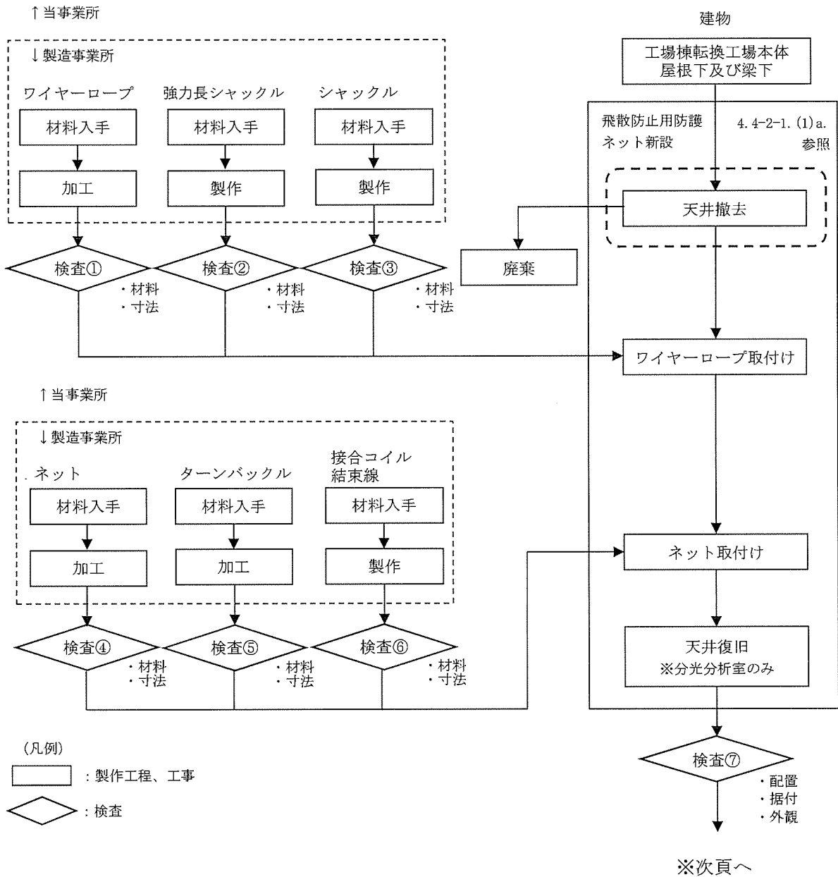
図リ 4-2-1 工場棟転換工場 緊急対策設備(2)飛散防止用防護ネット新設 の手順フロー図 (1/2)
