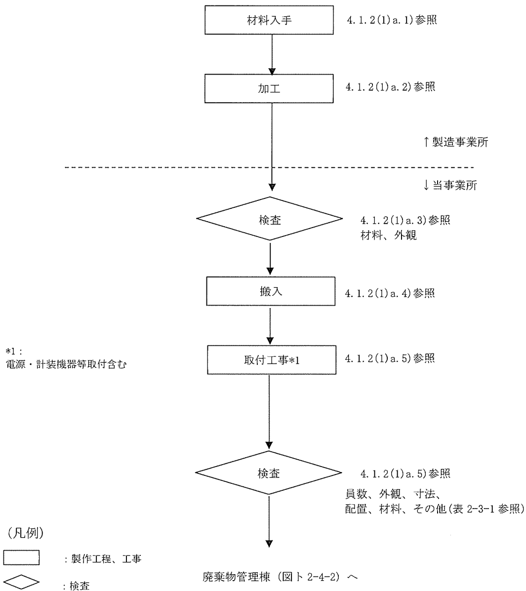
図ト 2-4-3 工事の手順フロー図
