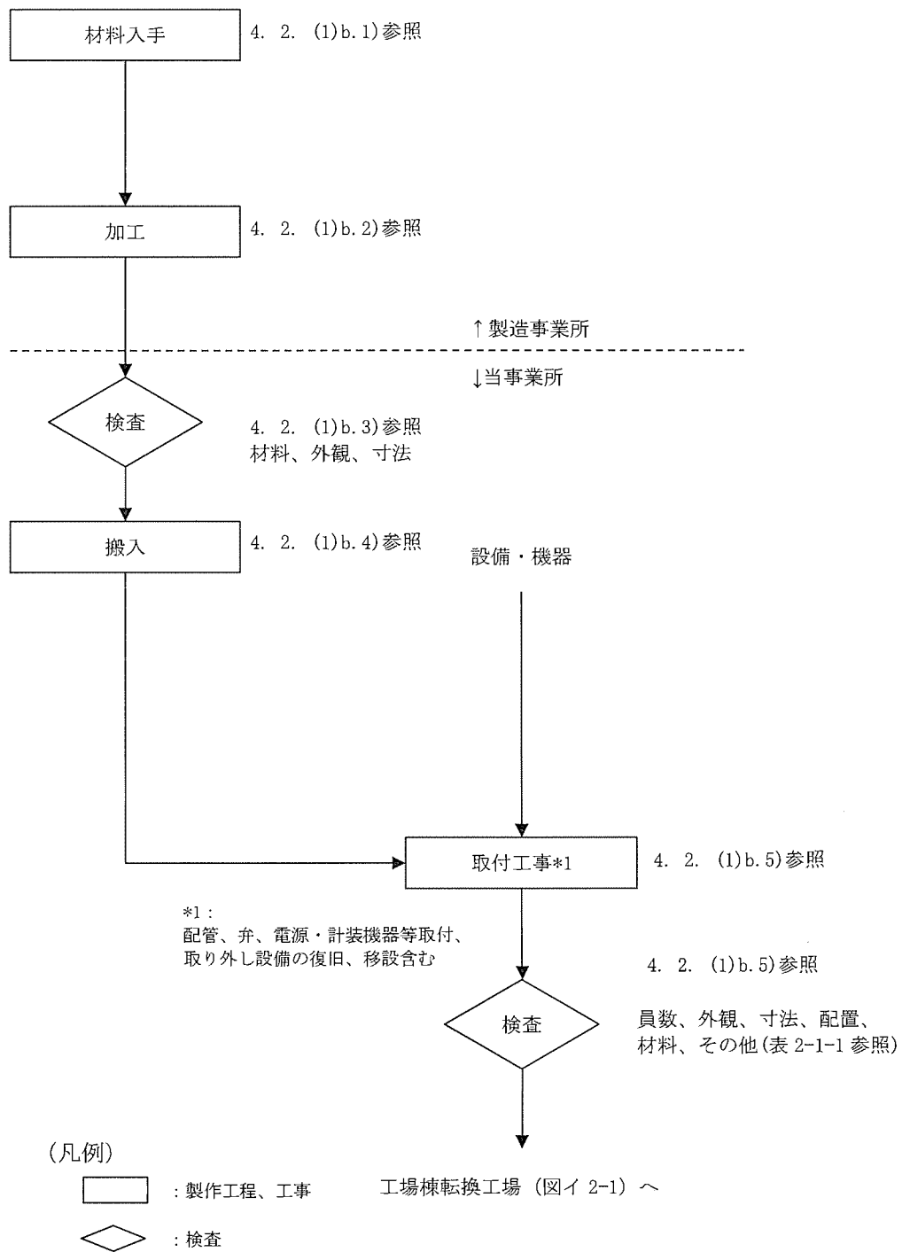
図イ 2-2-2 工事の手順フロー図 (改造する場合)
