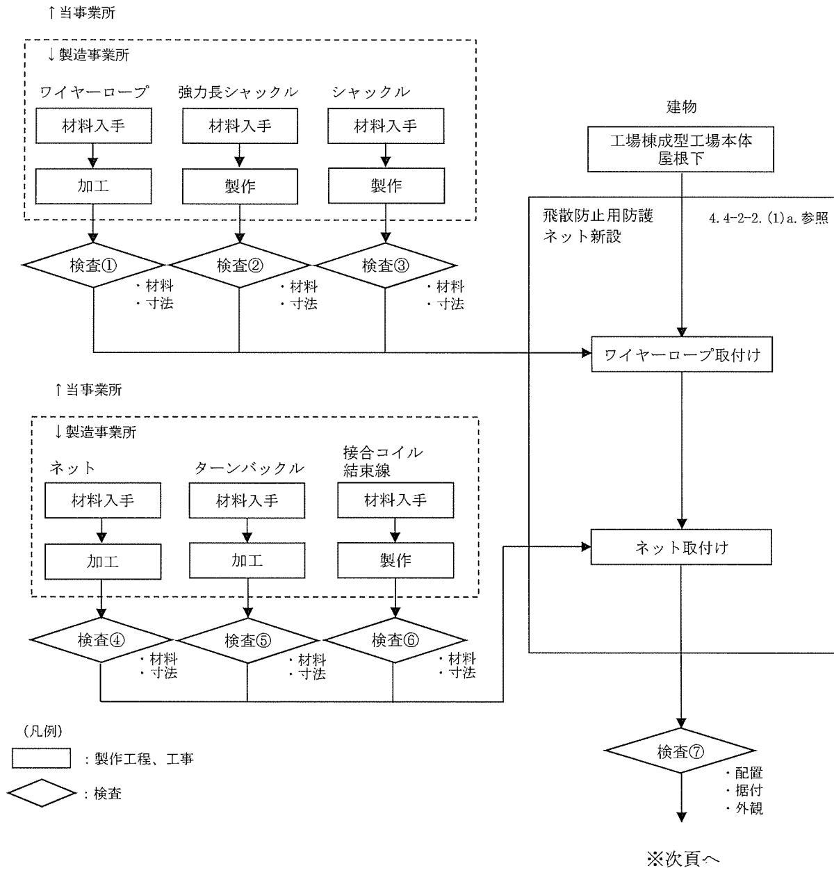
図リ 4-2-2 工場棟成型工場 緊急対策設備(2)飛散防止用防護ネット新設 の手順フロー図 (1/2)
