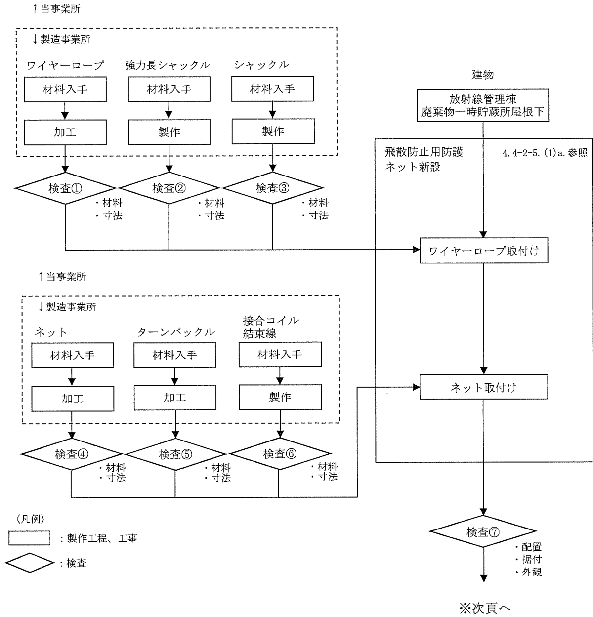
図リ 4-2-5 放射線管理棟 緊急対策設備(2)飛散防止用防護ネット新設 の手順フロー図 (1/2)
