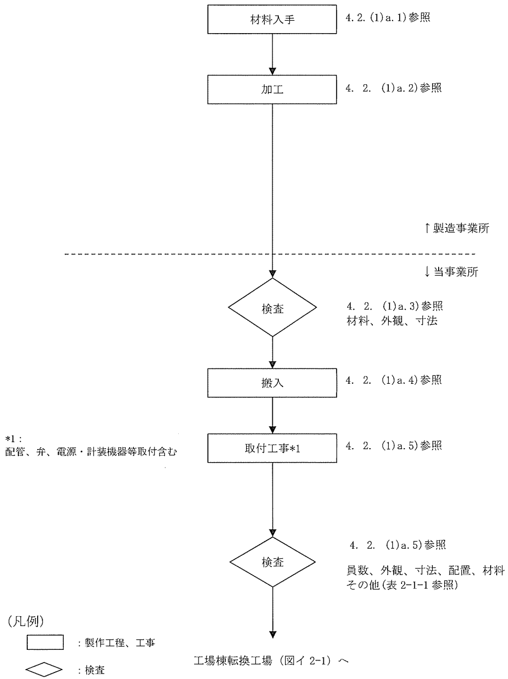
図イ 2-2-1 工事の手順フロー図 (新設する場合)
