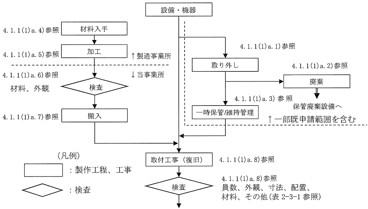
工場棟転換工場 (図イ 2-1)
