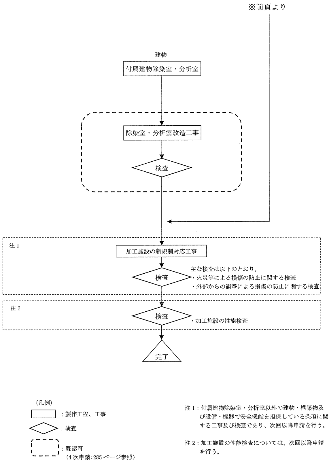
図リ 4-2-6 付属建物除染室・分析室 緊急対策設備(2)飛散防止用防護ネット(除染室)新設の手順フロー図 (2/2)
