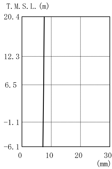
図 4-11(1) 最大応答変位 (基準地震動 S s , 鉛直方向)
