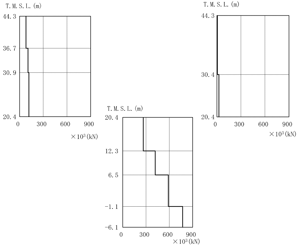
図 4-8 最大応答せん断力（基準地震動 S s , EW 方向）
