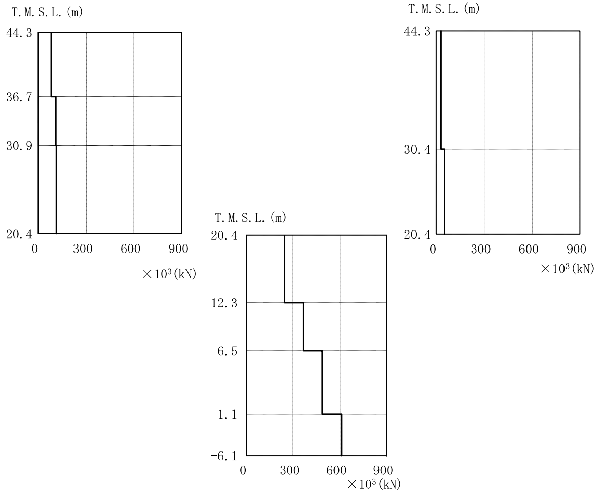
図 4-4 最大応答せん断力（基準地震動 S s ，NS 方向）
