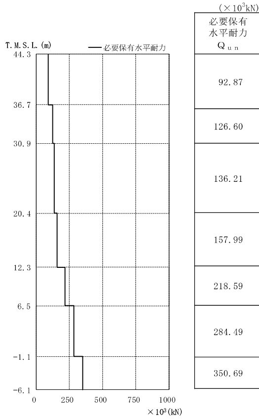
图 4-21 必要保有水平耐力 Q_{un} (EW 方向)
