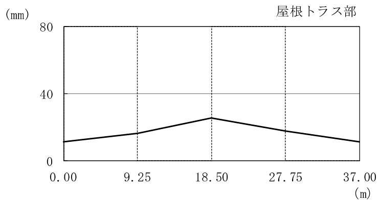
図 4-14(2) 最大応答変位 (基準地震動 S s , NS 方向, 誘発上下動, 屋根トラス)
