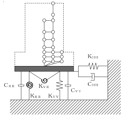
図 3-18 誘発上下動を考慮する場合の地震応答解析モデルの概念図
