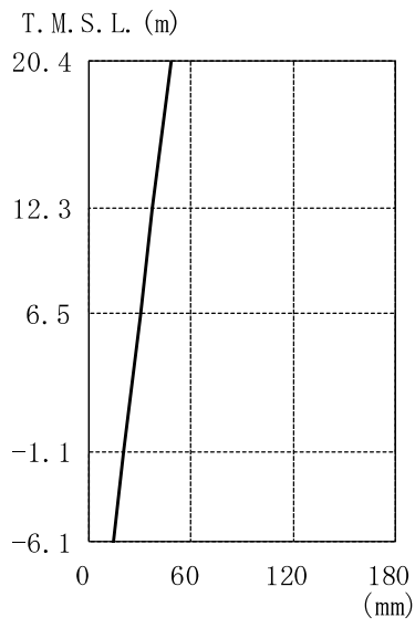
図 4-3 最大応答変位（基準地震動 S s ，NS 方向）
