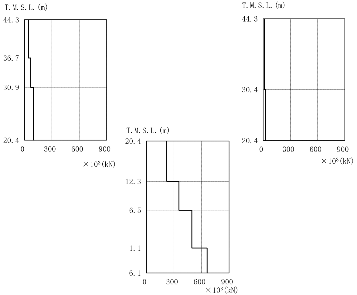
図 4-12 最大応答軸力（基準地震動 S s ，鉛直方向）
