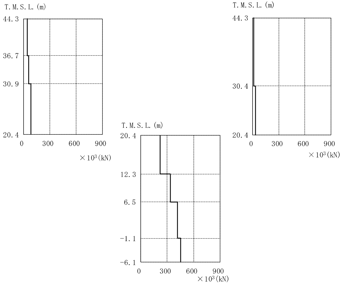
図 4-15 最大応答軸力 (基準地震動 S s , NS 方向, 誘発上下動)
