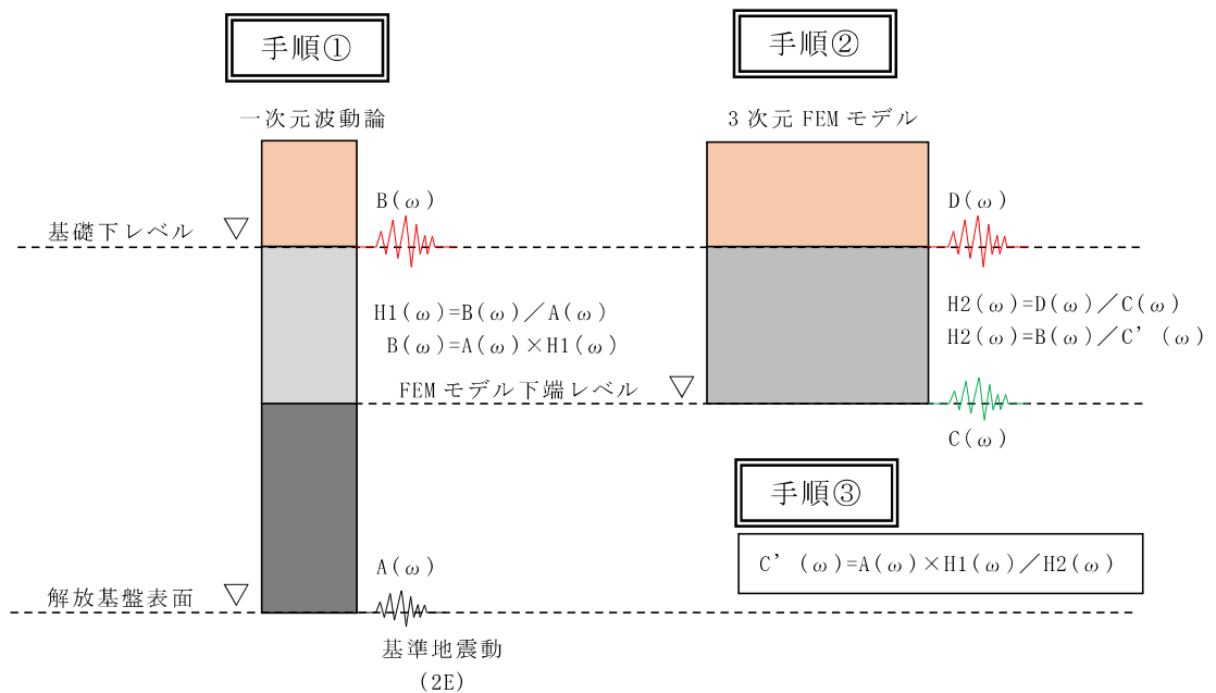
図 3-5 FEM モデルへの入力地震動の補正方法
