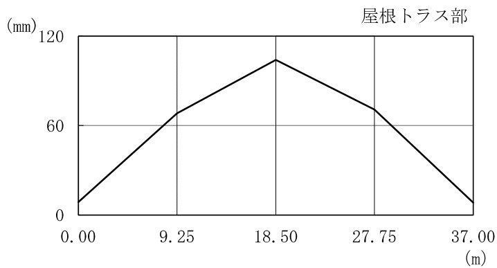
図 4-11(2) 最大応答変位 (基準地震動 S s , 鉛直方向, 屋根トラス)
