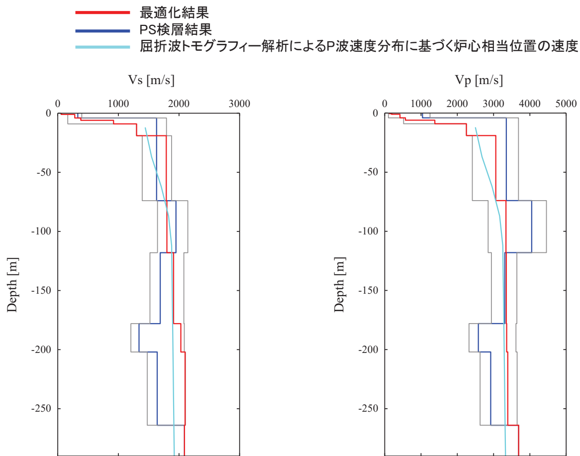
《 推定された鉛直分布 Vs 》
