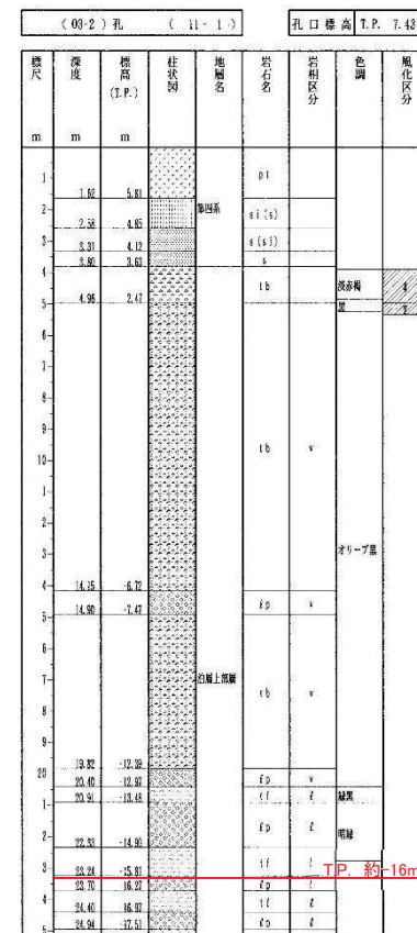
地質柱状図及びピコア写真
