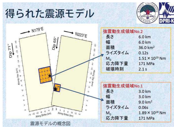
震源モデル
