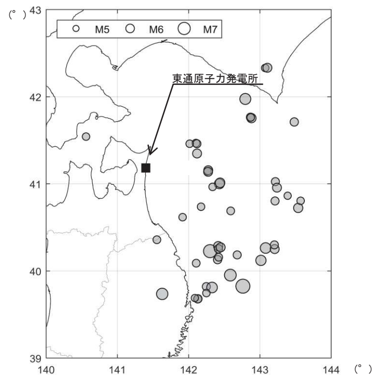
震央分布
