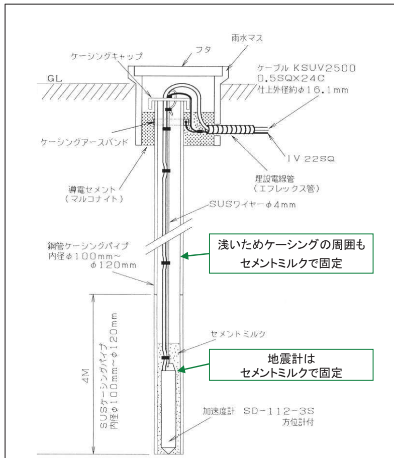
既設地震計[T.P.+2m]の設置概要図
