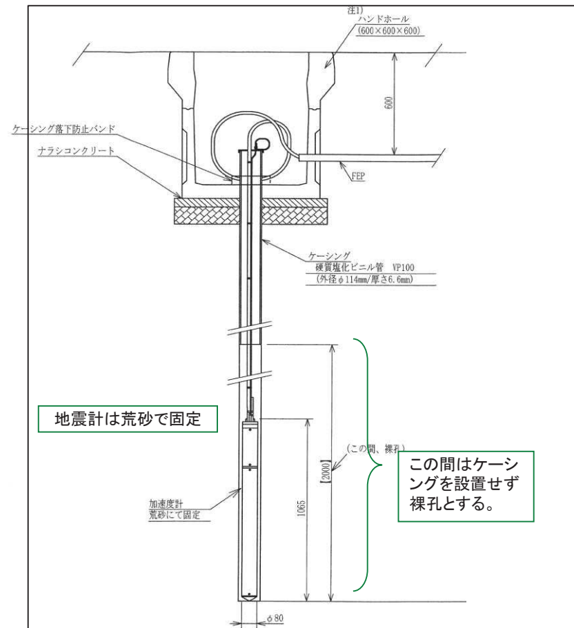
増設地震計[T.P.+2m]の設置概要図
