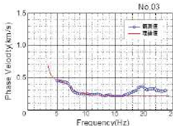
観測点No.3における分散曲線と推定S波速度構造
