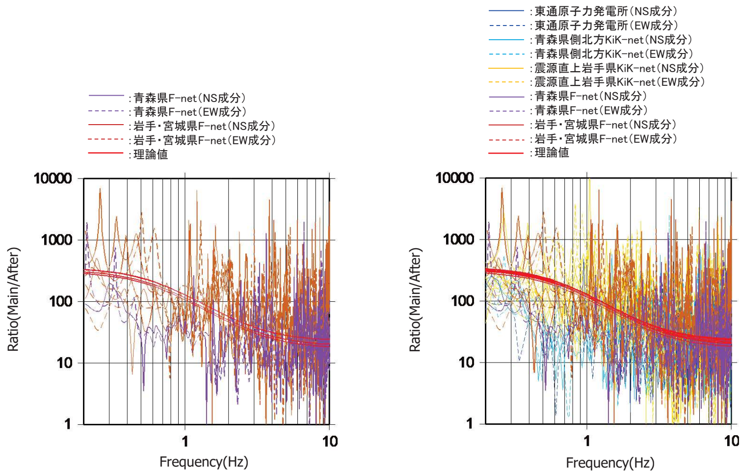
(1) F-net観測点
