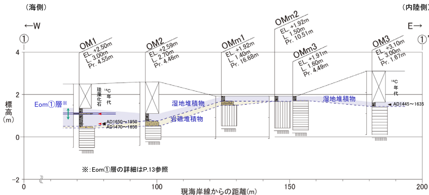
①-①'断面図
