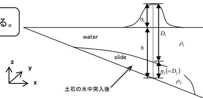
二層流モデル中の変数の定義
