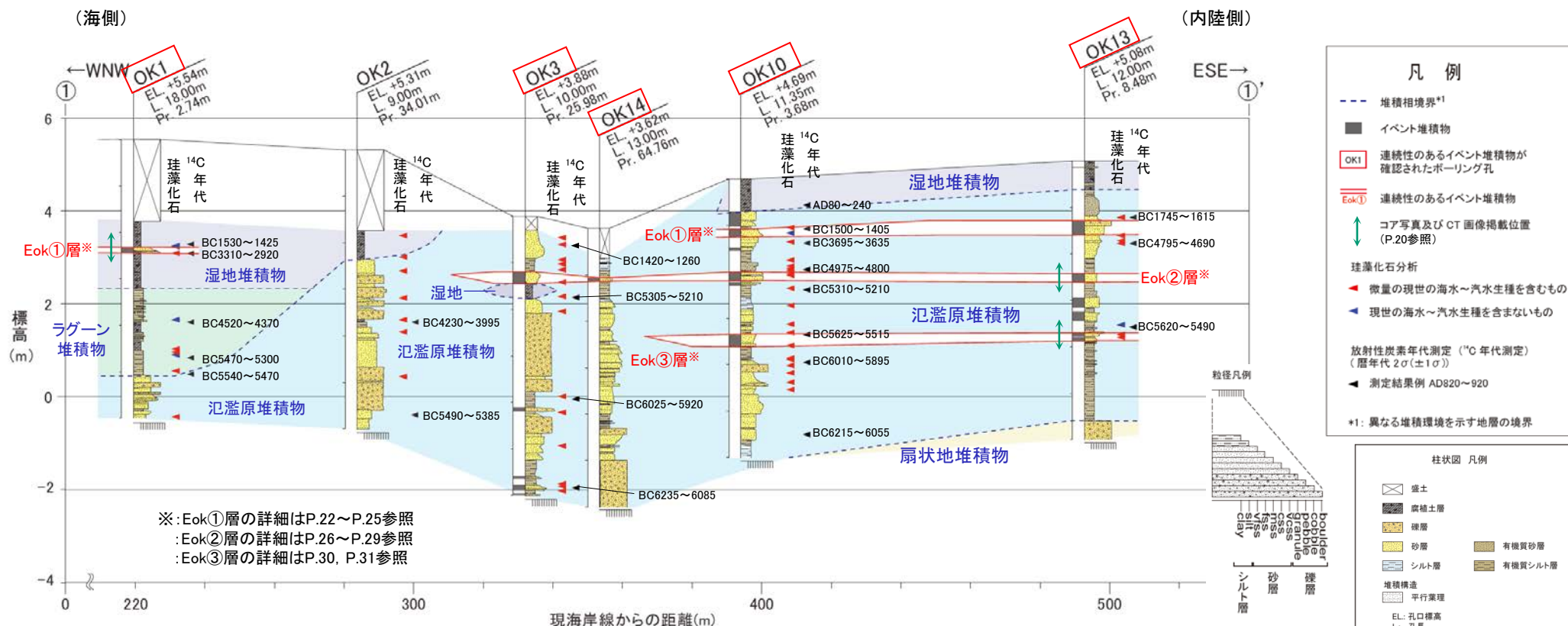
①-①'断面図
