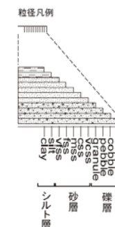
柱状図 凡例
