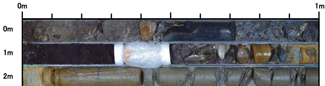
ボーリングコア写真
