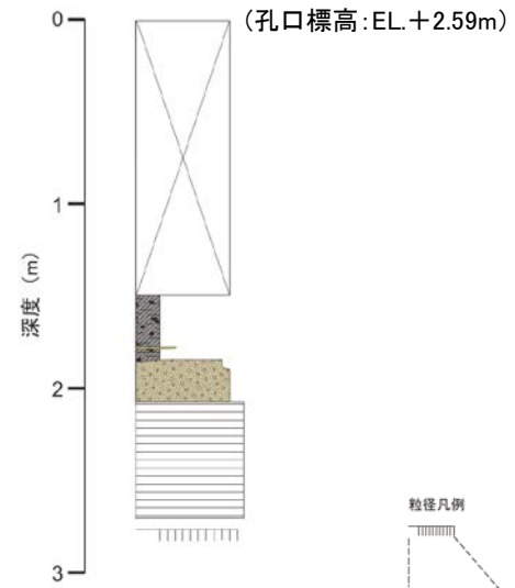
統合柱状図
