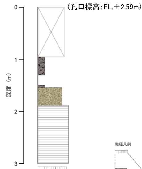
柱状図
