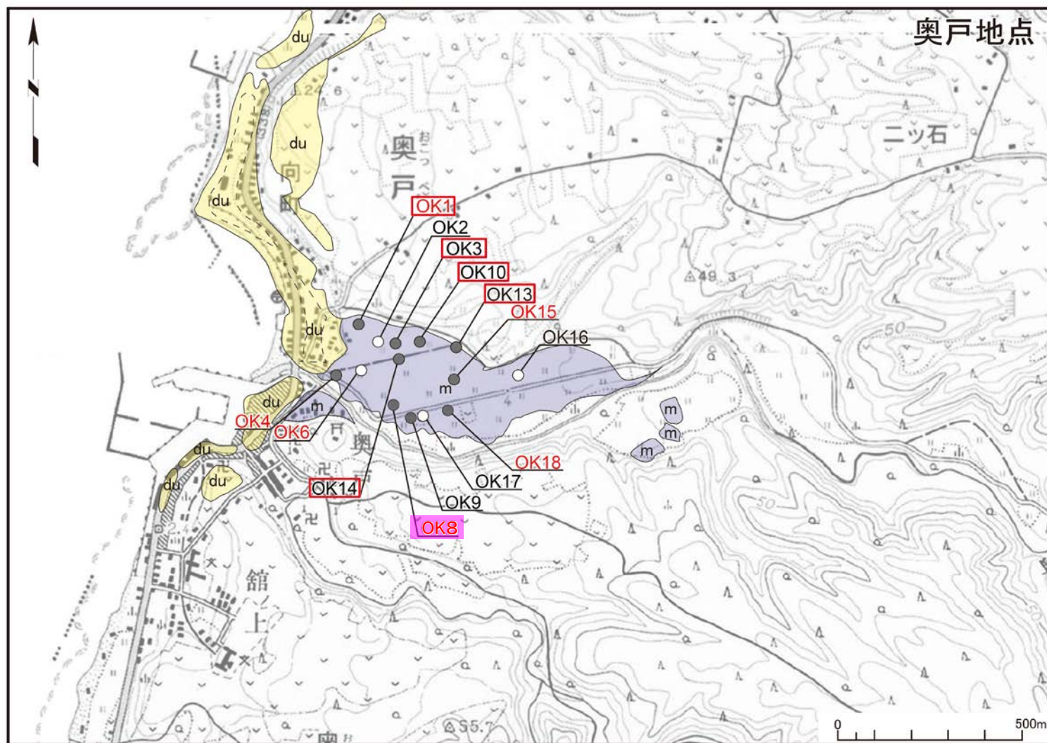
奥戸地点の調査位置図
