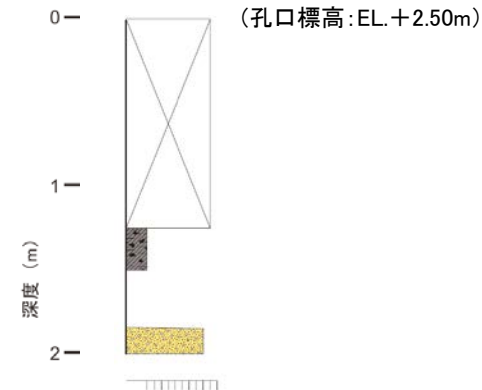
柱状図
