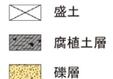
柱状図 凡例
