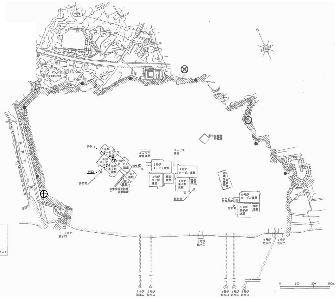
第1図 実効線量計算地点図
