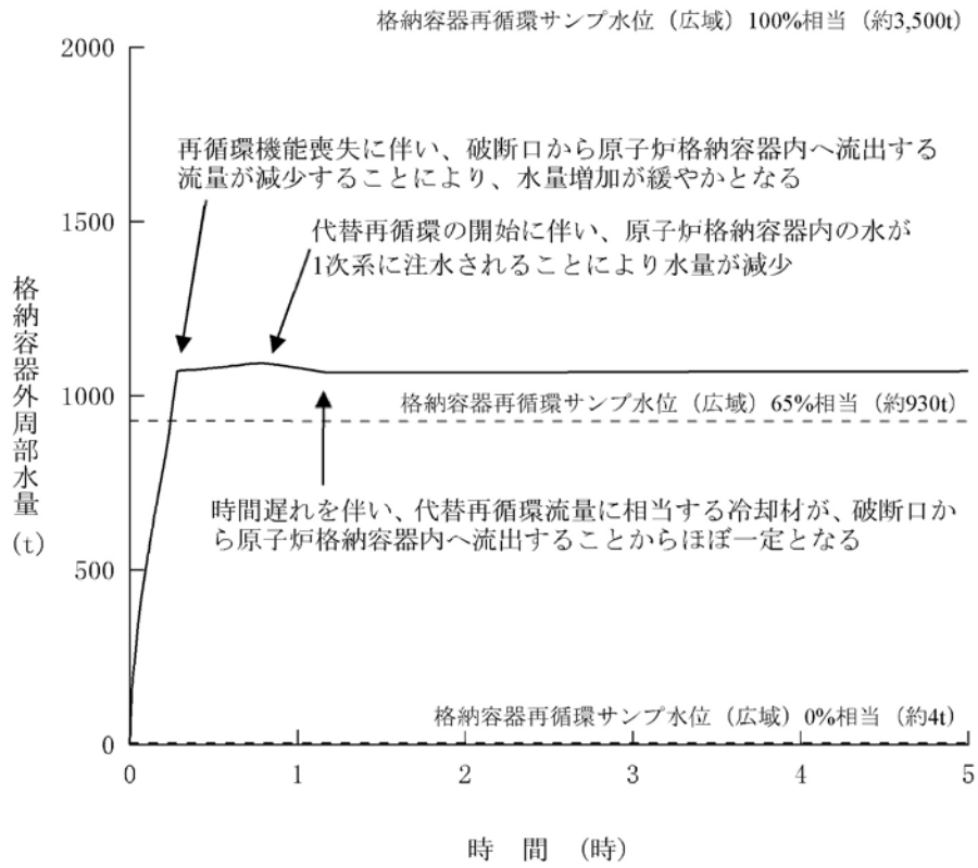
第1.15-311図 格納容器外周部水量の推移
