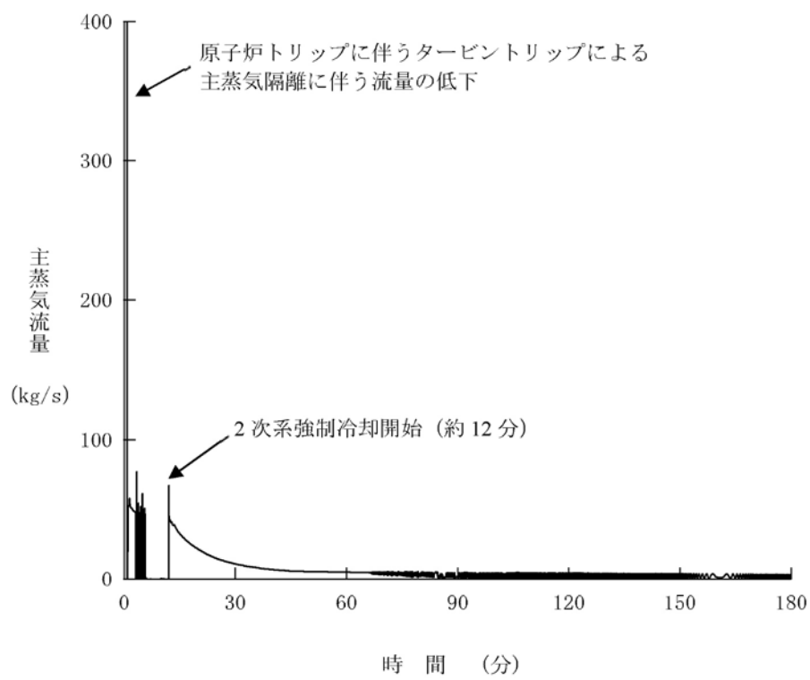
第1.15-284図 主蒸気流量の推移(2inch破断)
