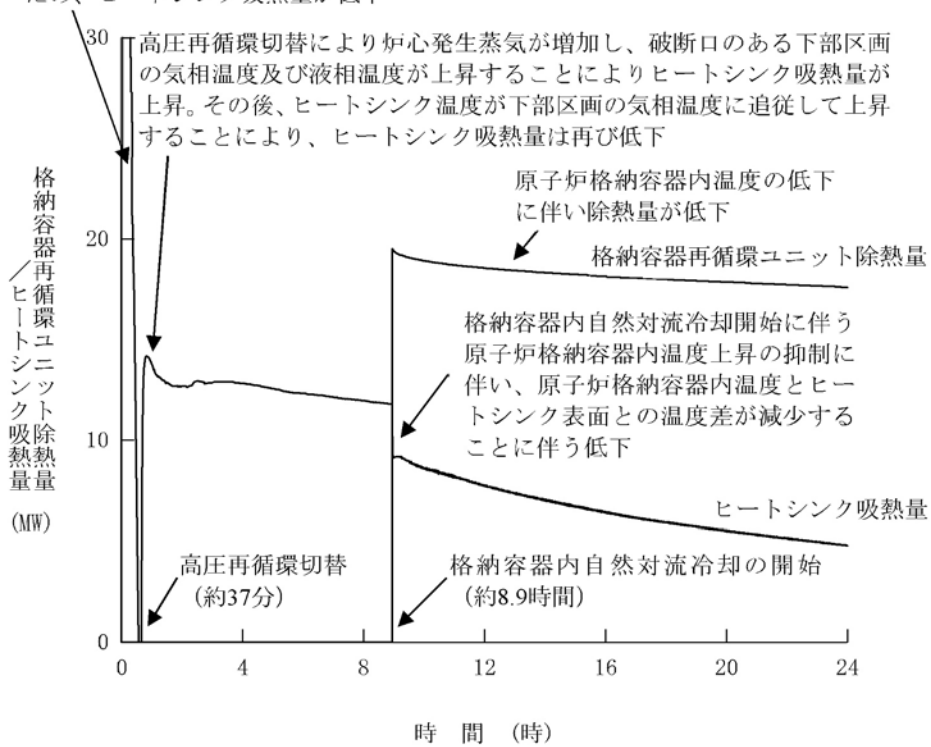
第1.15-219図 原子炉格納容器からの除熱量の推移
