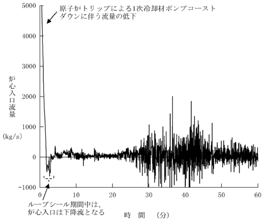
第1.15-260図 炉心入口流量の推移 (6inch破断)
