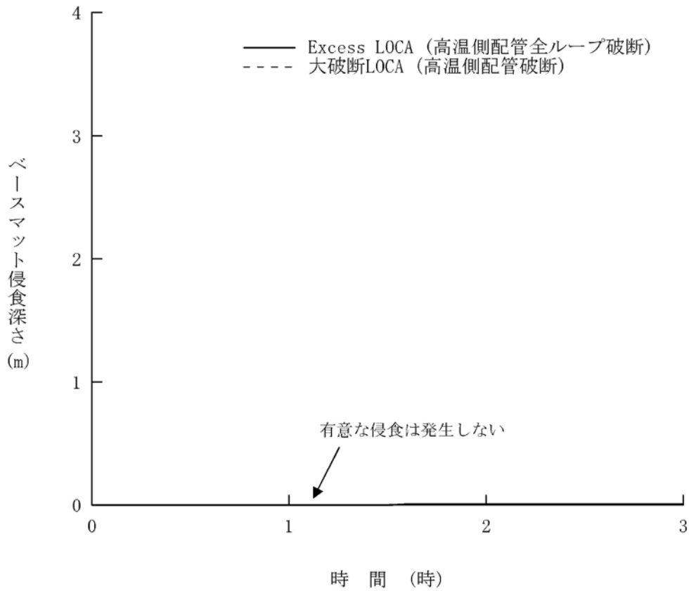
第1.15-442図 ベースマット侵食深さの推移 (高温側配管全ループ破断時の影響確認)
