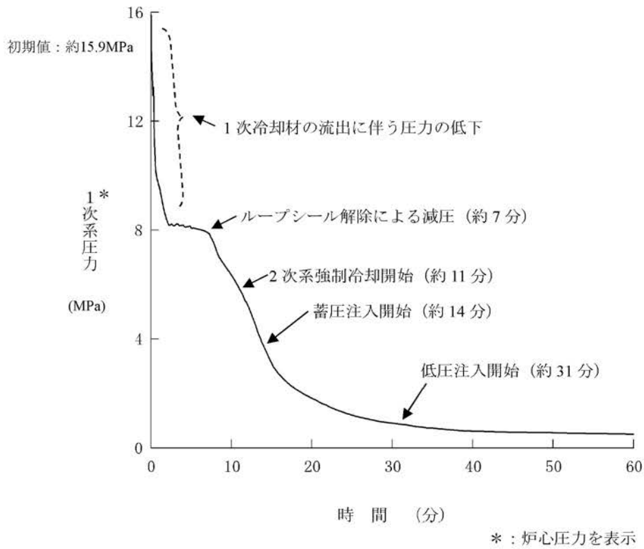
第1.15-265図 1次系圧力の推移(4inch破断)
