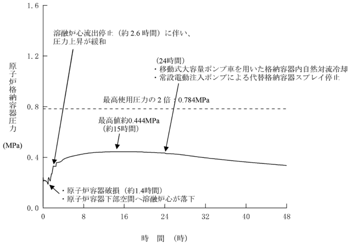
第1.15-385図 原子炉格納容器圧力の推移
