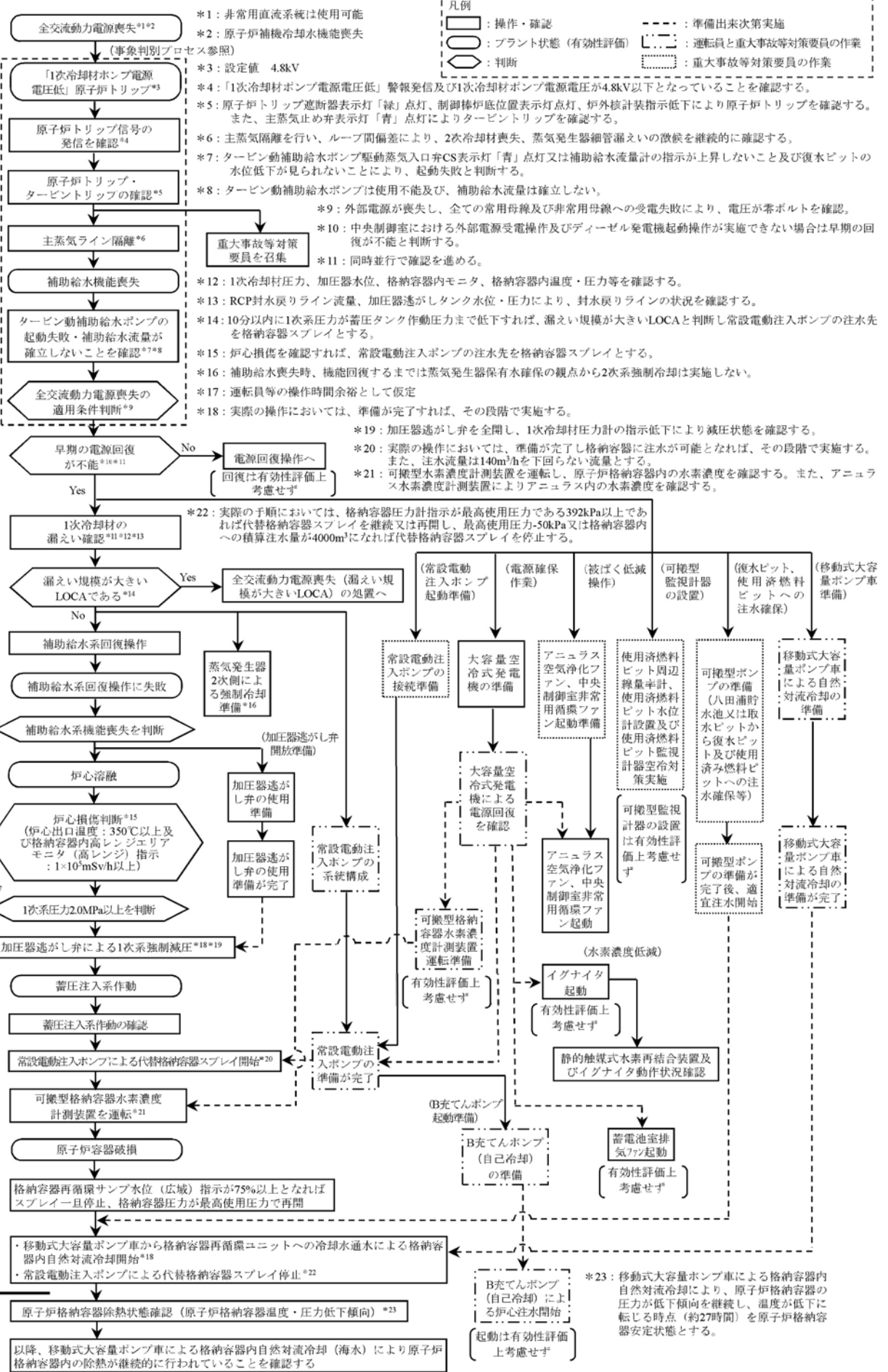
第1.15-409図 「雰囲気圧力・温度による静的負荷(格納容器過温破損)」の事象進展 (外部電源喪失時に非常用所内交流動力電源が喪失し、補助給水機能が喪失する事故)
