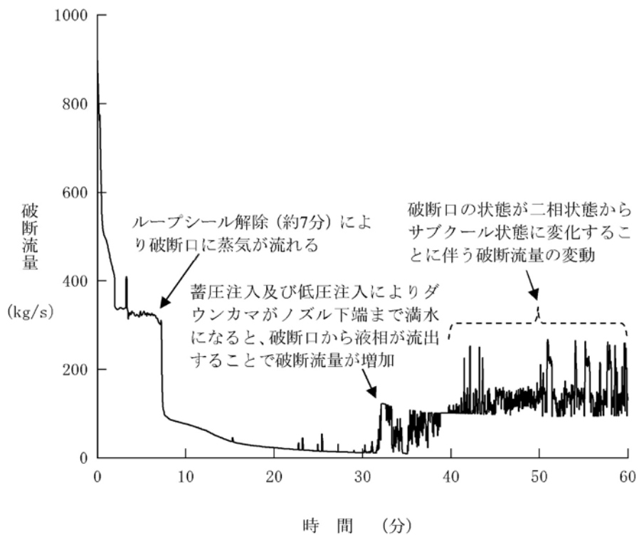
第1.15-268図 破断流量の推移(4inch破断)
