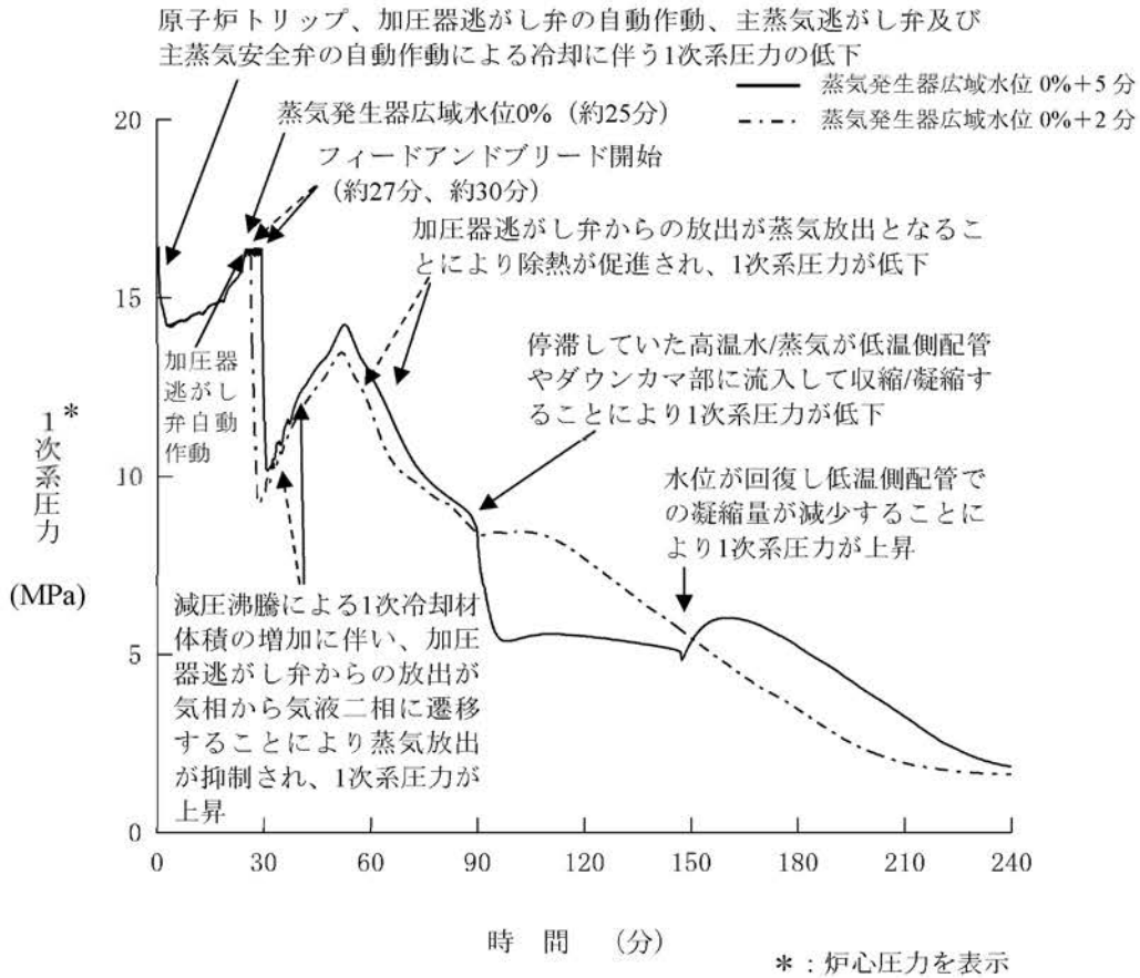
第1.15-157図 1次系圧力の推移(開始が早くなる場合)
