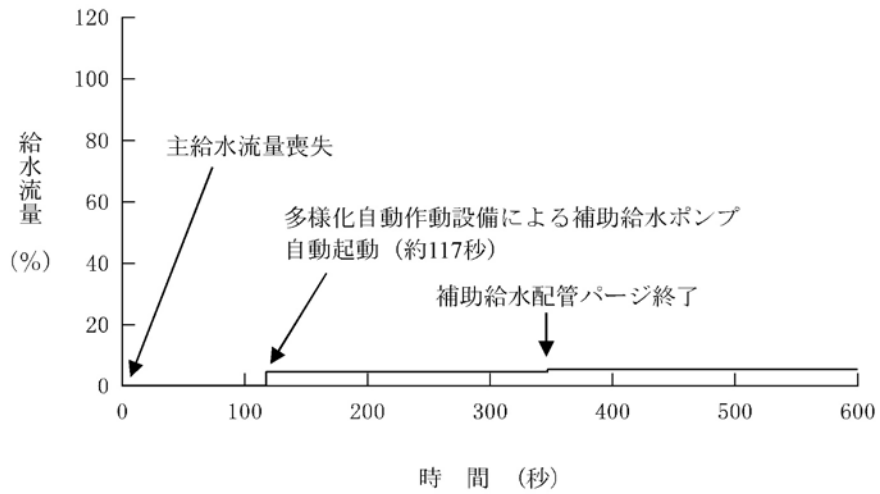
第1.15-250図 給水流量の推移 (負荷の喪失時に原子炉トリップ機能が喪失する事故)
