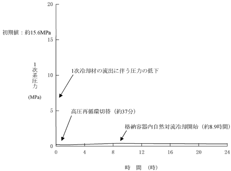
第1.15-211図 1次系圧力の推移
