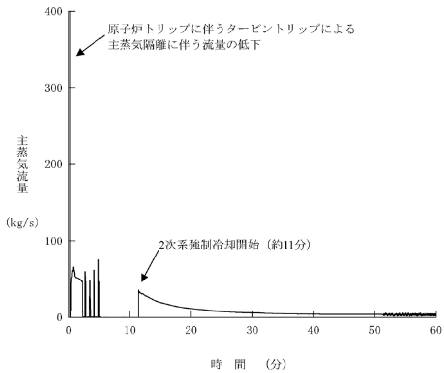
第1.15-274図 主蒸気流量の推移(4inch破断)
