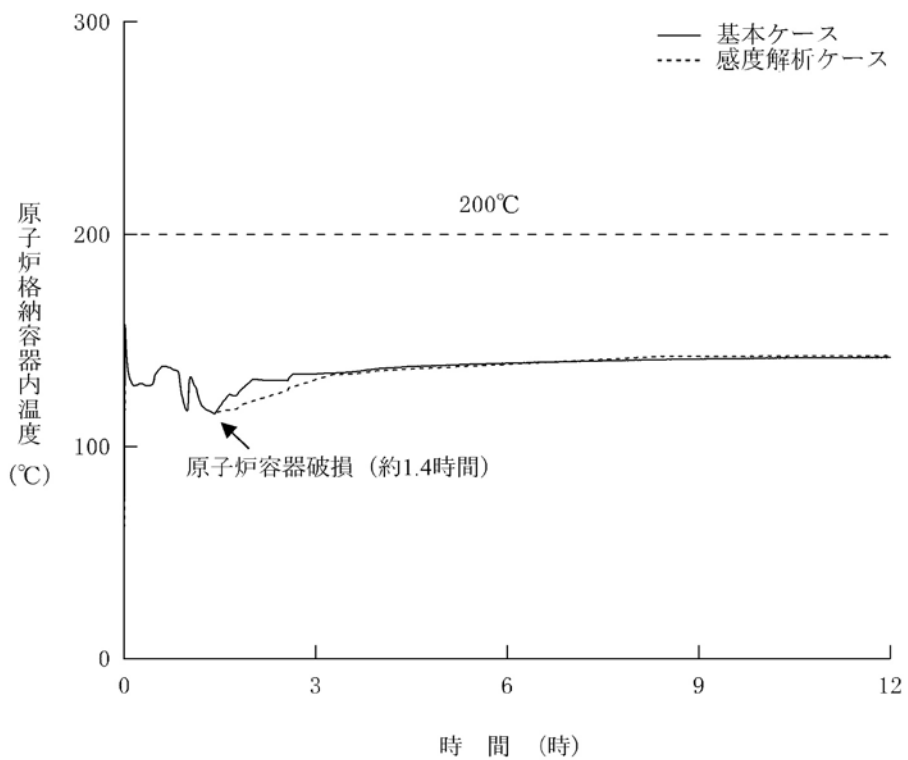
第1.15-393図 原子炉格納容器内温度の推移 (溶融炉心・コンクリート相互作用による影響確認)
