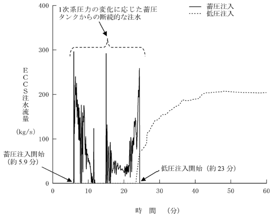
第1.15-257図 ECCS注水流量の推移(6inch破断)
