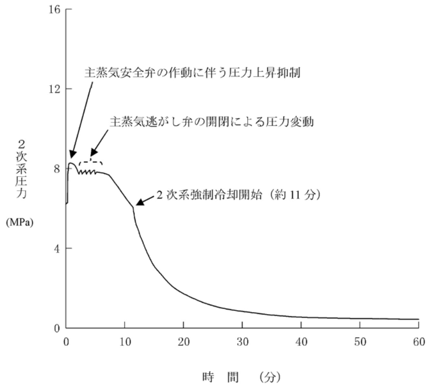
第1.15-272図 2次系圧力の推移(4inch破断)
