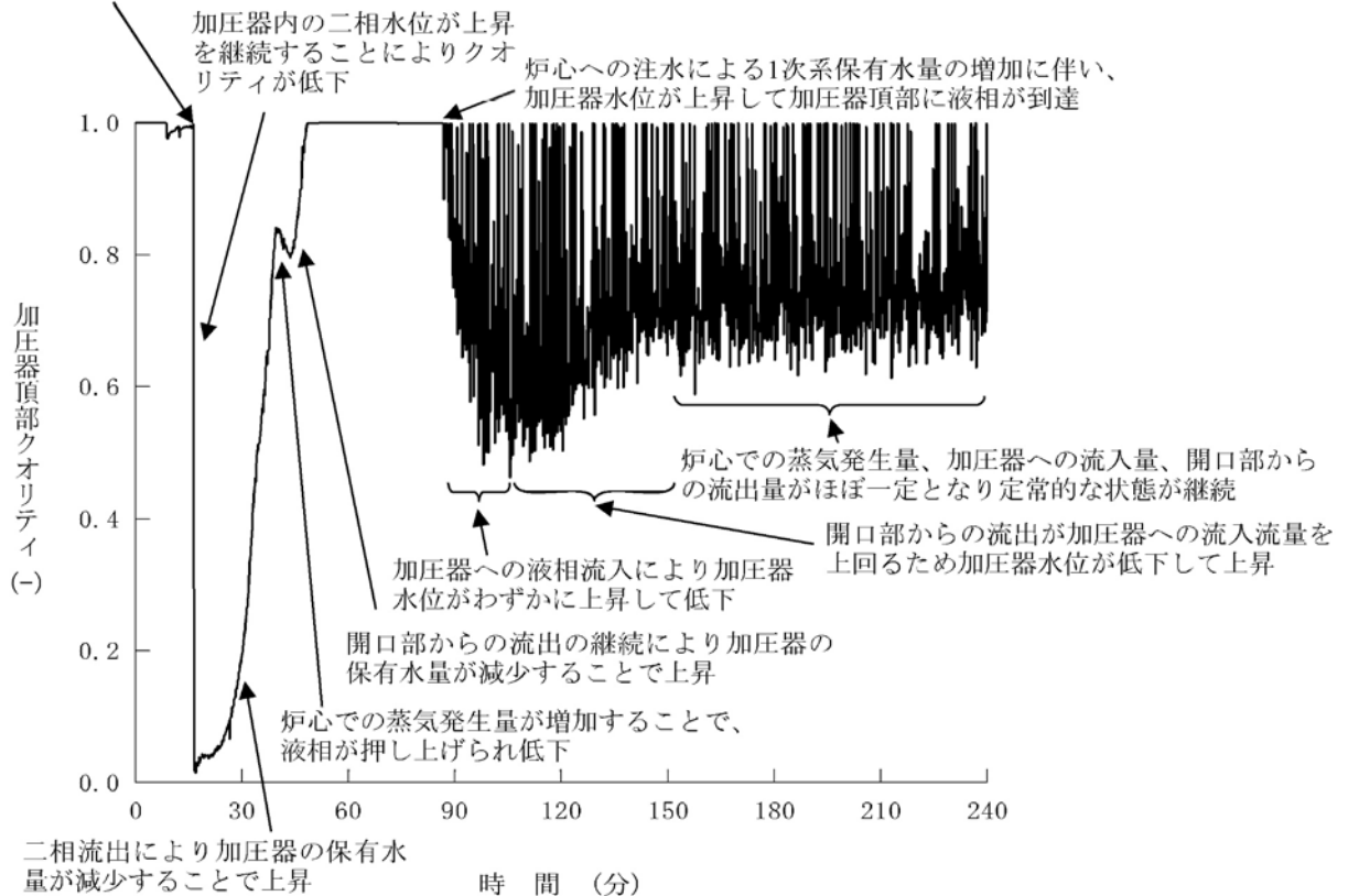
第1.15-361図 加圧器頂部クオリティの推移
