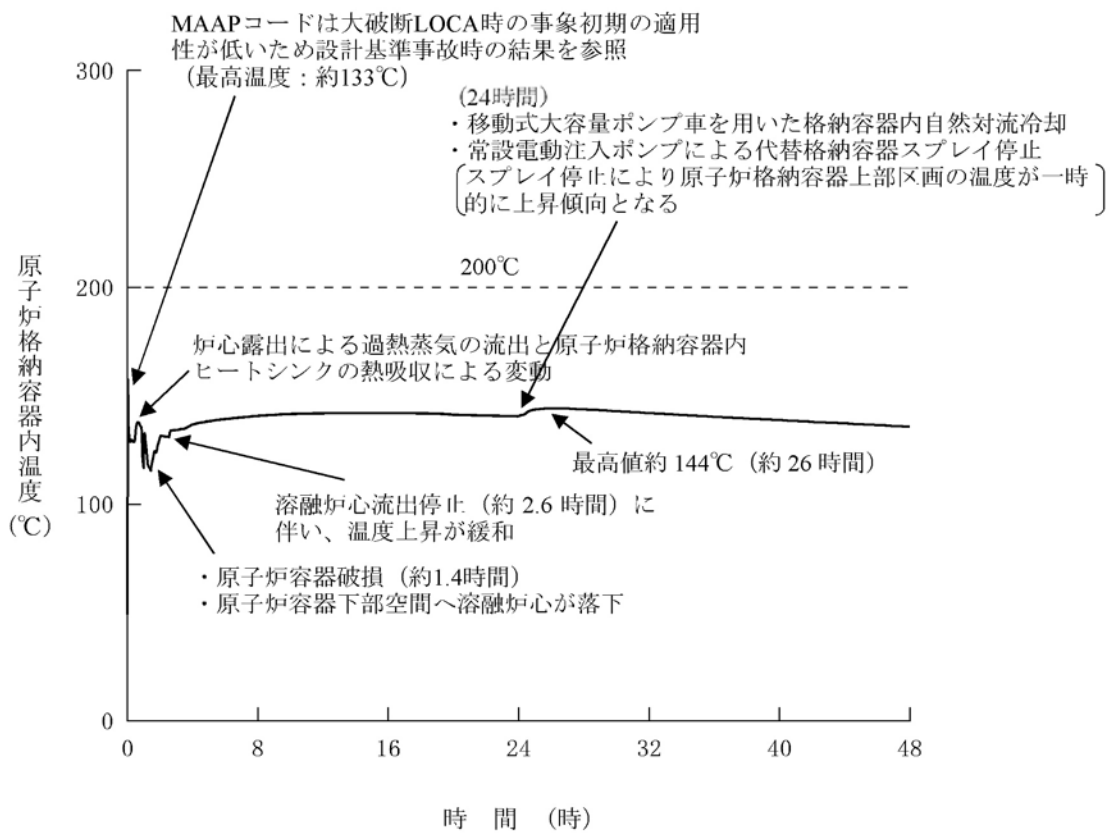
第1.15-386図 原子炉格納容器内温度の推移
