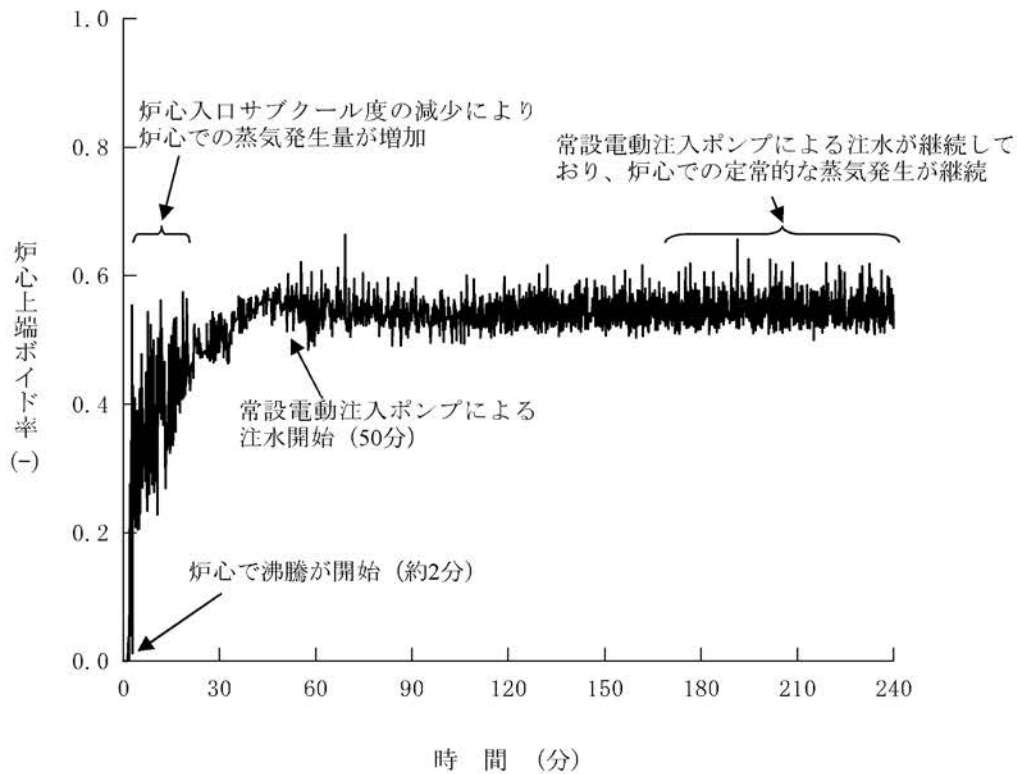
第1.15-359図 炉心上端ボイド率の推移
