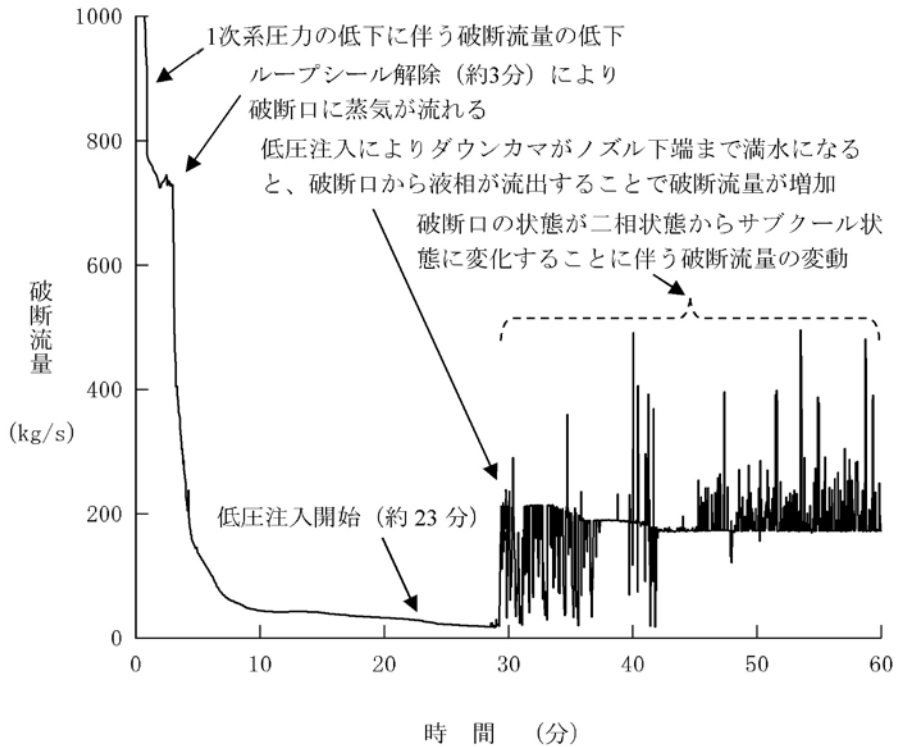
第1.15-258図 破断流量の推移(6inch破断)
