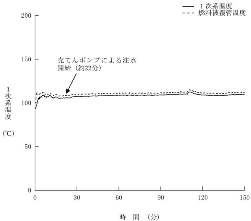
第1.15-376図 1次系温度の推移
