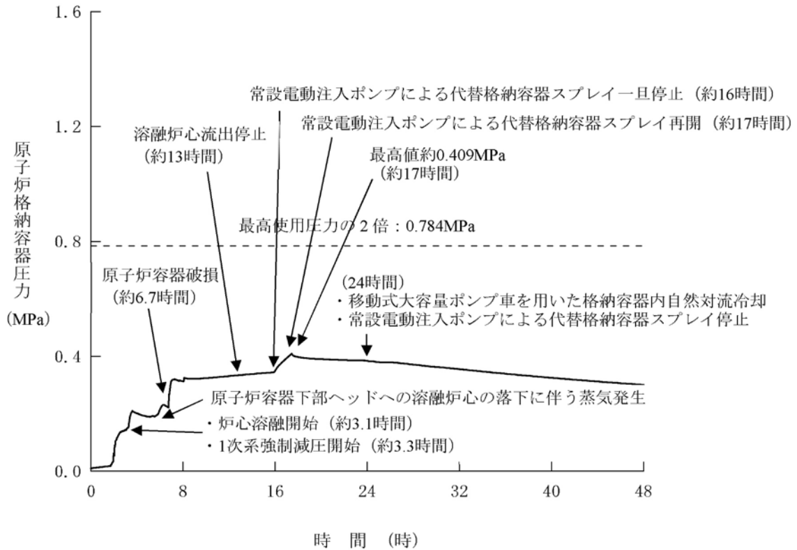
第1.15-412図 原子炉格納容器圧力の推移
