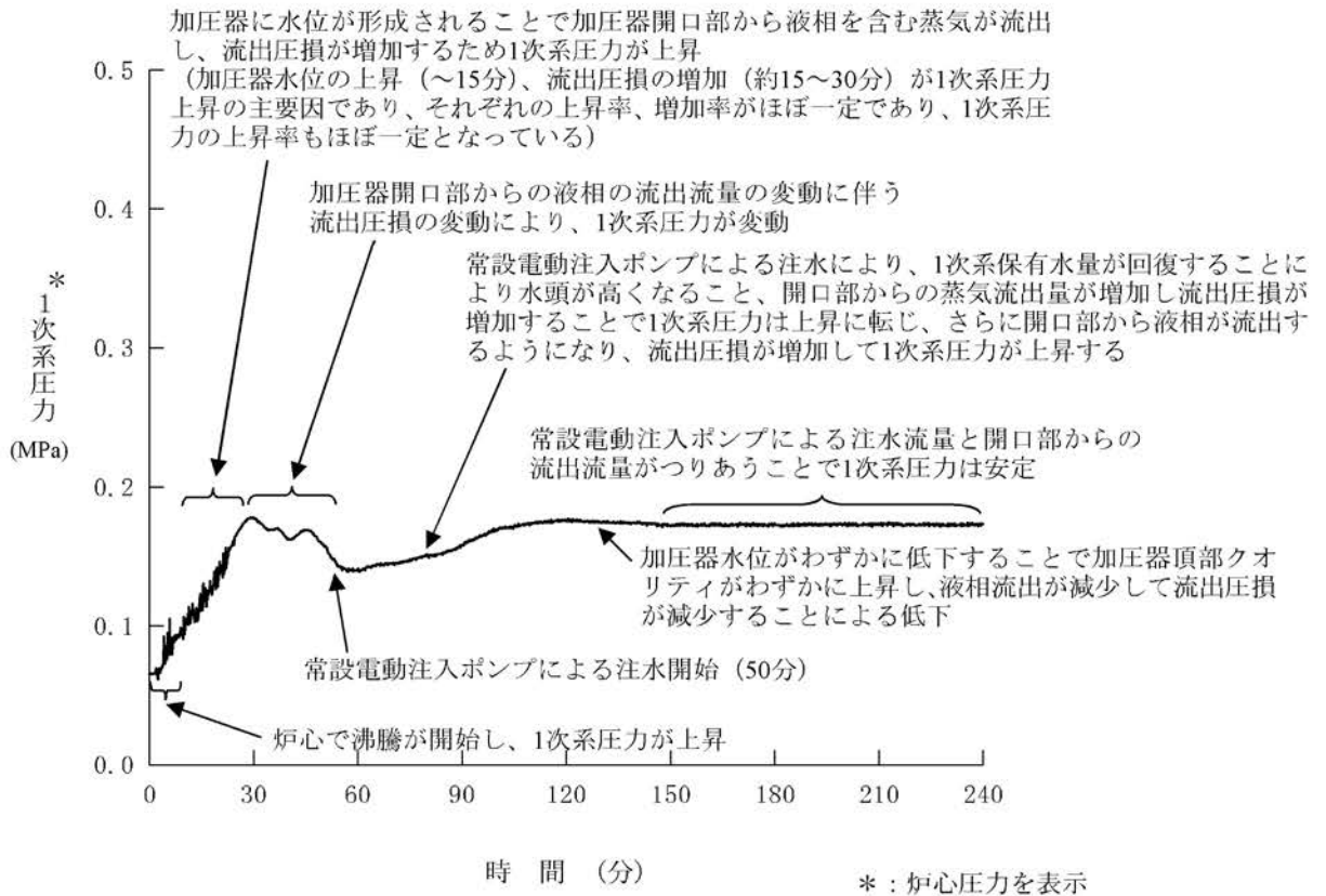
第1.15-358図 1次系圧力の推移
