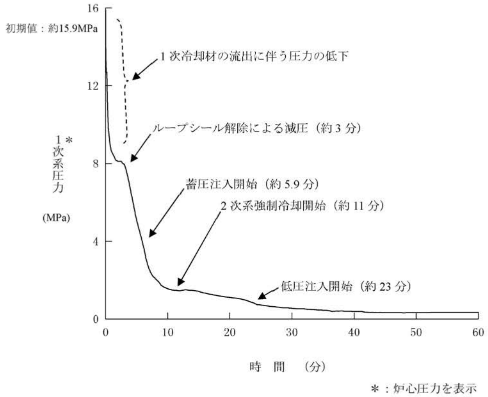
第1.15-255図 1次系圧力の推移(6inch破断)
