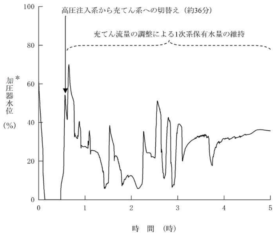
第1.15-340図 加圧器水位の推移 (蒸気発生器伝熱管破損時に破損側蒸気発生器の隔離に失敗する事故)
