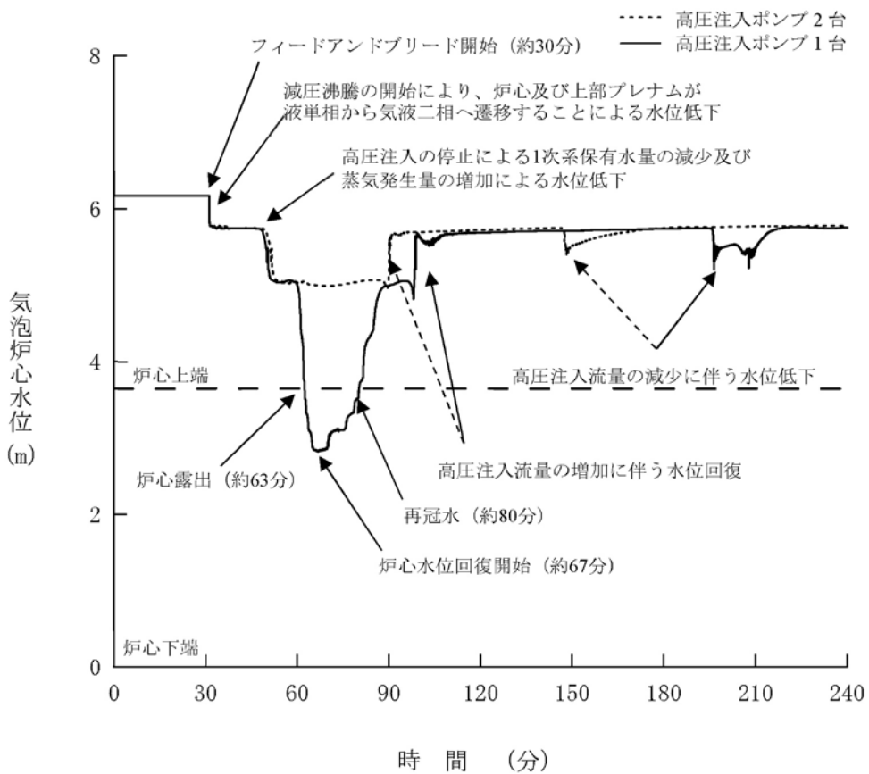
第1.15-155図 気泡炉心水位の推移 (高圧注入ポンプ1台の場合)
