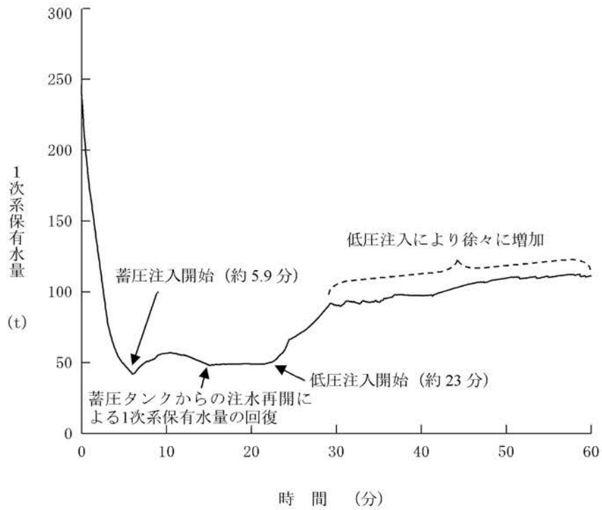
第1.15-256図 1次系保有水量の推移(6inch破断)
