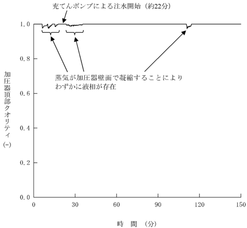
第1.15-371図 加圧器頂部クオリティの推移
