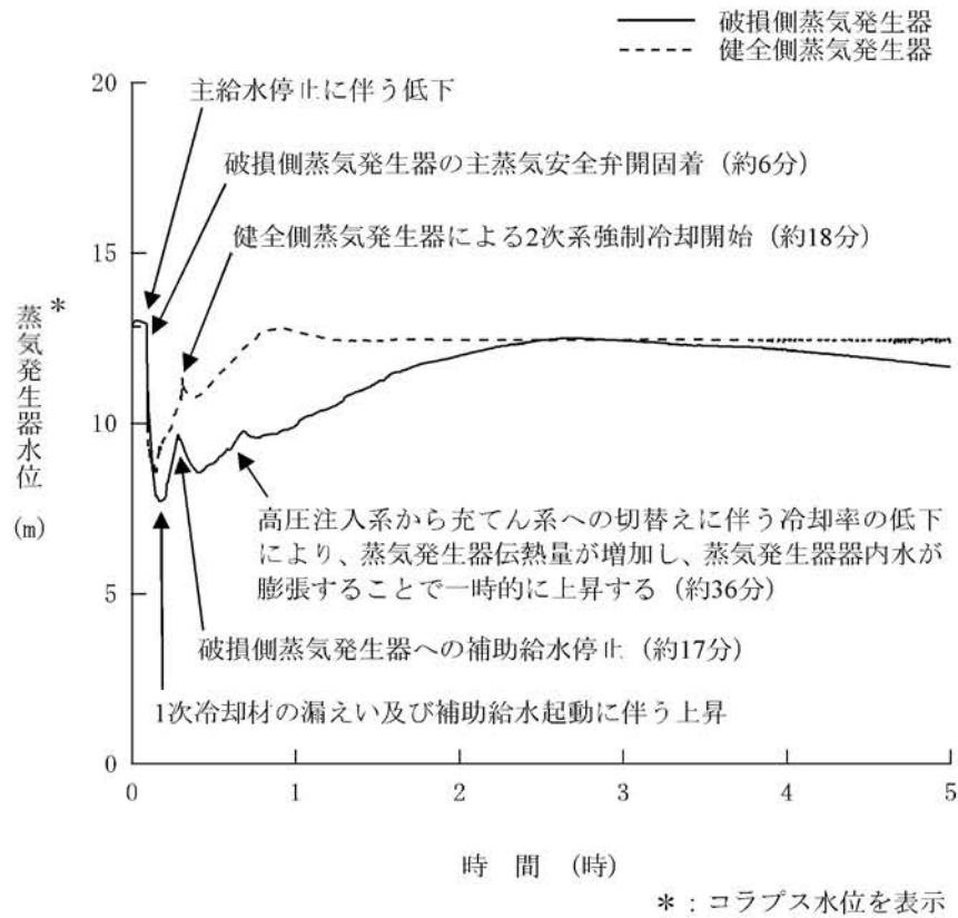
第1.15-343図 蒸気発生器水位の推移 (蒸気発生器伝熱管破損時に破損側蒸気発生器の隔離に失敗する事故)
