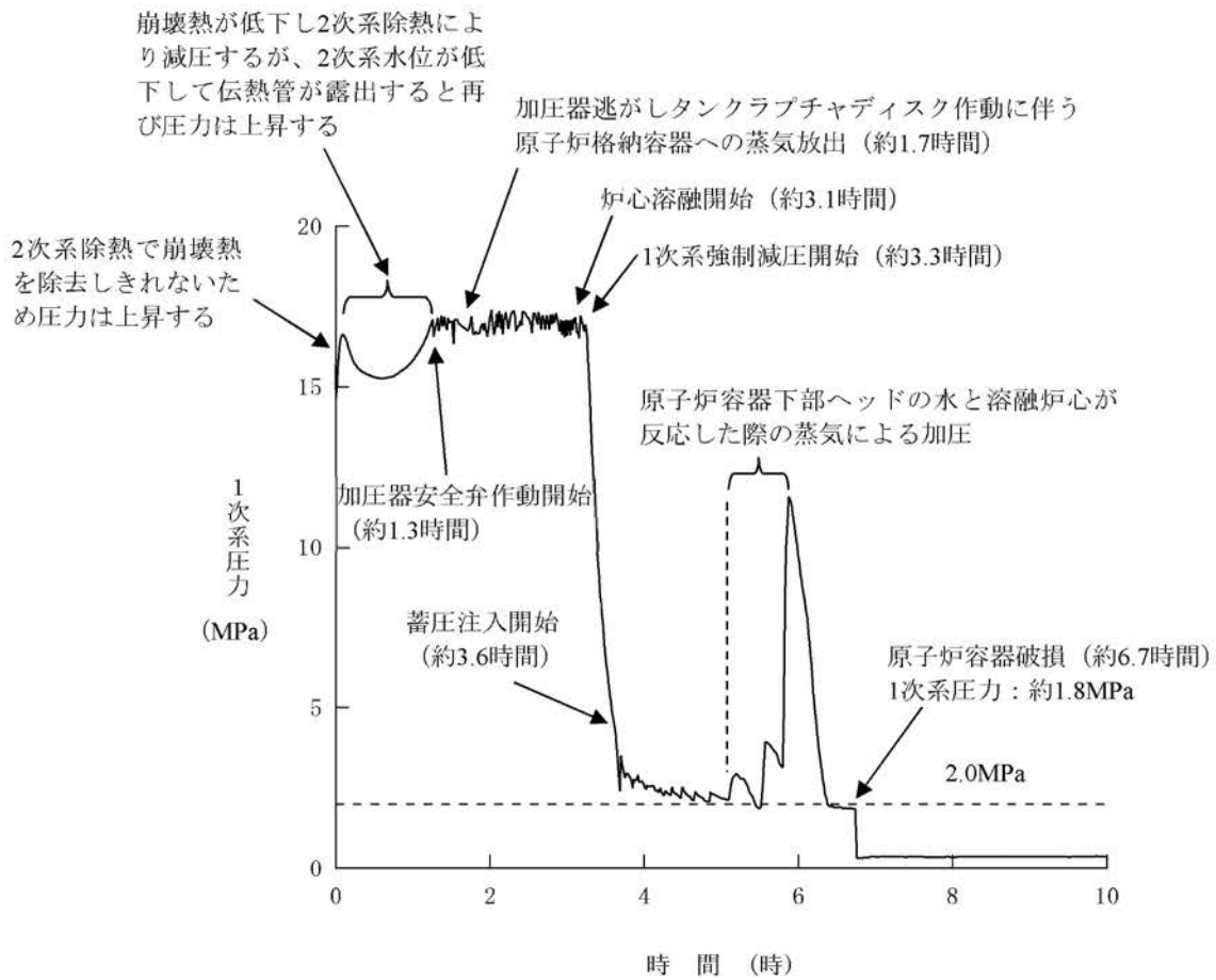
第1.15-422図 1次系圧力の推移
