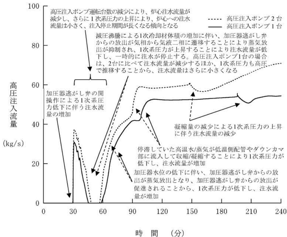
第1.15-153図 高圧注入流量の推移(高圧注入ポンプ1台の場合)
