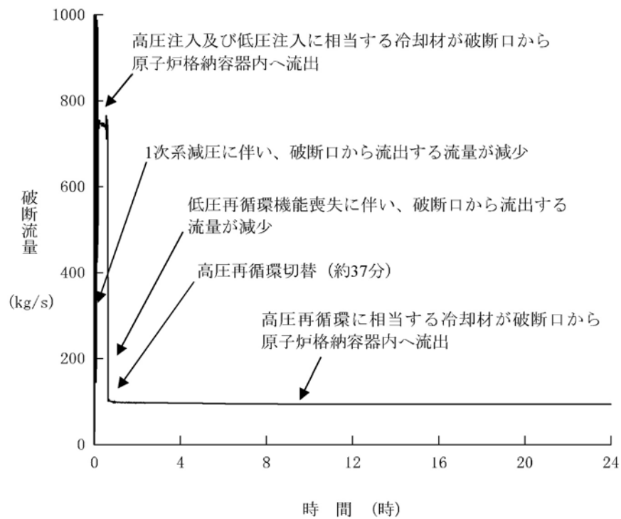
第1.15-212図 破断流量の推移
