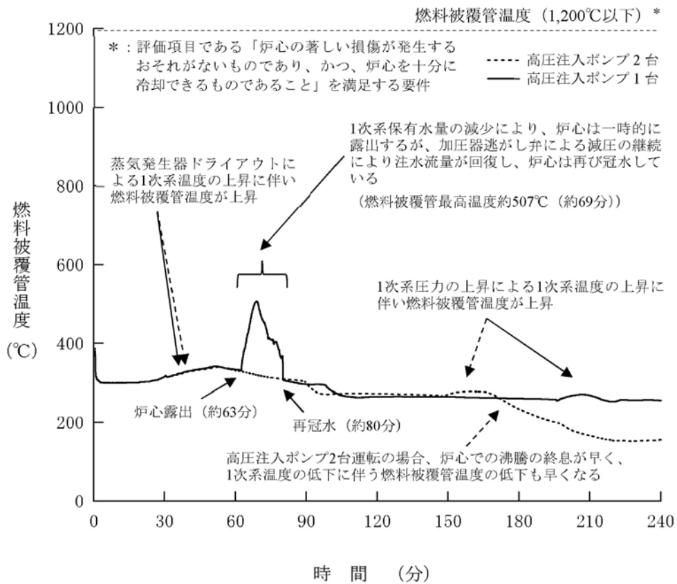
第1.15-156図 燃料被覆管温度の推移 (高圧注入ポンプ1台の場合)
