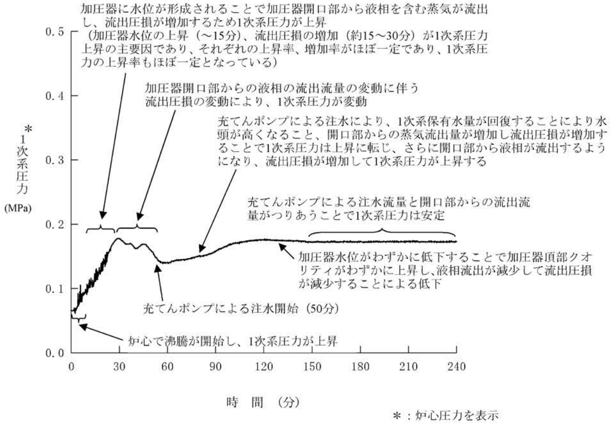
第1.15-348図 1次系圧力の推移
