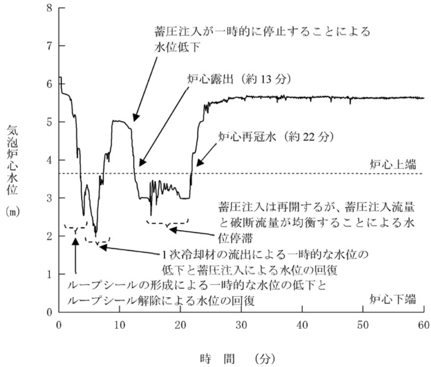
第1.15-259図 気泡炉心水位の推移 (6inch破断)
