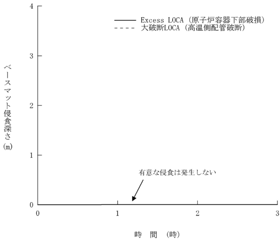
第1.15-446図 ベースマット侵食深さの推移 (原子炉容器下端における破損時の影響確認)
