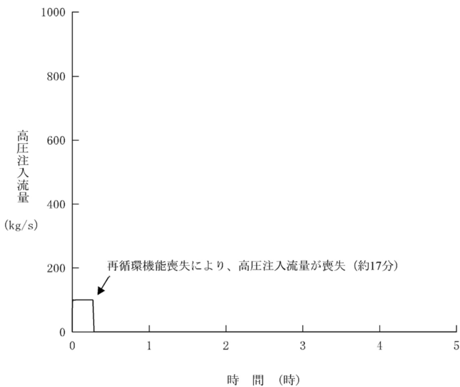
第1.15-306図 高圧注入流量の推移
