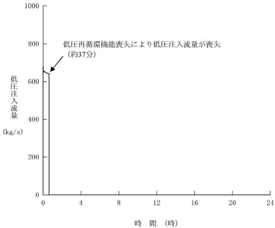
第1.15-214図 低圧注入流量の推移
