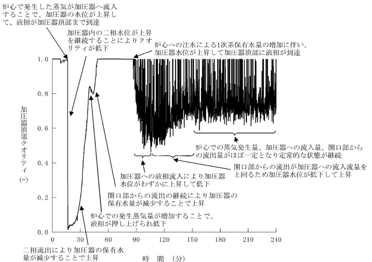
第1.15-351図 加圧器頂部クオリティの推移
