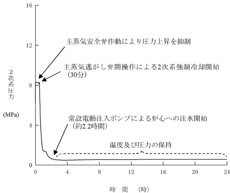
第1.15-180図 2次系圧力の推移 (RCPシールLOCAが発生する場合)
