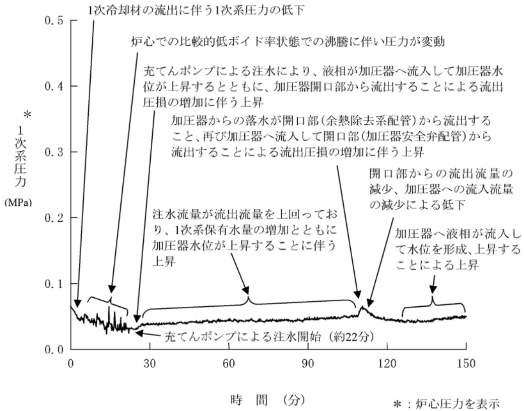
第1.15-368図 1次系圧力の推移
