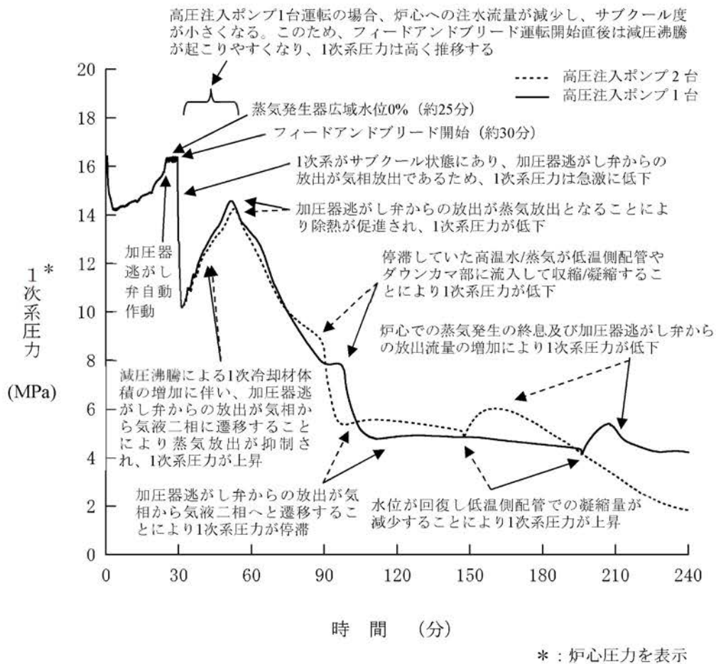
第1.15-152図 1次系圧力の推移(高圧注入ポンプ1台の場合)
