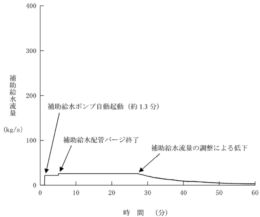
第1.15-263図 補助給水流量の推移 (6inch破断)
