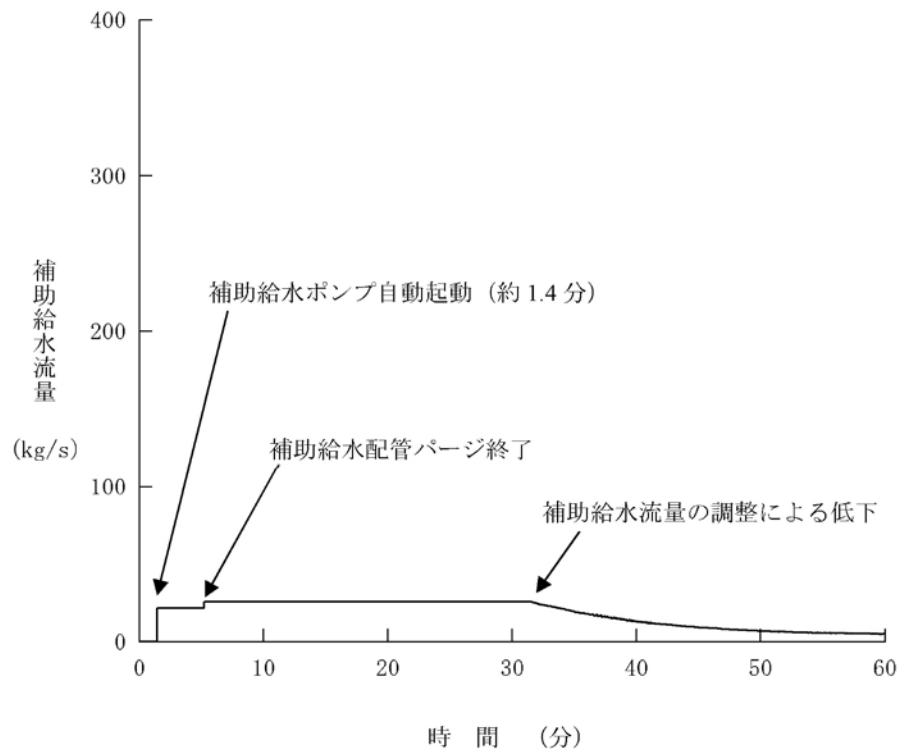
第1.15-273図 補助給水流量の推移(4inch破断)
