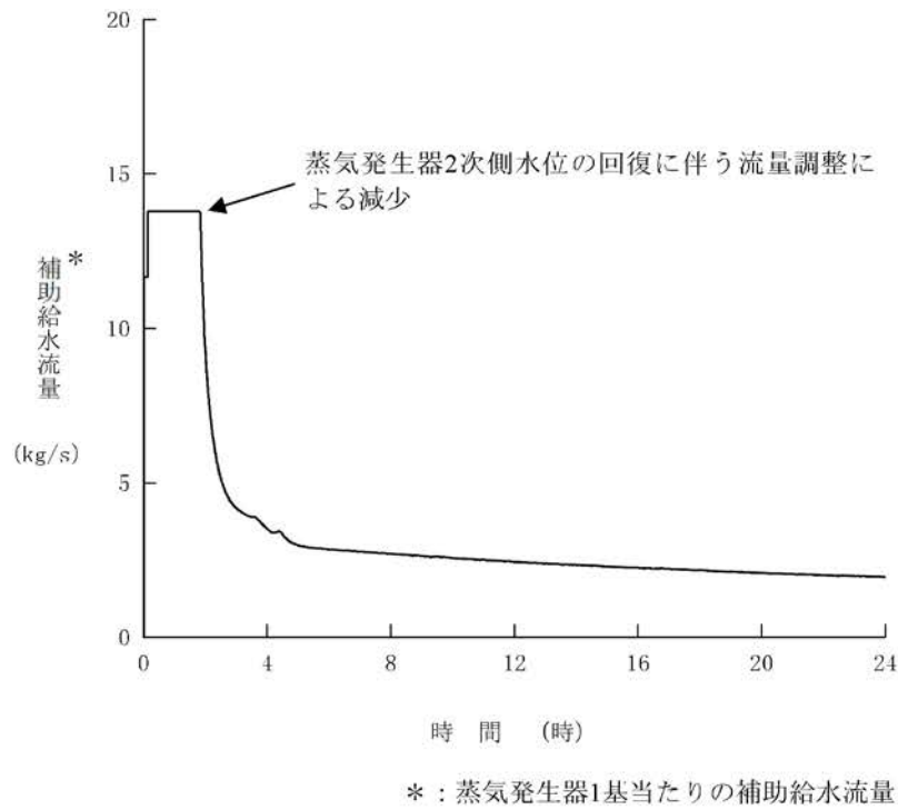
第1.15-184図 補助給水流量の推移 (RCPシールLOCAが発生する場合)
