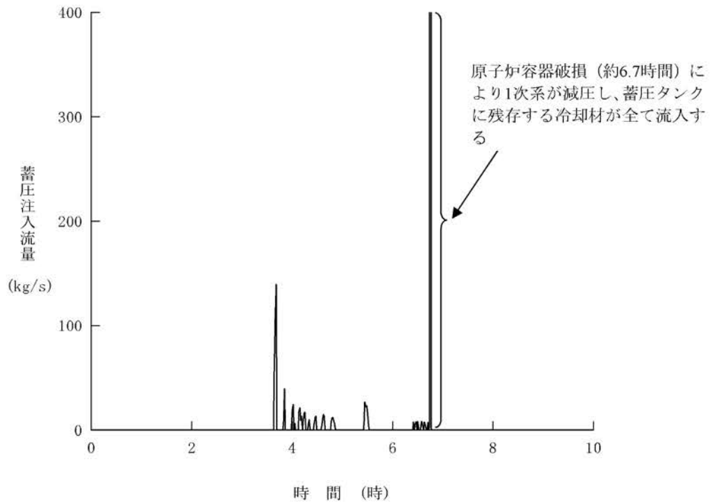
第1.15-423図 蓄圧注入流量の推移
