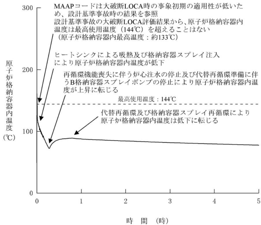
第1.15-314図 原子炉格納容器内温度の推移
