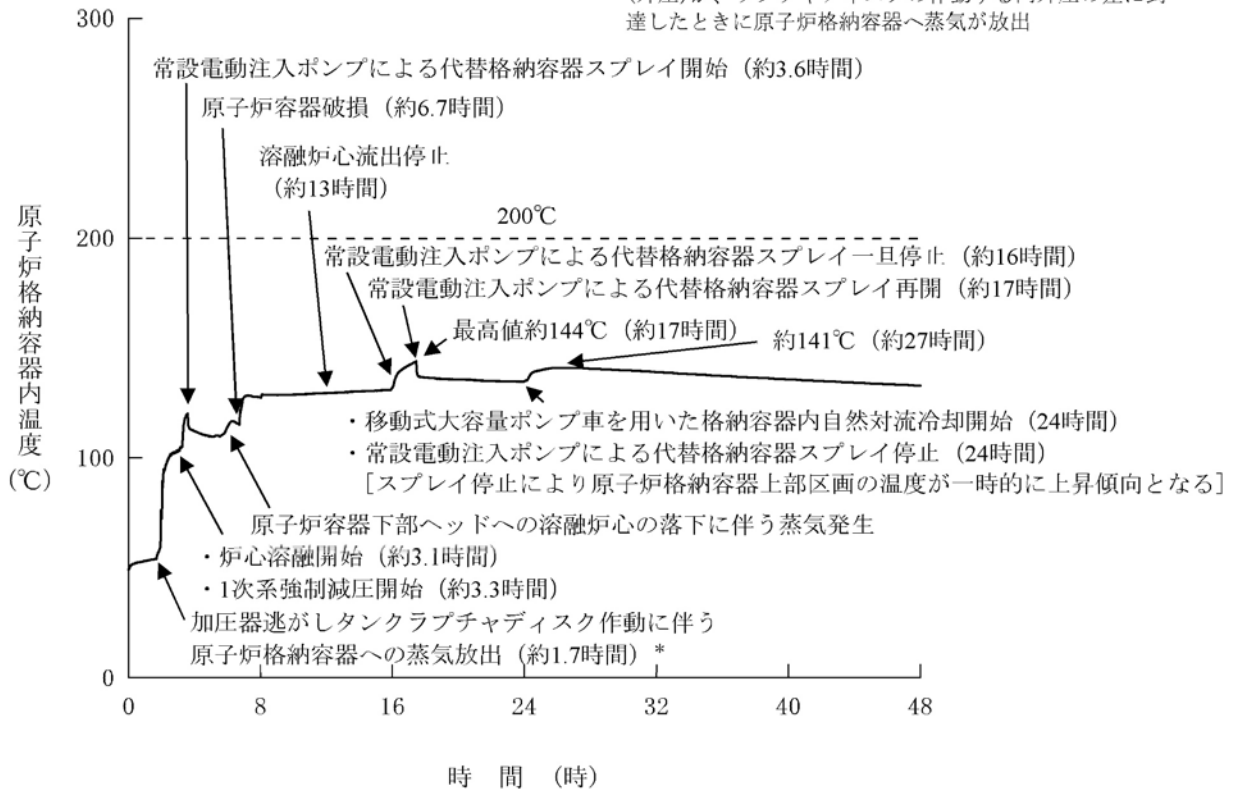
第1.15-413図 原子炉格納容器内温度の推移
