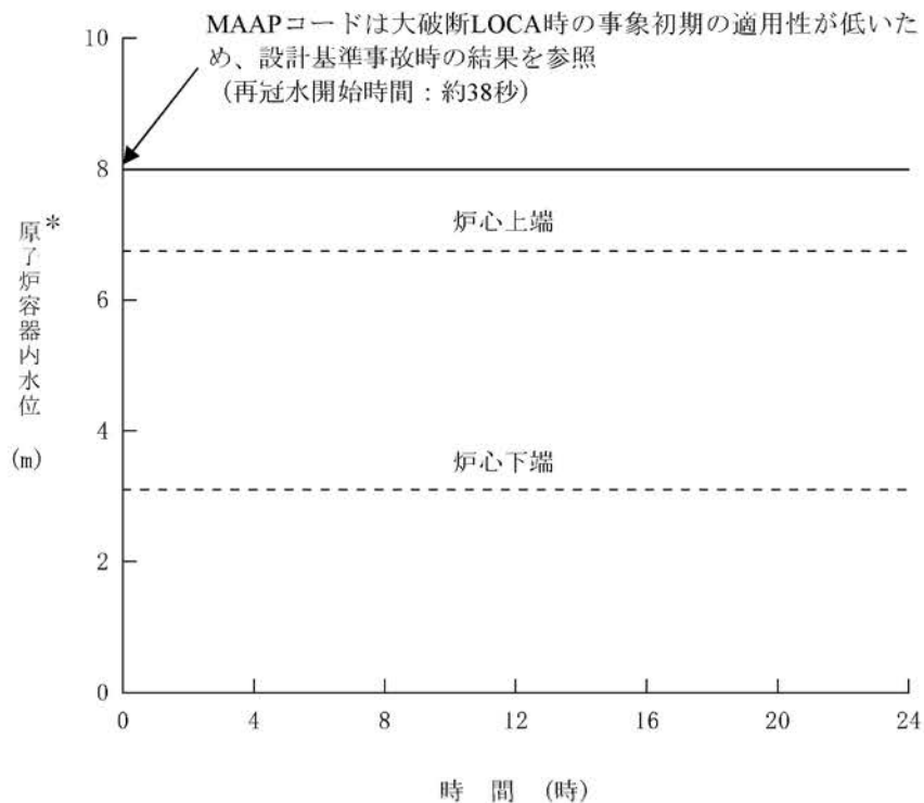
第1.15-215図 原子炉容器内水位の推移
