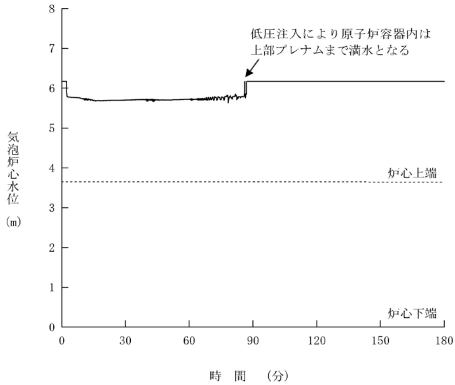
第1.15-279図 気泡炉心水位の推移 (2inch破断)
