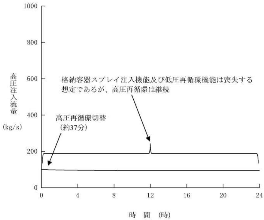
第1.15-213図 高圧注入流量の推移
