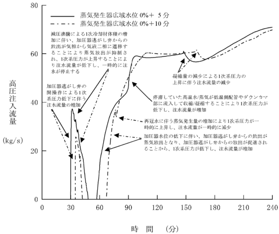
第1.15-165図 高圧注水流量の推移(開始が遅くなる場合)
