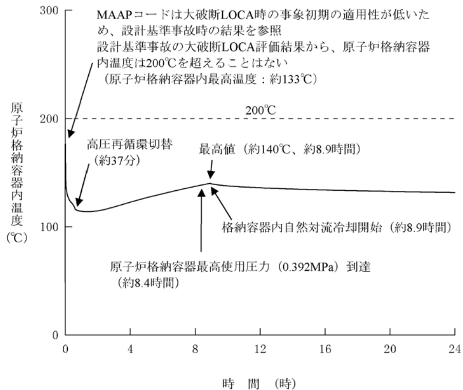
第1.15-221図 原子炉格納容器内温度の推移
