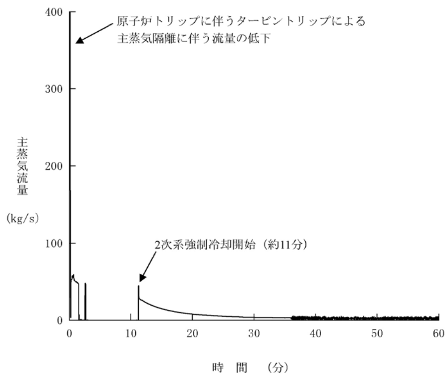
第1.15-264図 主蒸気流量の推移(6inch破断)
