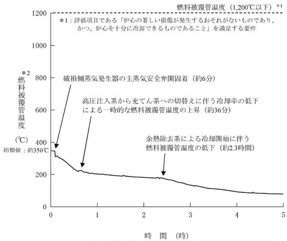
第1.15-342図 燃料被覆管温度の推移 (蒸気発生器伝熱管破損時に破損側蒸気発生器の隔離に失敗する事故)
