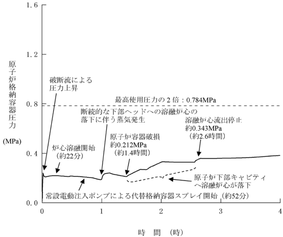
第1.15-387図 原子炉格納容器圧力の推移(～4時間)
