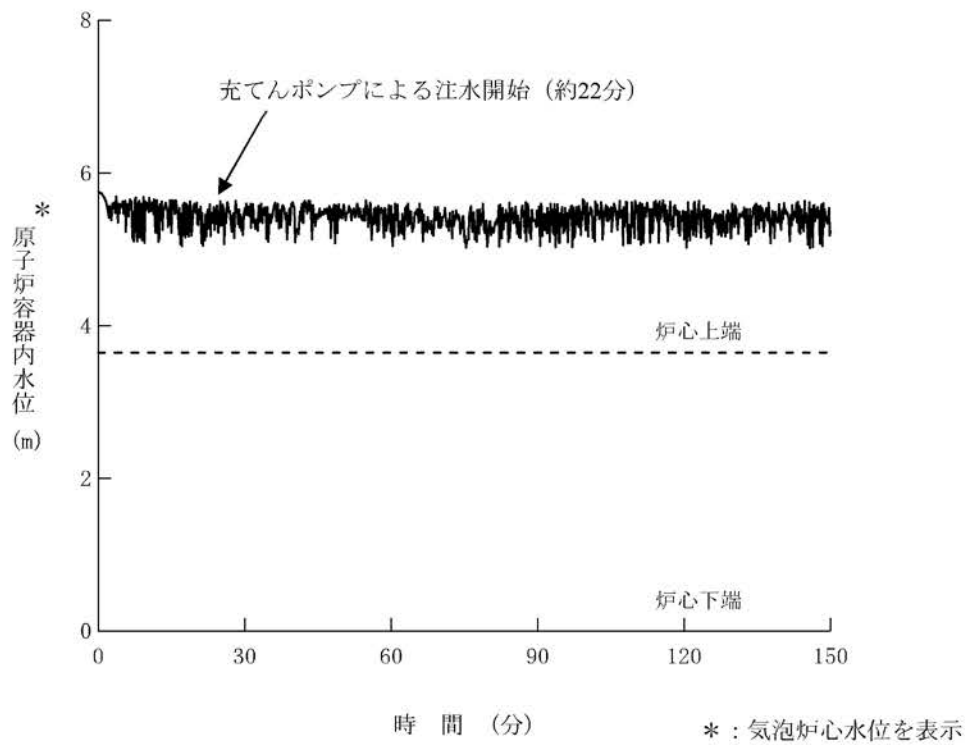
第1.15-373図 原子炉容器内水位の推移
