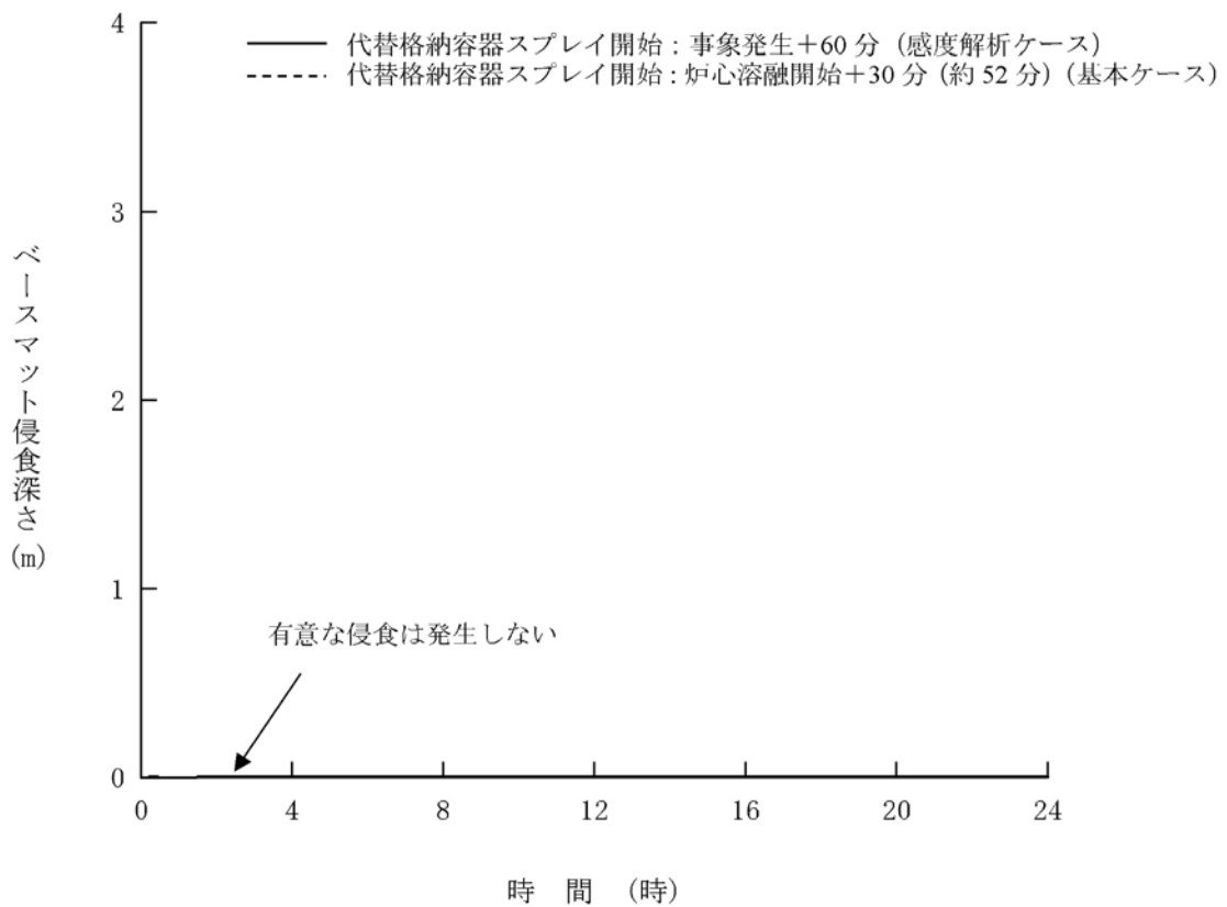
第1.15-448図 ベースマツト侵食深さの推移 (代替格納容器スプレイ操作時間余裕確認)
