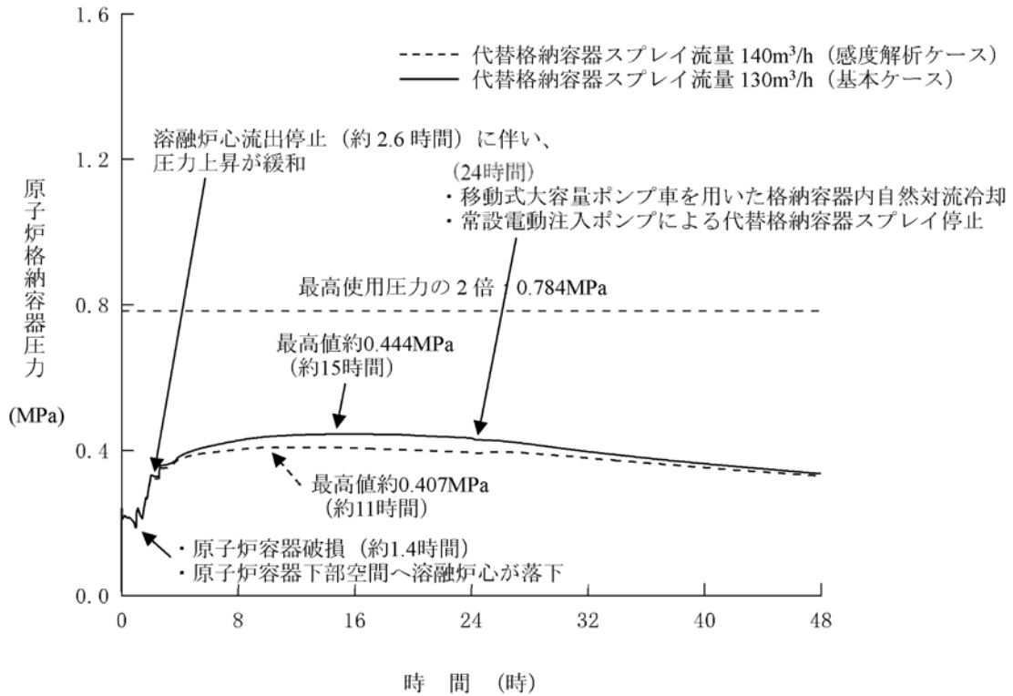
第1.15-400図 原子炉格納容器圧力の推移 (常設電動注入ポンプによる代替格納容器スプレイ流量の影響確認)
