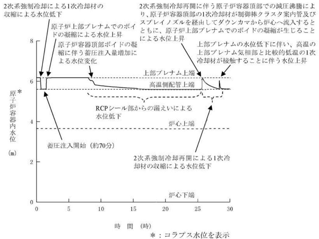
第1.15-197図 原子炉容器内水位の推移 (RCPシールLOCAが発生しない場合)
