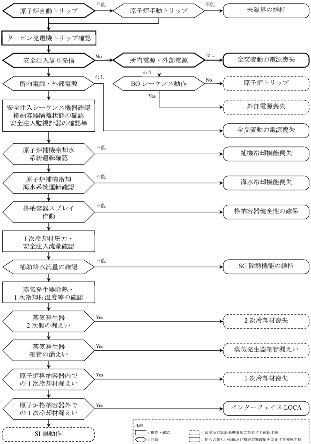
第1.15-408図 「雰囲気圧力・温度による静的負荷(格納容器過温破損)」の事象進展 (事象判別プロセス)
