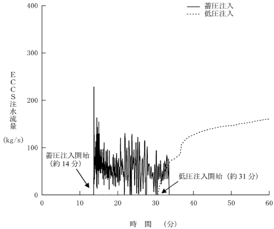
第1.15-267図 ECCS注水流量の推移(4inch破断)
