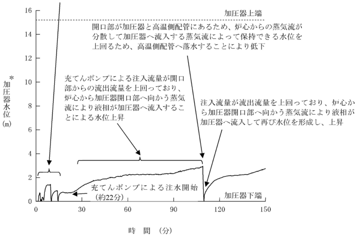
第1.15-375図 加圧器水位の推移
