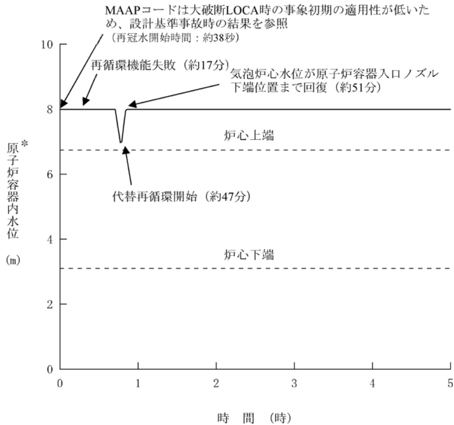
第1.15-309図 原子炉容器内水位の推移
