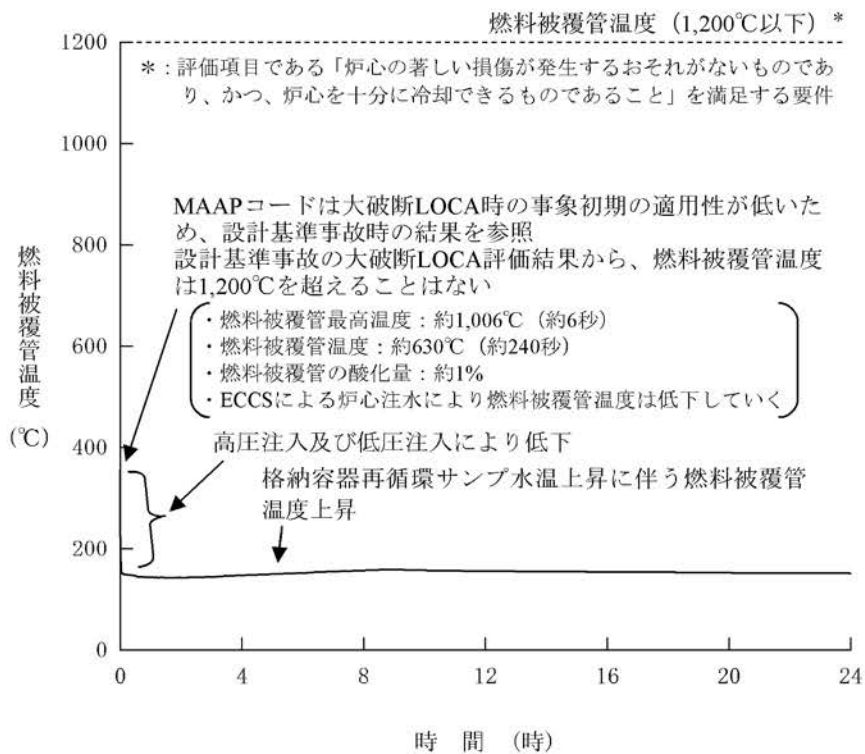
第1.15-216図 燃料被覆管温度の推移
