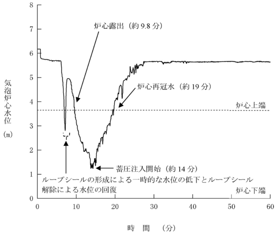
第1.15-269図 気泡炉心水位の推移(4inch破断)
