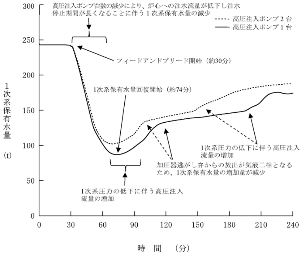
第1.15-154図 1次系保有水量の推移 (高圧注入ポンプ1台の場合)
