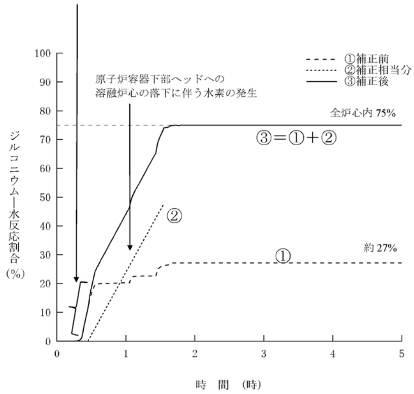
第1.15-431図 ジルコニウム-水反応割合の推移 (MAAPコード)
