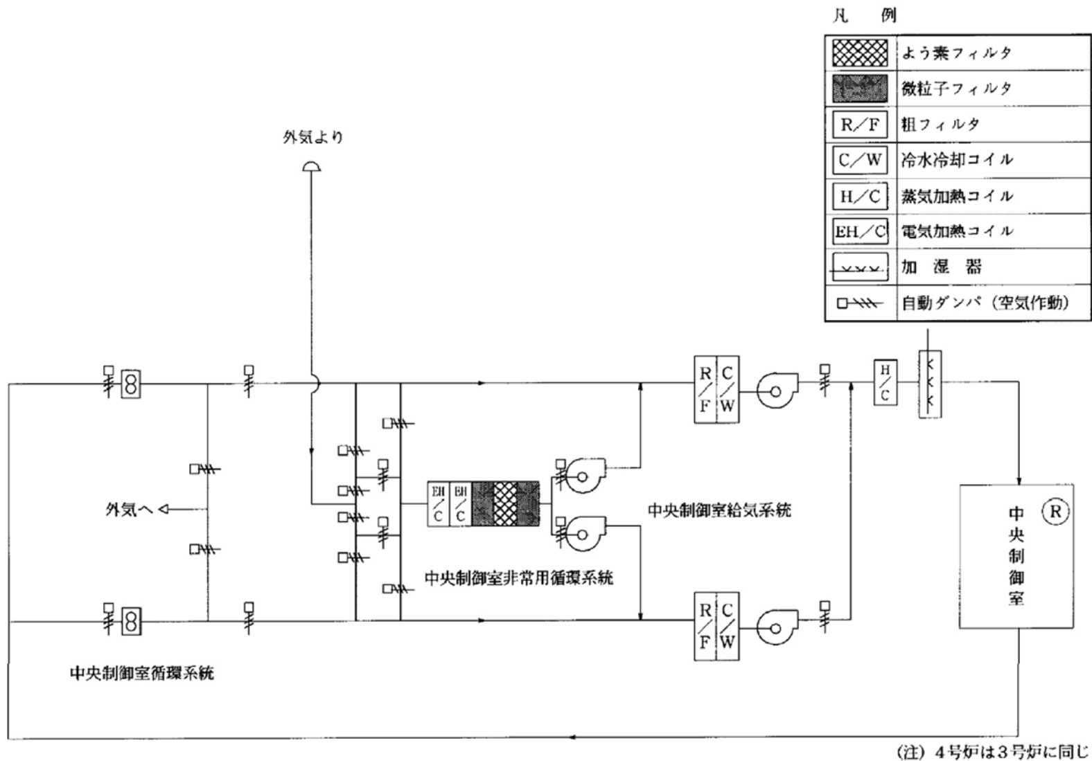
第1.12-25図 補助建屋換気空調設備系統説明図(中央制御室)
