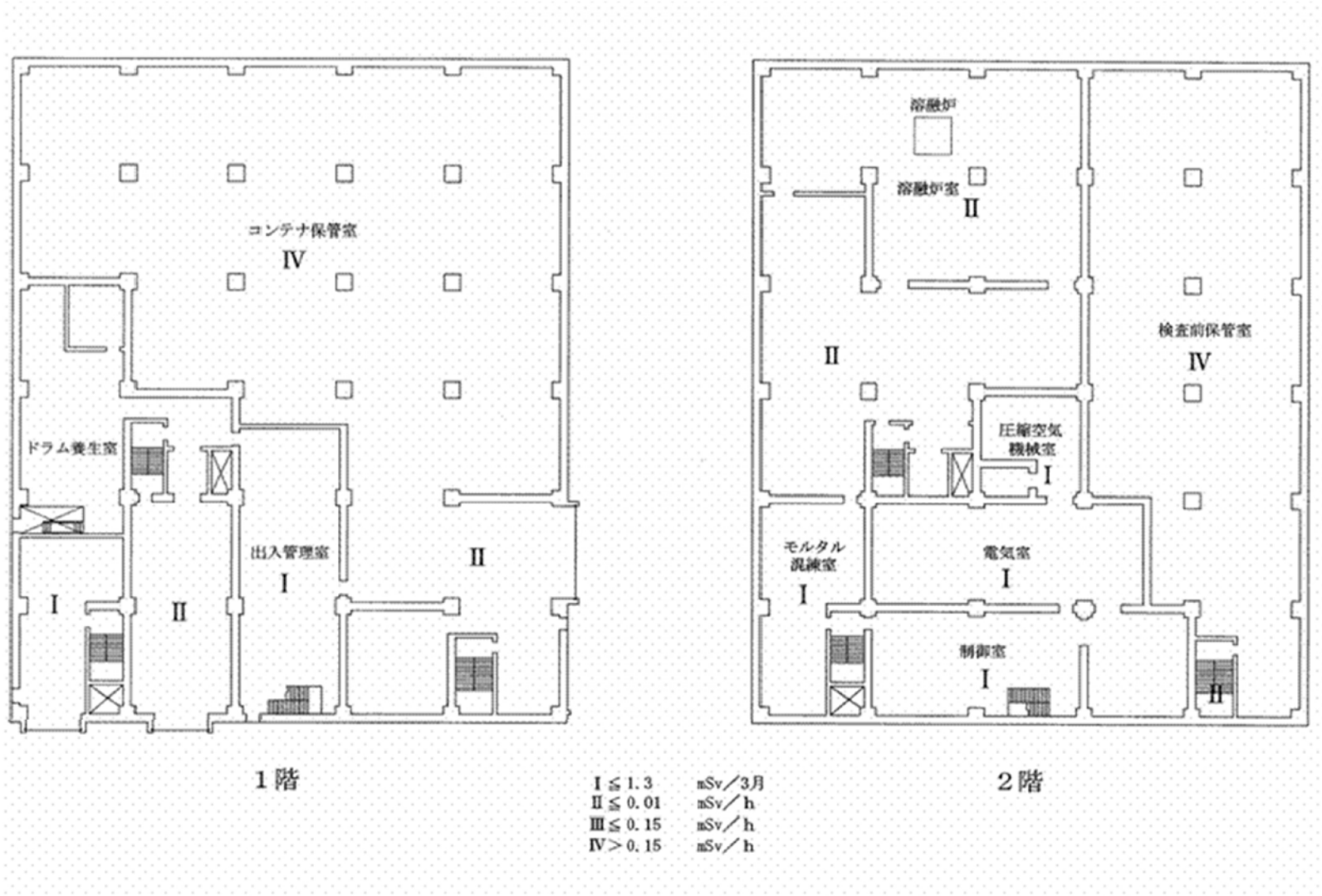
第1.12-17図 雑固体溶融処理建屋遮蔽設計区分概略図(1階及び2階)
