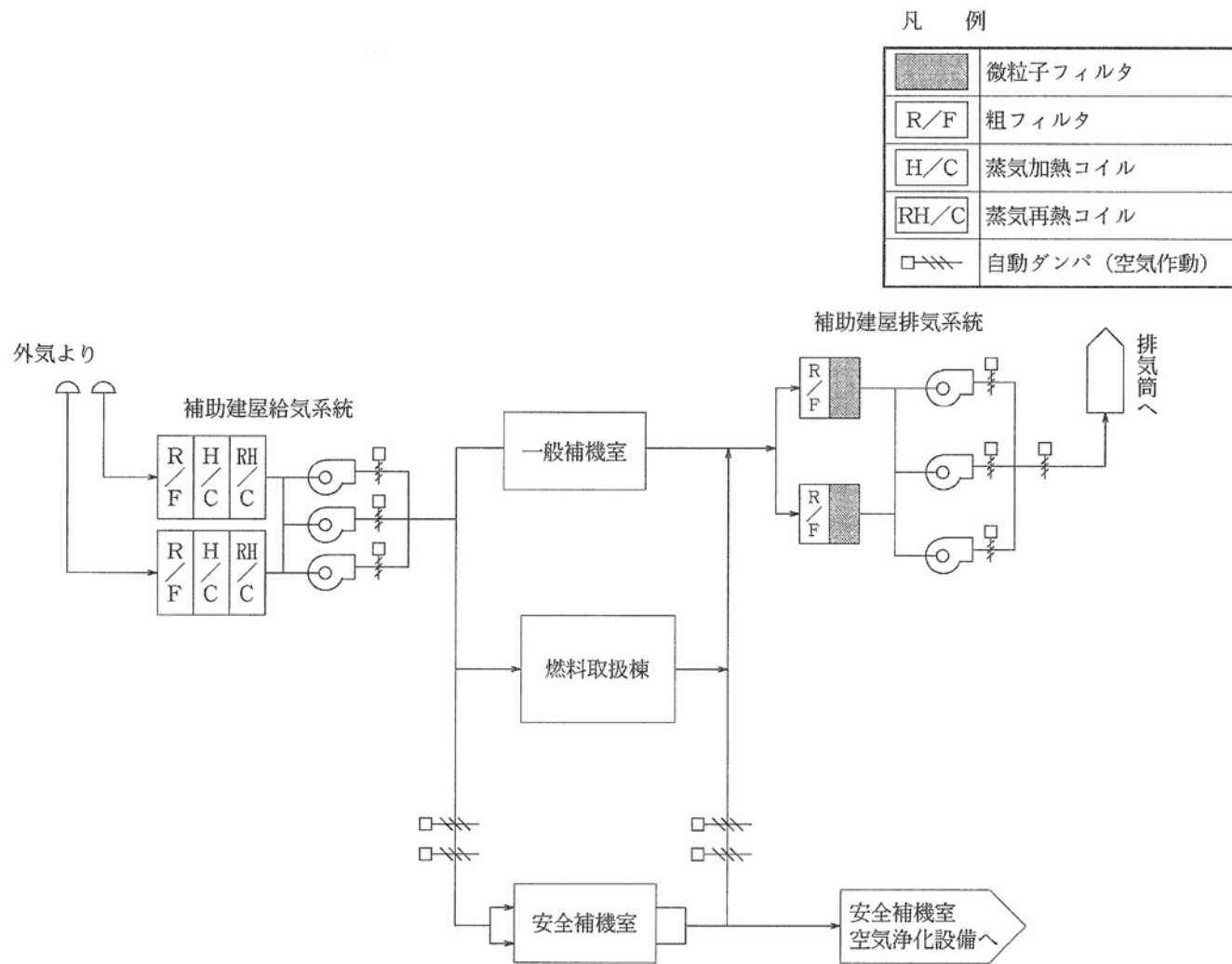
第1.12-21図 補助建屋換気空調設備系統説明図(一般補機室、燃料取扱棟及び安全補機室)(4号機)
