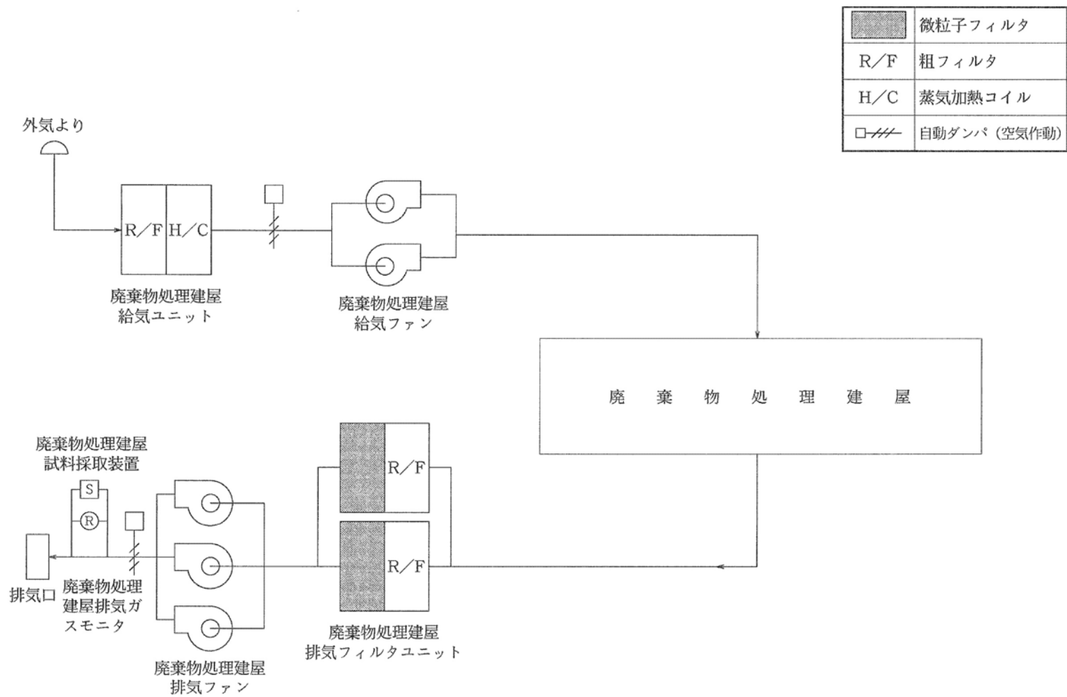
第1.12-26図 廃棄物処理建屋空調装置説明図(3、4号機共用)
