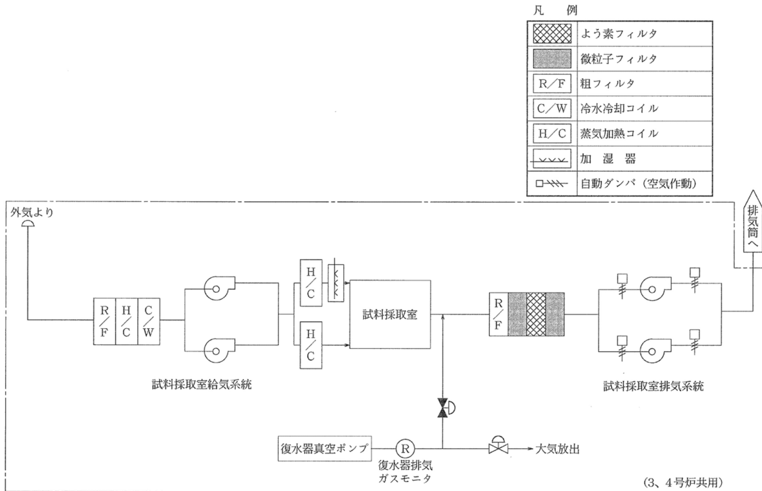
第1.12-23図 補助建屋換気空調設備系統説明図(試料採取室)
