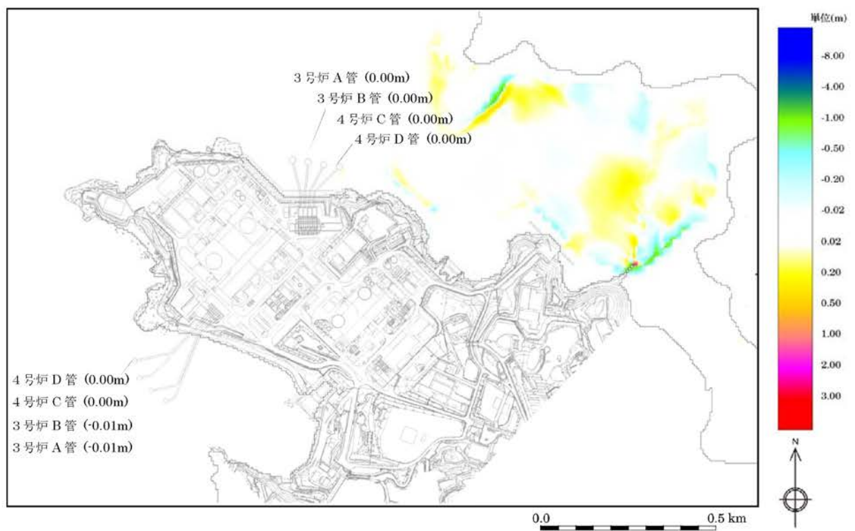
第1.2-13図(2) 砂移動による最終地形変化量（水位下降側）
