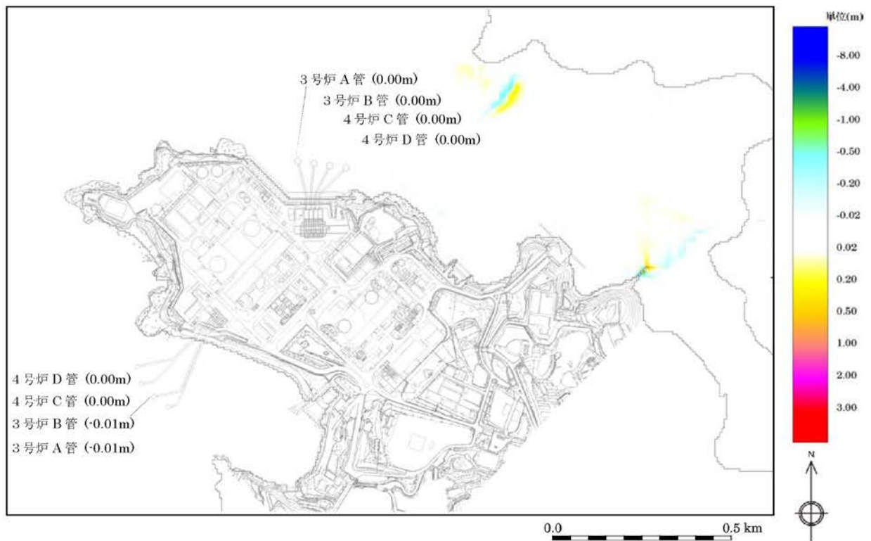
第1.2-13図(1) 砂移動による最終地形変化量（水位上昇側）
