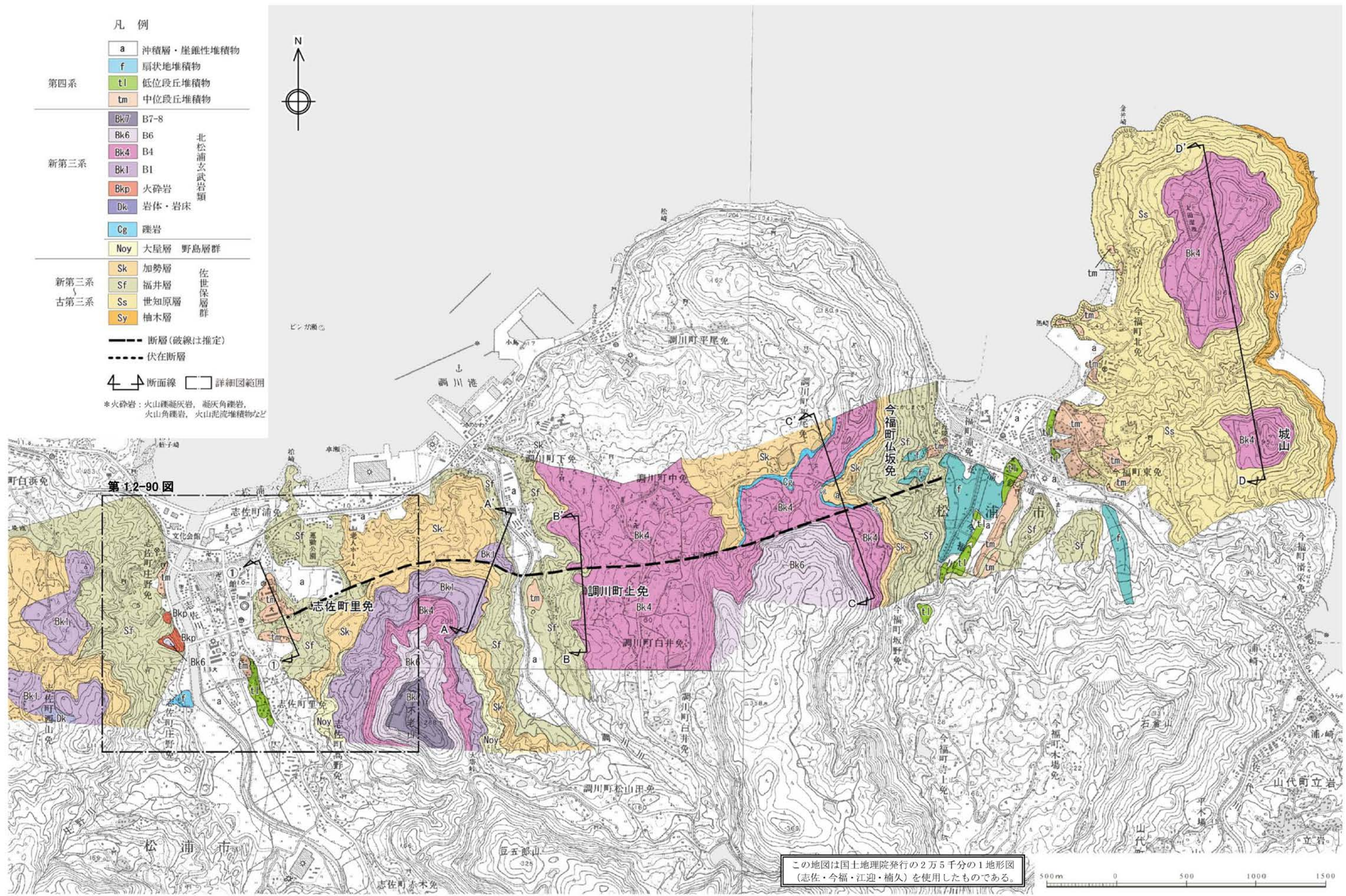
第1.2-88図 今福断層周辺の地質図
