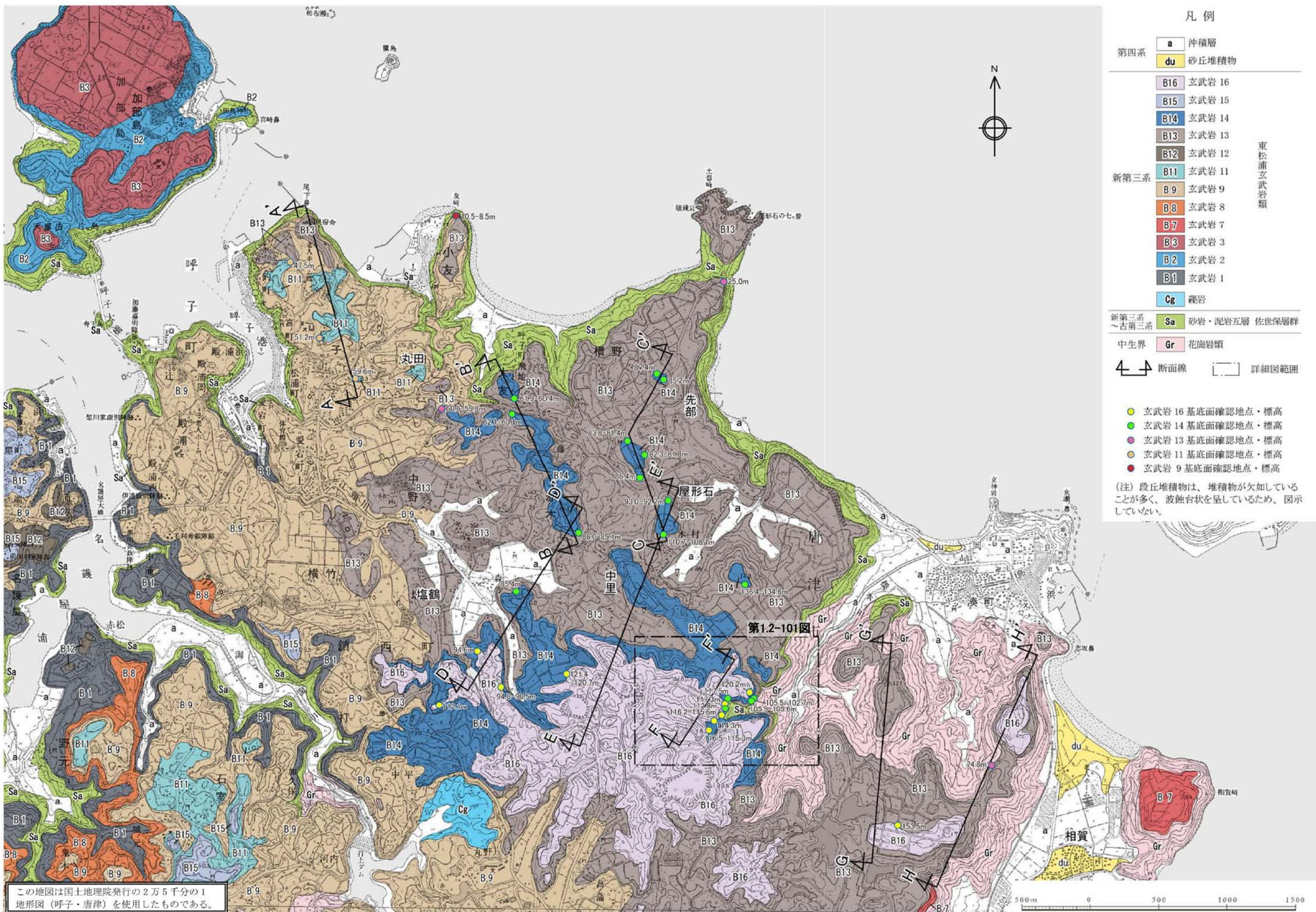
第1.2-99図 呼子北リニアメント・呼子南リニアメント周辺の地質図 1.2-494
