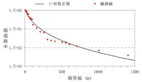
超過確率
