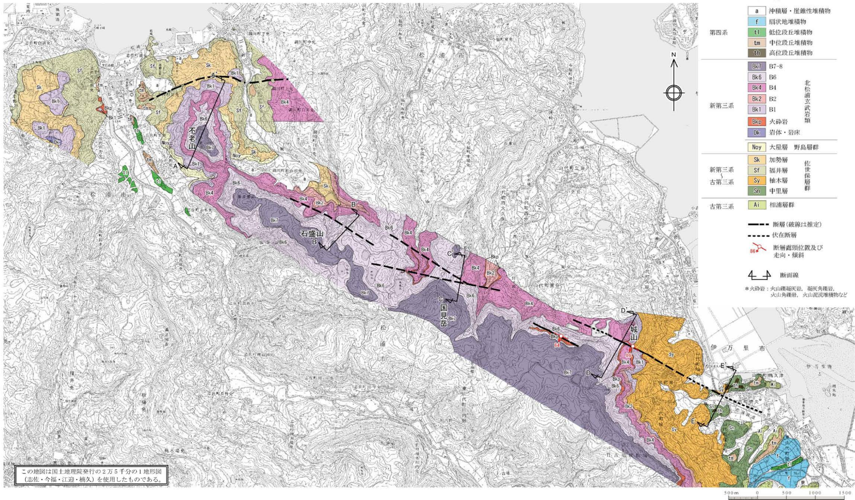
第1.2-81図 楠久断層周辺の地質図
