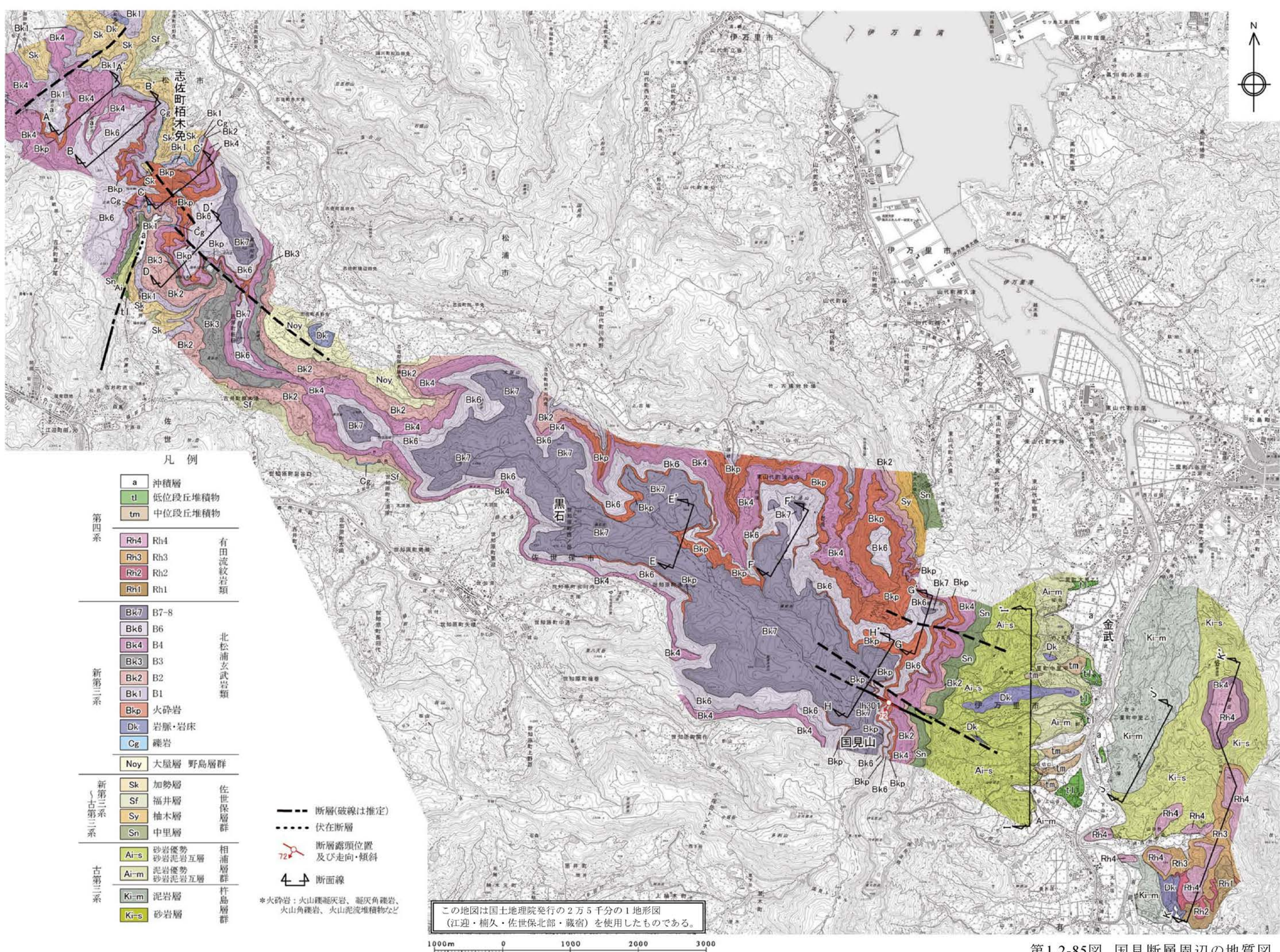
第1.2-85図 国見断層周辺の地質図 1.2-479
