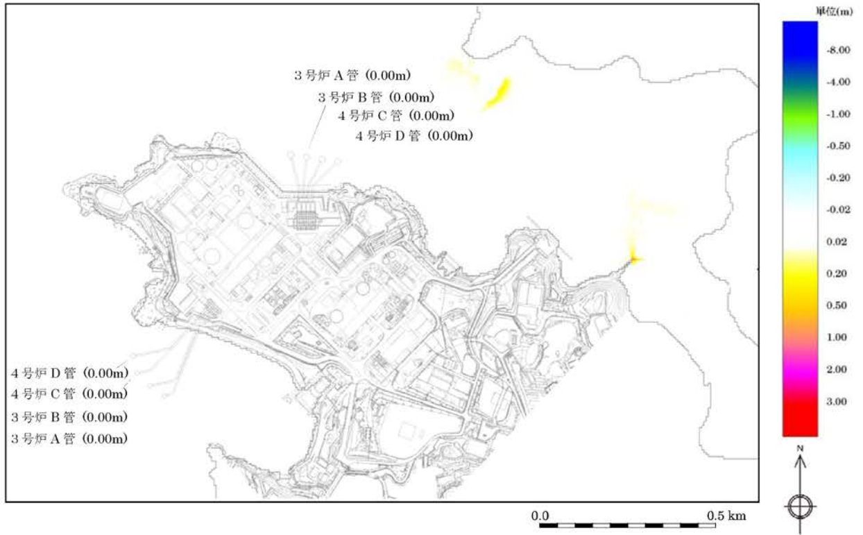
第1.2-13図(3) 砂移動による最大堆積厚（水位上昇側）
