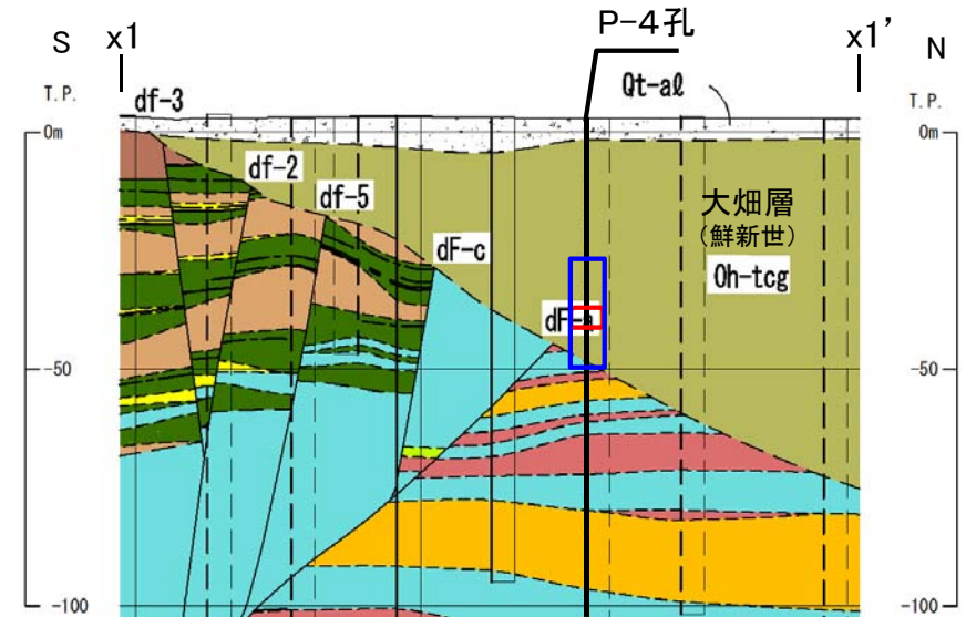
地質鉛直断面図(南北方向 x1-x1') 注) 凡例はP.3-27参照。
