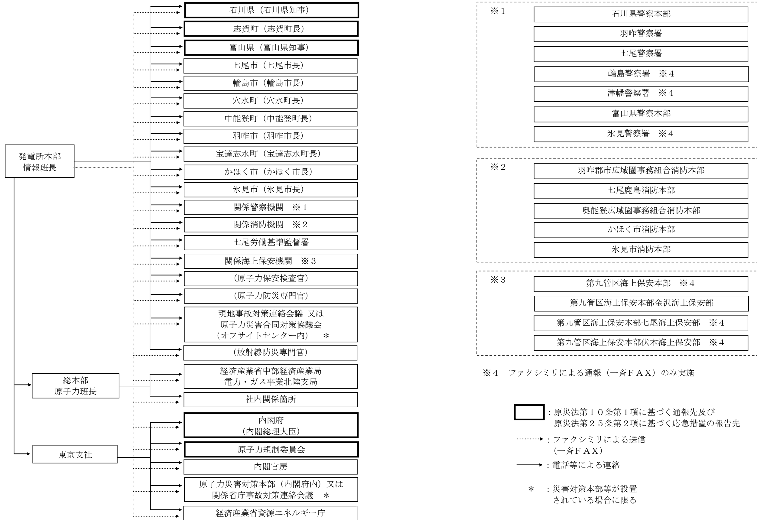
別図-4 原災法第10条第1項の通報（初回）後の連絡経路（1/2）
