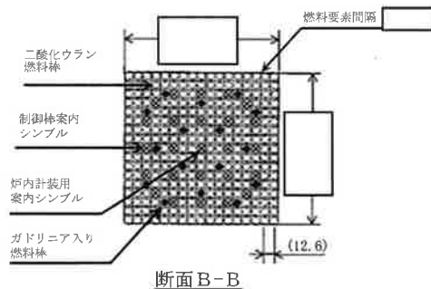
断面B-B (ガドリニア入り二酸化ウラン燃料要素配置)
