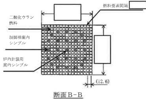
断面B-B (二酸化ウラン燃料要素配置)
