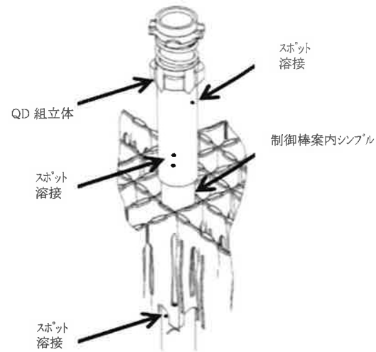
上部支持格子及び制御棒案内 シンプル上部スリーブと制御 棒案内シンプルの接合 (b)
