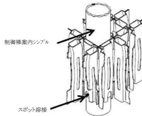
中間部支持格子と制御棒 案内シンプルの接合 (c)
