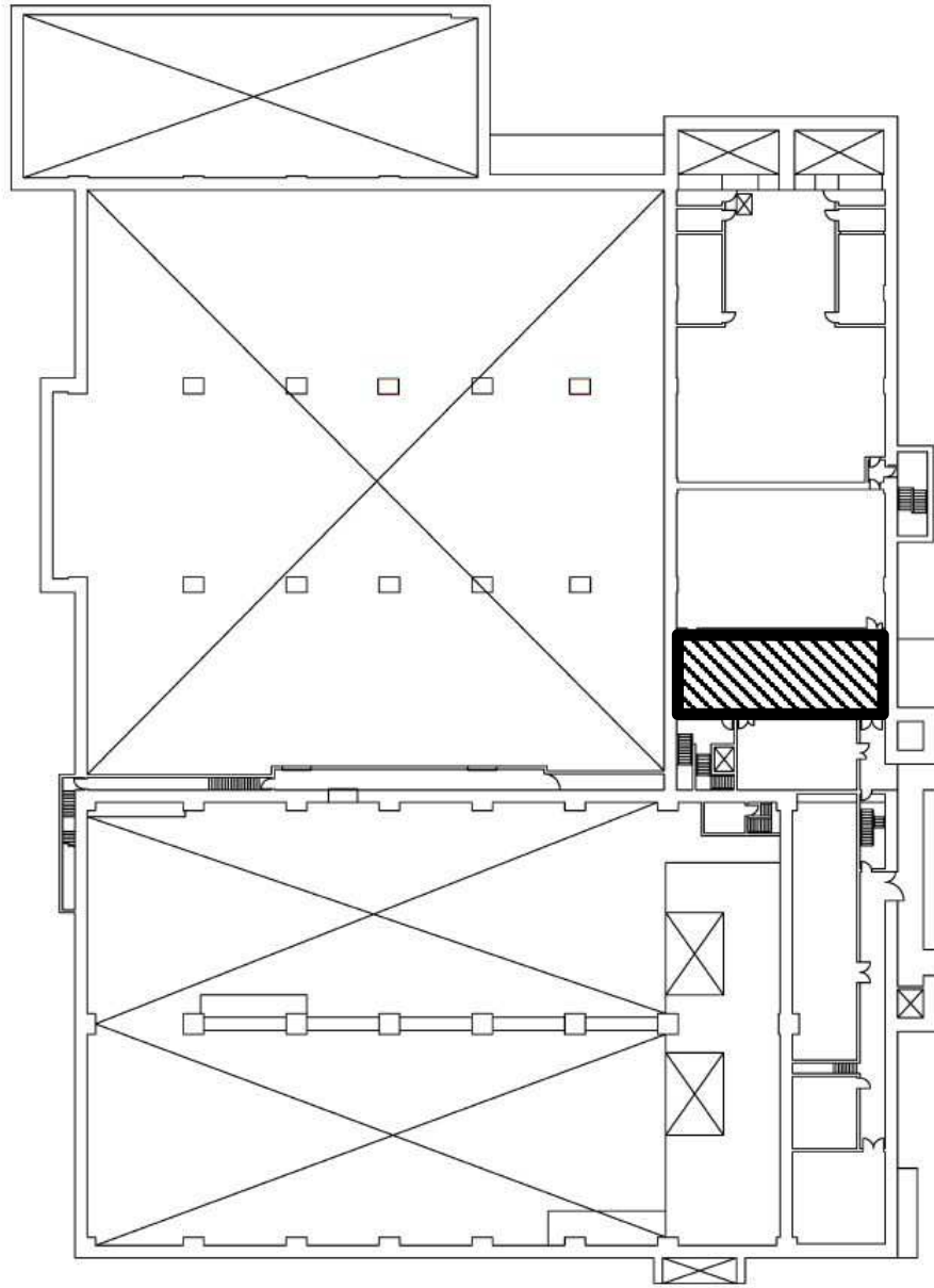
第10-12図 使用済燃料の受入れ施設及び貯蔵施設の制御室 可搬型代替照明 配置概要図
