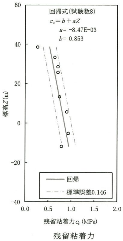
第 4.5-9 図(7) 強度特性 (三軸圧縮試験による強度定数と標高の関係)
