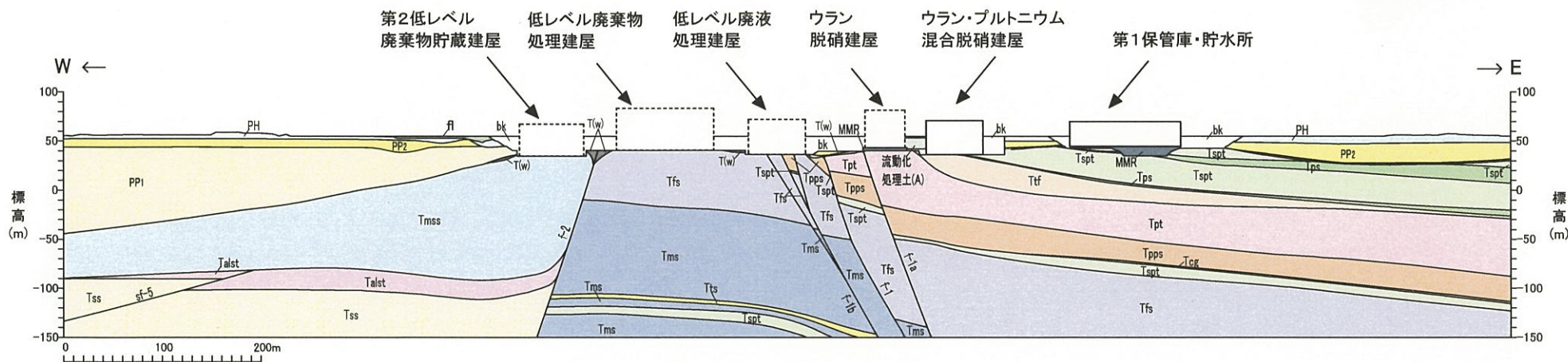
第4.5-6図(18) 耐震重要施設等及び常設重大事故等対処施設設置位置付近の岩盤分類図 (鉛直断面図：N測線)
