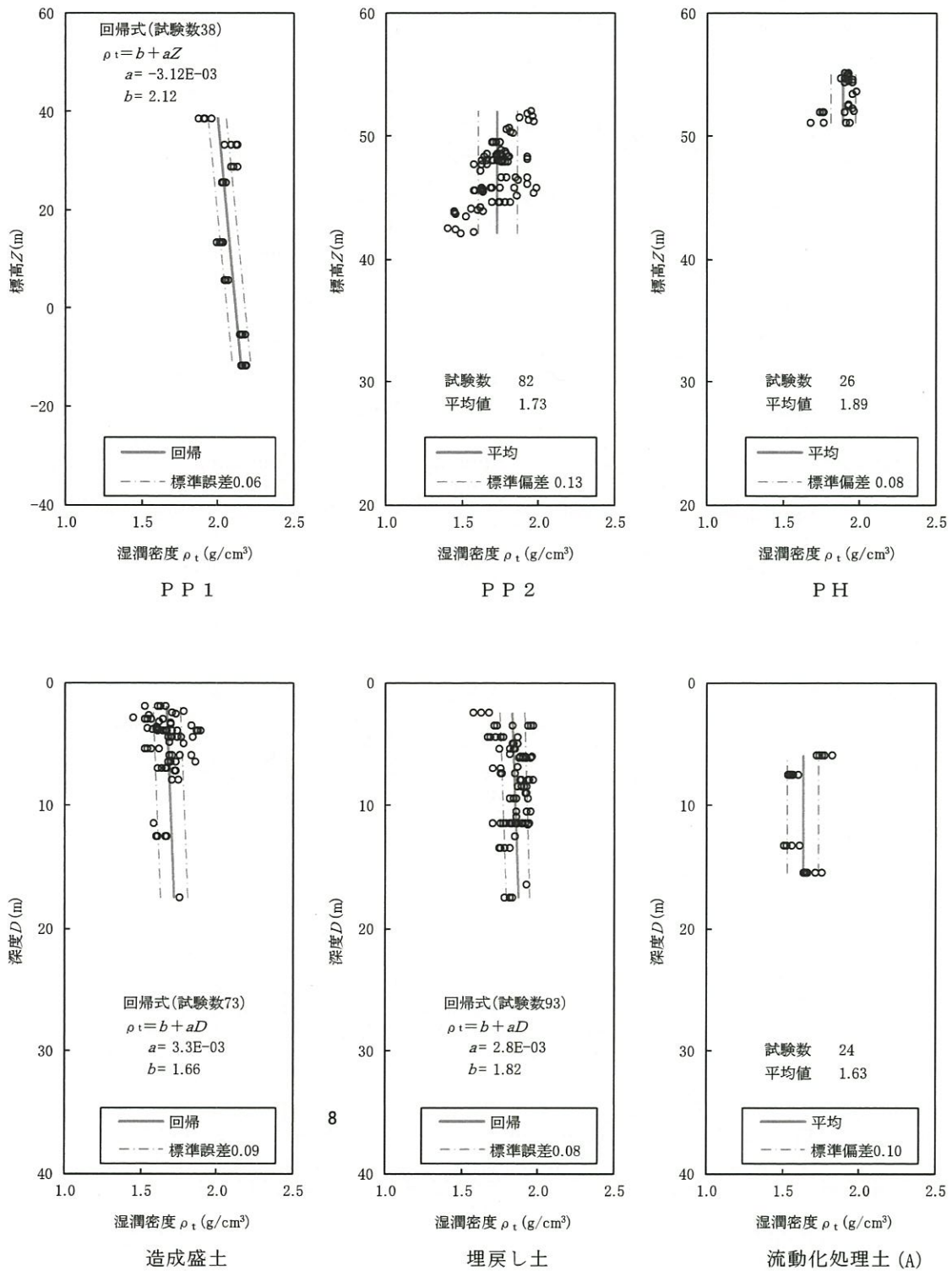
第 4.5-7 図(3) 湿潤密度と標高または地表からの深度の関係
