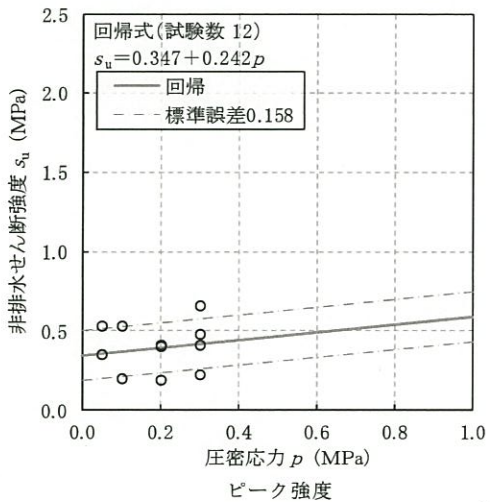
第 4.5-9 図(6) 強度特性 (非排水せん断強度と圧密応力の関係)
