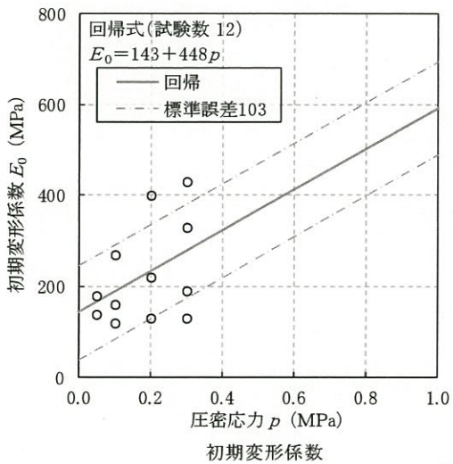
第 4.5-10 図(6) 静的変形特性 (初期変形係数及びポアソン比と圧密応力の関係)
