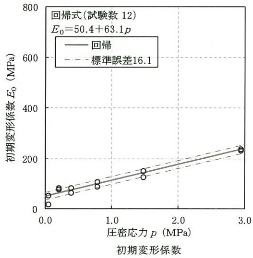
第 4.5-10 図(4) 静的変形特性 (初期変形係数及びポアソン比と圧密応力の関係)
