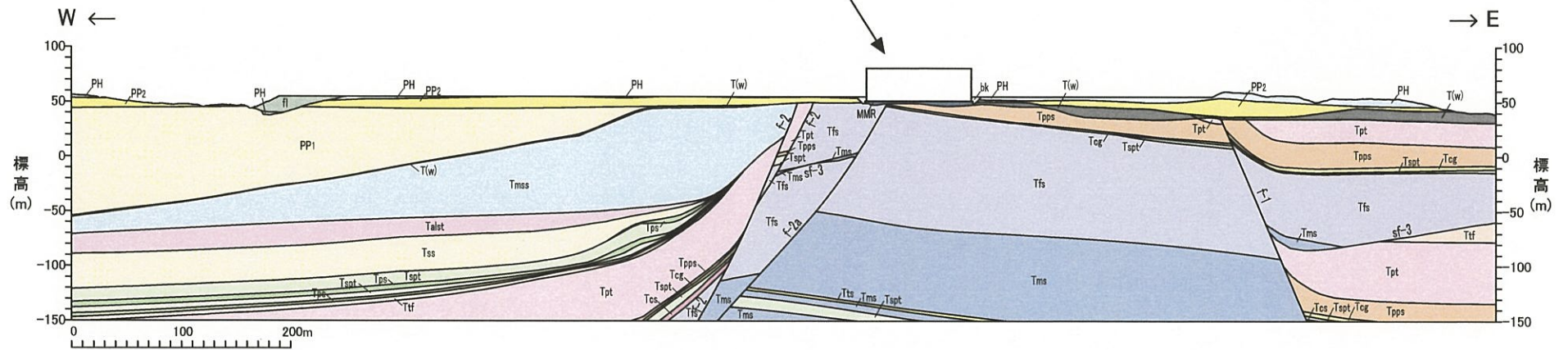
第4.5-6図(10) 耐震重要施設等及び常設重大事故等対処施設設置位置付近の岩盤分類図 (鉛直断面図：G2測線)
