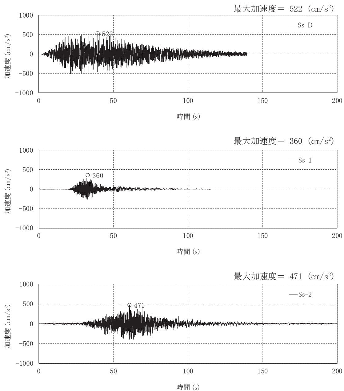
図 3-13 入力地震動の加速度時刻歴波形(鉛直方向, Ss, 基礎底面位置)
