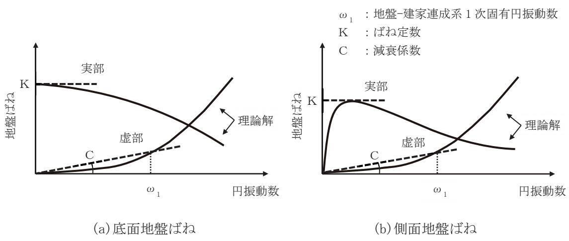
図 4-4 地盤ばね定数及び減衰係数と理論解との関係
