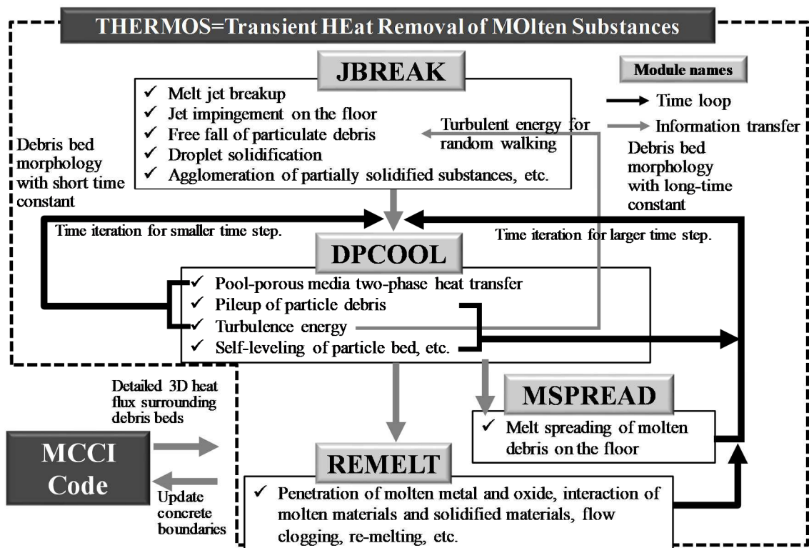
図1 多次元の熔融デブリ及びデブリベッドの形態変化及び冷却性解析コードシステム THERMOS の概要
