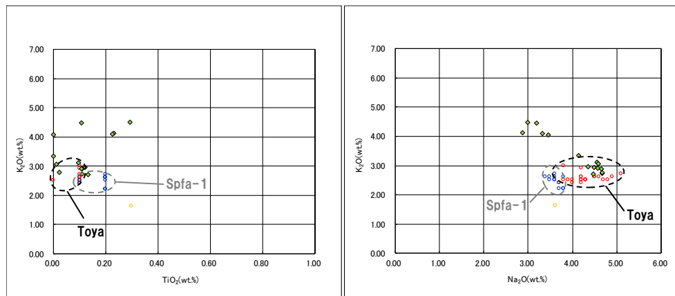
SKB-d' 火山ガラスのK 2 O-TiO 2 図(左図), K 2 O-Na 2 O図(右図)
