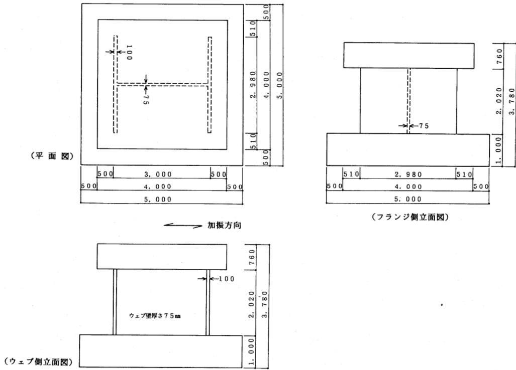
(a) 試験体形状
