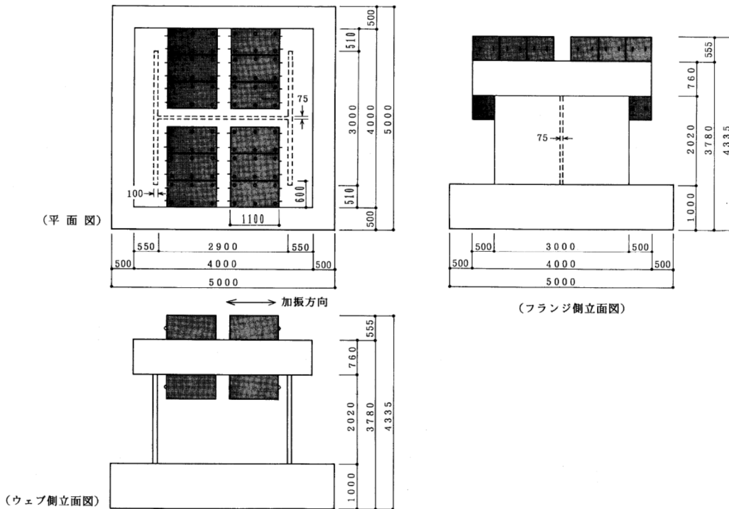
(b) 重鐘付加図
