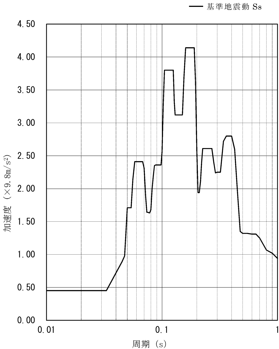
第 4-1 図(2/2) 基準地震動 Ss (基礎 EL.-10.10m 減衰定数 1.0% 鉛直方向 包絡)
