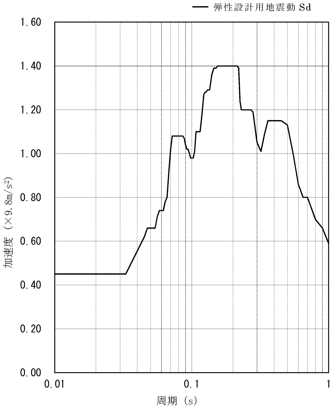
第 5-2 図(1/2) 弹性設計用地震動 Sd (基礎 EL. - 10.10m 減衰定数 4.0% 水平方向 包絡)
