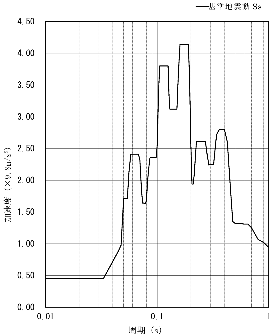
第 5-1 図(2/2) 基準地震動 Ss (基礎 EL. - 10.10m 減衰定数 1.0% 鉛直方向 包絡)
