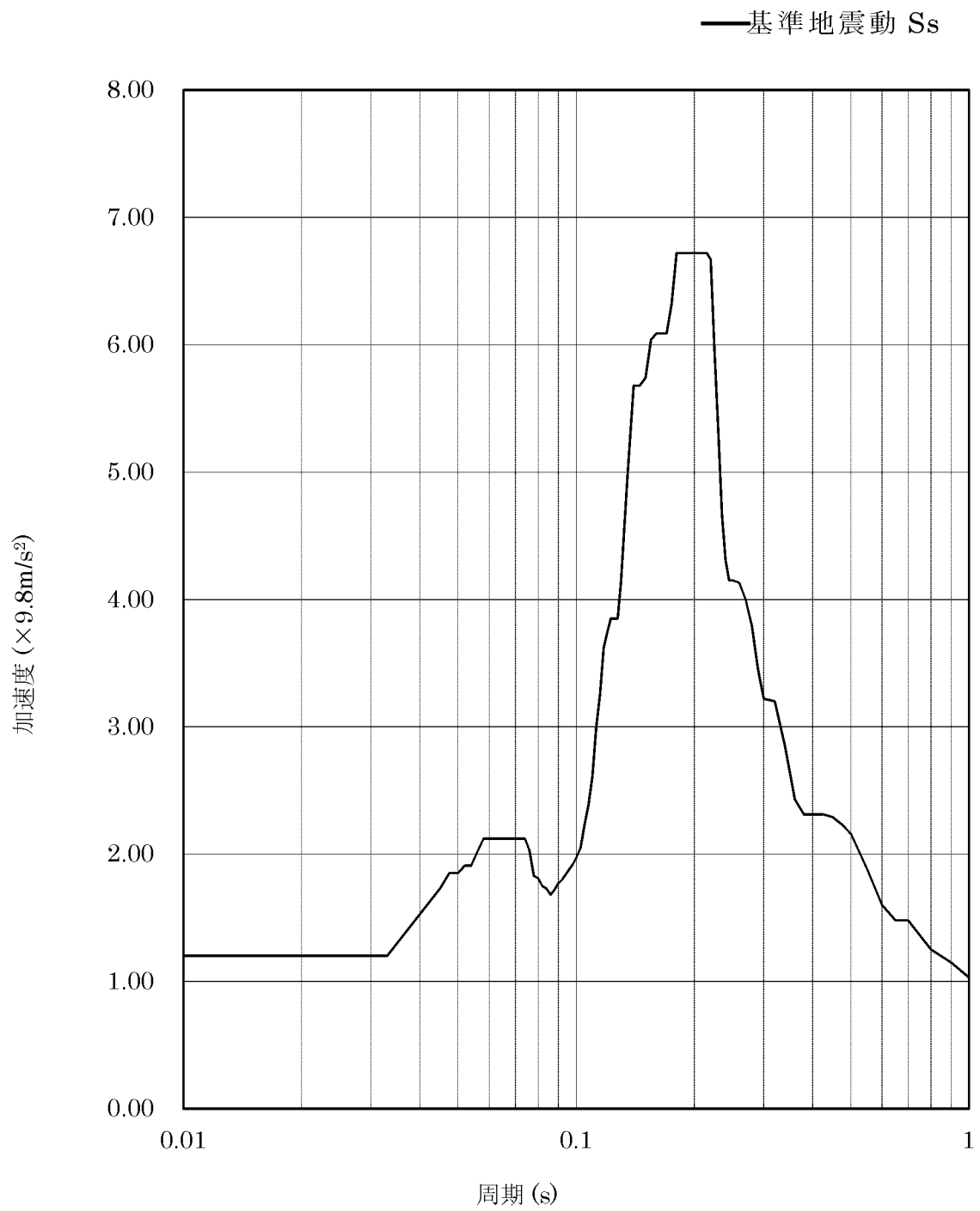
第 5-1 図 (1/2) 基準地震動 ( S_s ) (原子炉補助建屋EL.3.7m 減衰定数4.0% 水平方向 包絡)
