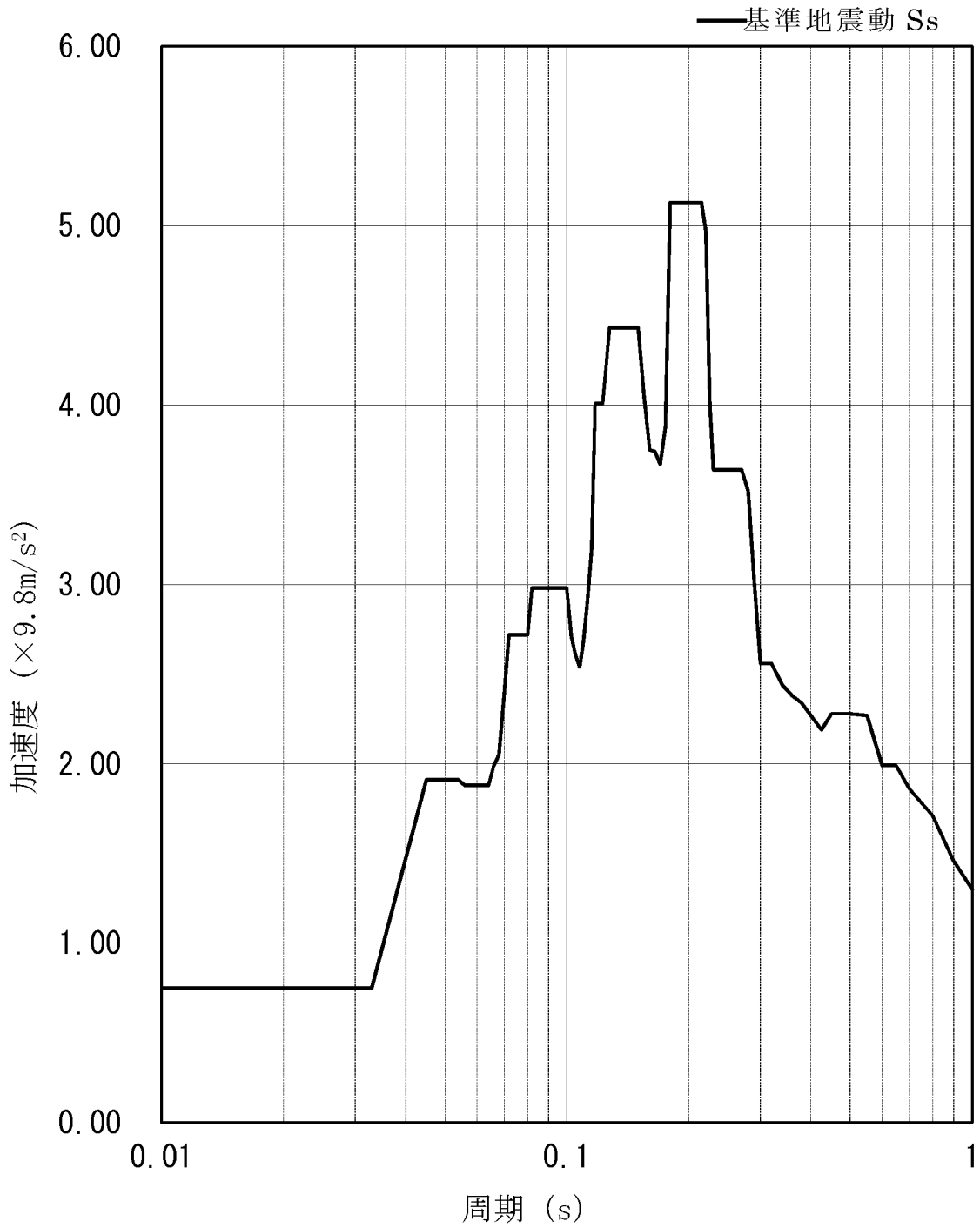
第 4-1 図(1/2) 基準地震動 Ss (基礎 EL. - 10.10m 減衰定数 1.0% 水平方向 包絡)
