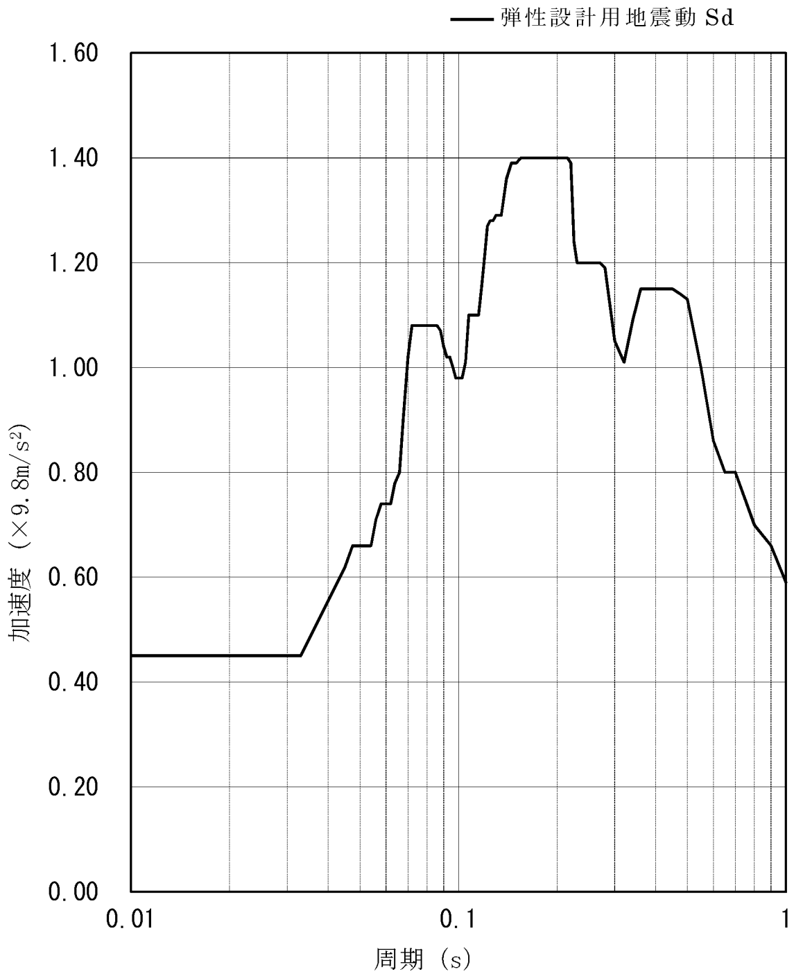
第 4-2 図(1/2) 弾性設計用地震動 Sd (基礎 EL. - 10.10m 減衰定数 4.0% 水平方向 包絡)
