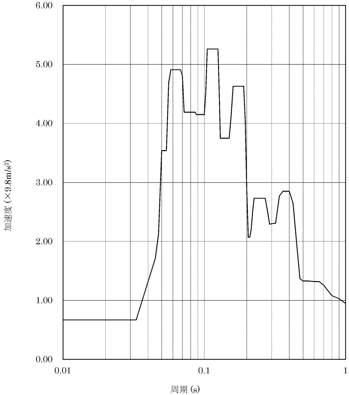
第 5-1 図 (2/2) 基準地震動 (Ss) (原子炉補助建屋EL. 3.7m 減衰定数1.0% 鉛直方向 包絡)
