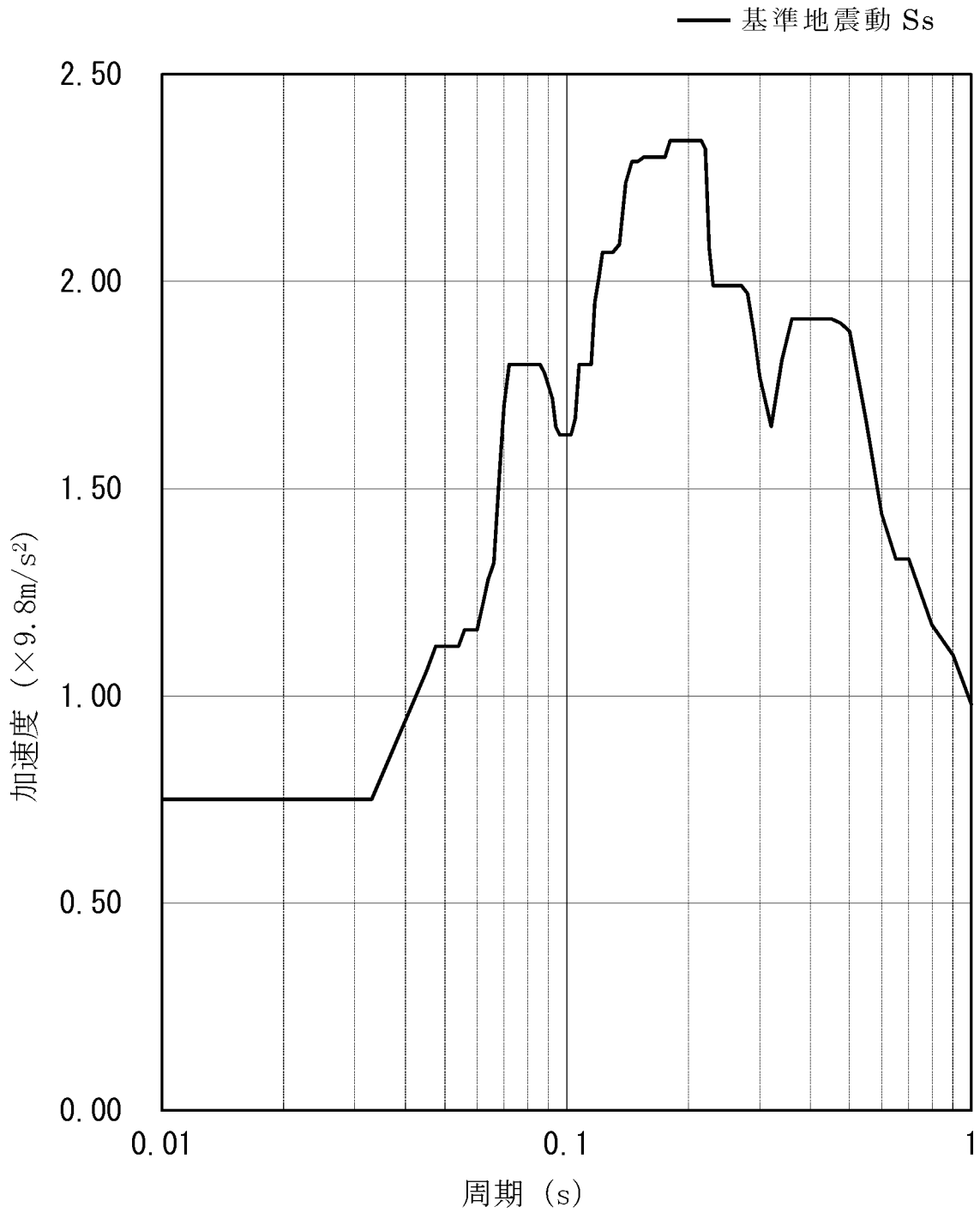
第 4-1 図(1/2) 基準地震動 Ss (基礎 EL. - 10.10m 減衰定数 4.0% 水平方向 包絡)
