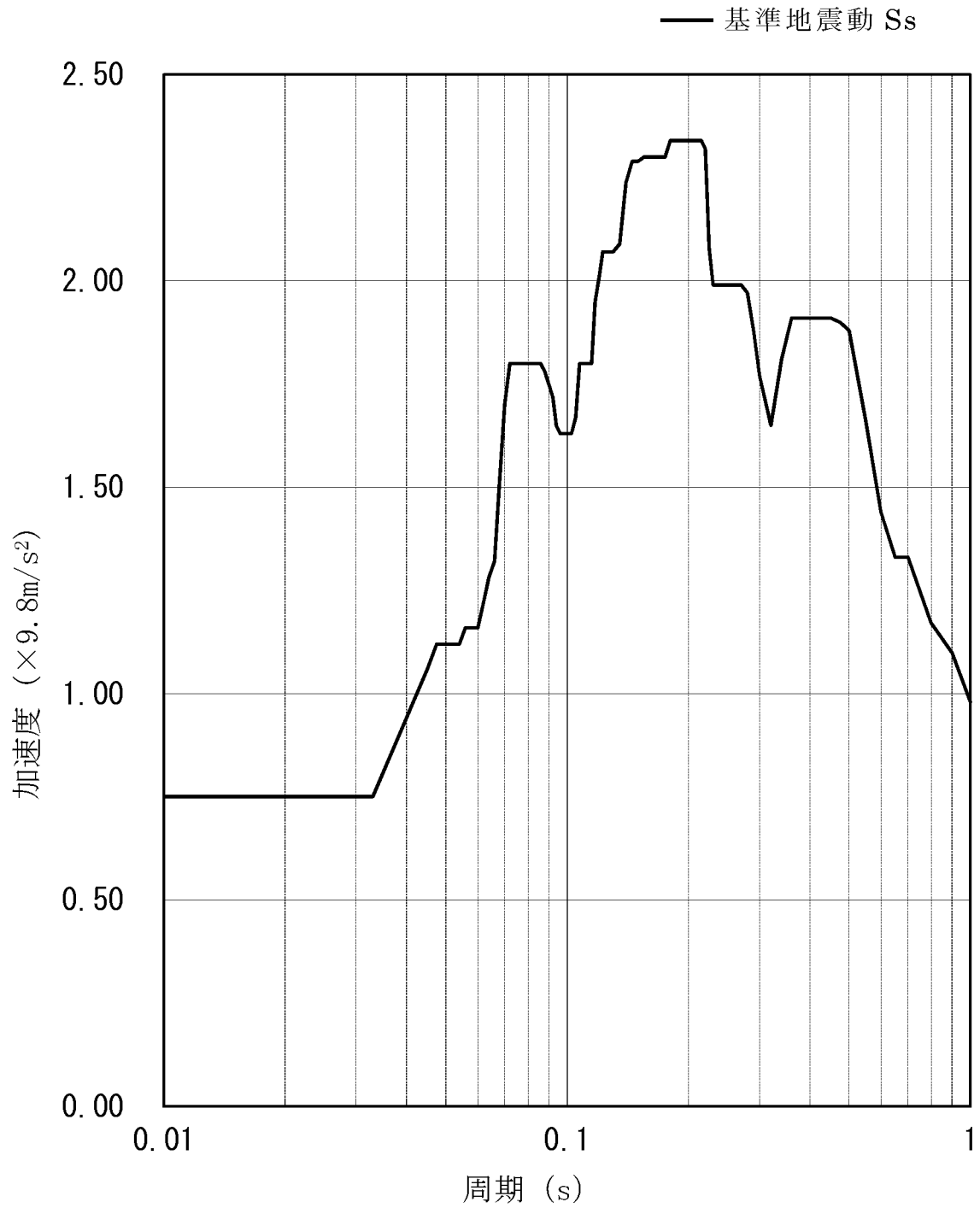
第 5-1 図(1/2) 基準地震動 Ss (基礎 EL. - 10.10m 減衰定数 4.0% 水平方向 包絡)
