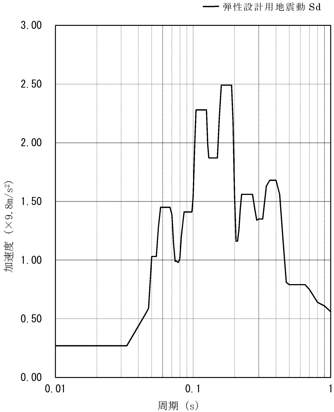
第 5-2 図(2/2) 弹性設計用地震動 Sd (基礎 EL. - 10.10m 減衰定数 1.0% 鉛直方向 包絡)
