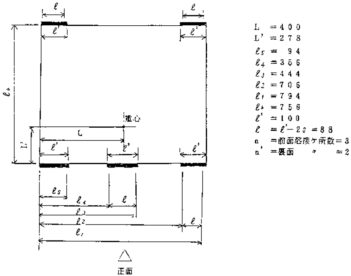
第 5-2 図 溶接長
