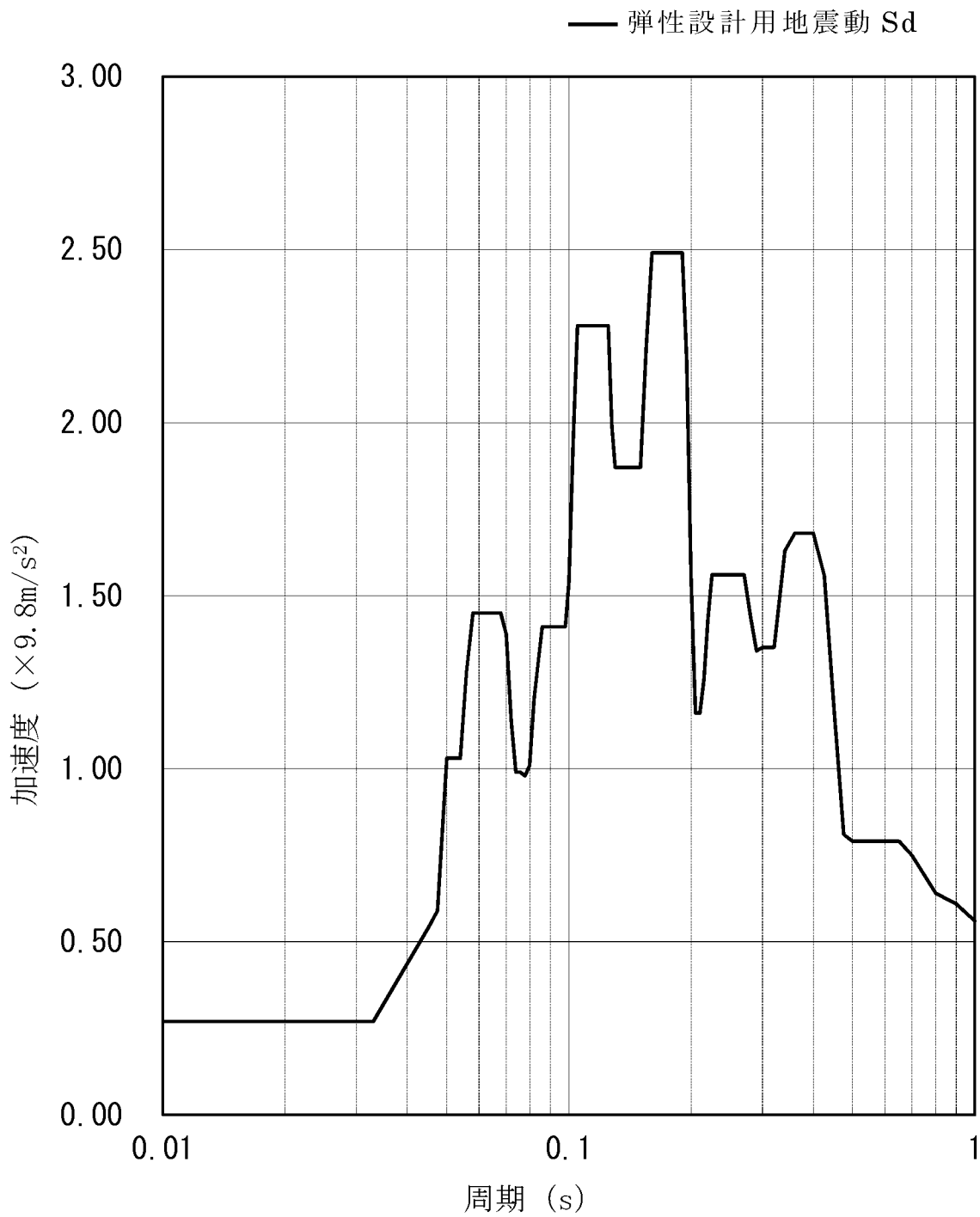
第 4-2 図(2/2) 弾性設計用地震動 Sd (基礎 EL. - 10.10m 減衰定数 1.0% 鉛直方向 包絡)
