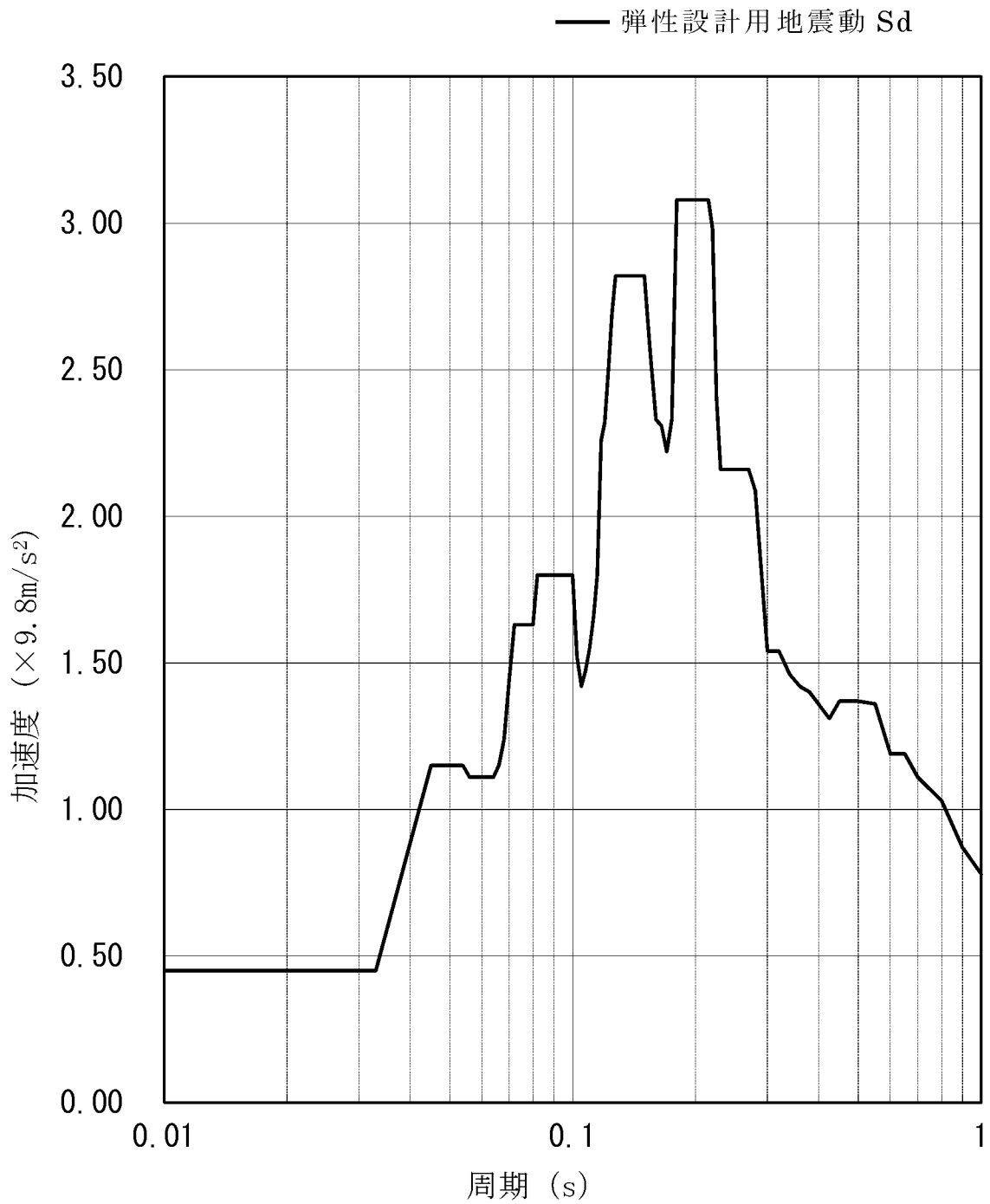
第 4-2 図(1/2) 弾性設計用地震動 Sd (基礎 EL. - 10.10m 減衰定数 1.0% 水平方向 包絡)
