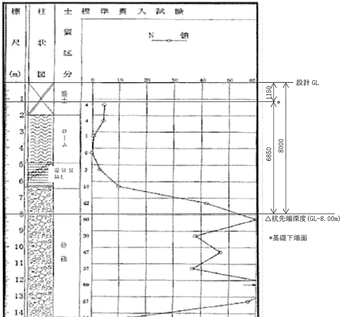
添説建 2-V.1.9-3 図 ボーリング柱状図 (②地点)
