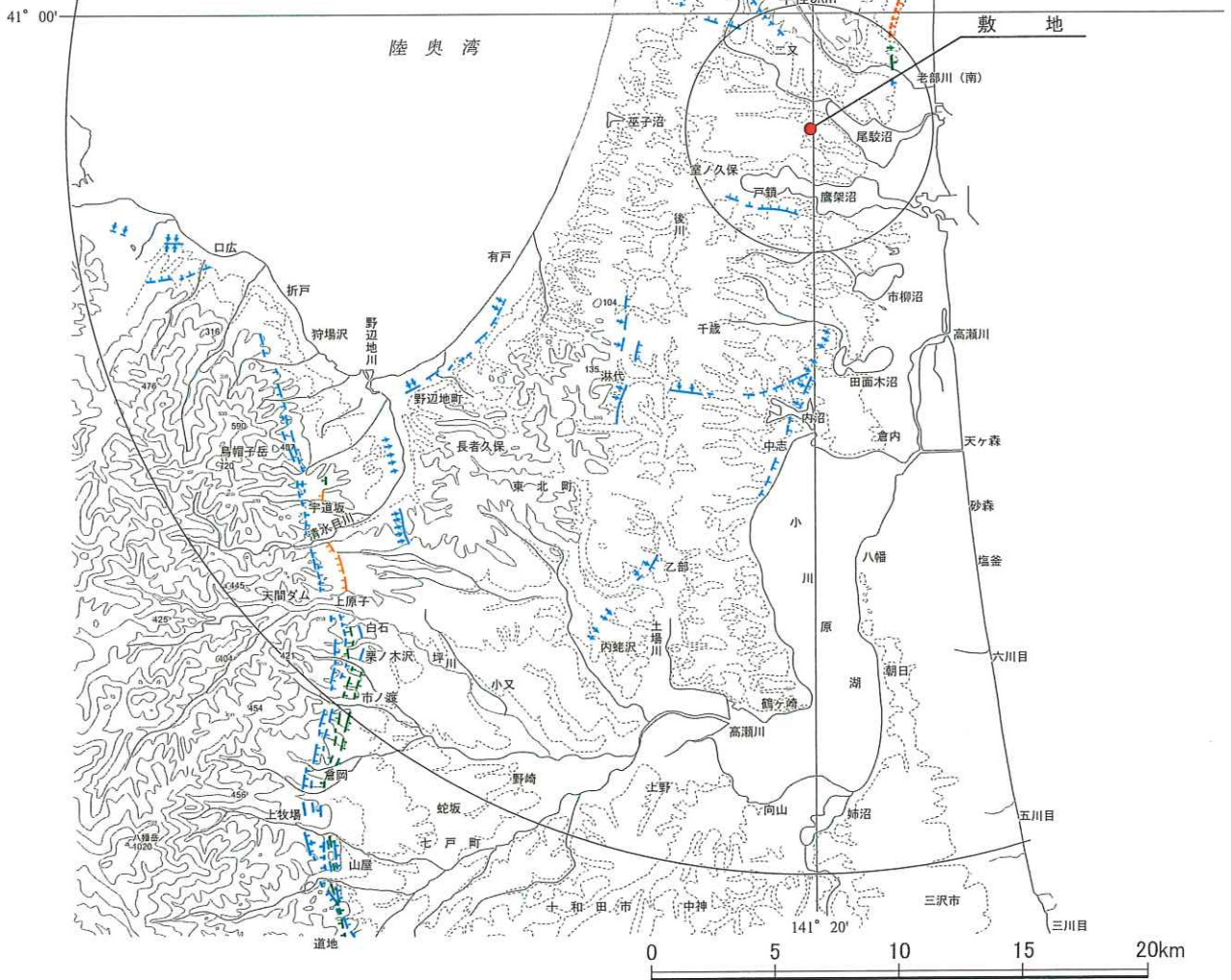
第4.2-7図 敷地周辺陸域のリニアメント・変動地形の分布図
