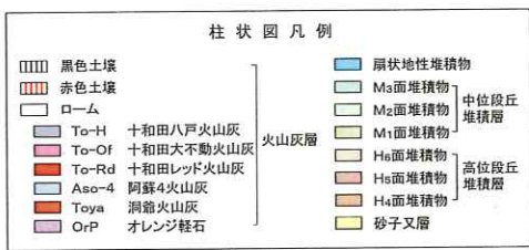
第4.2-31図 野辺地断層北方の地形断面図
