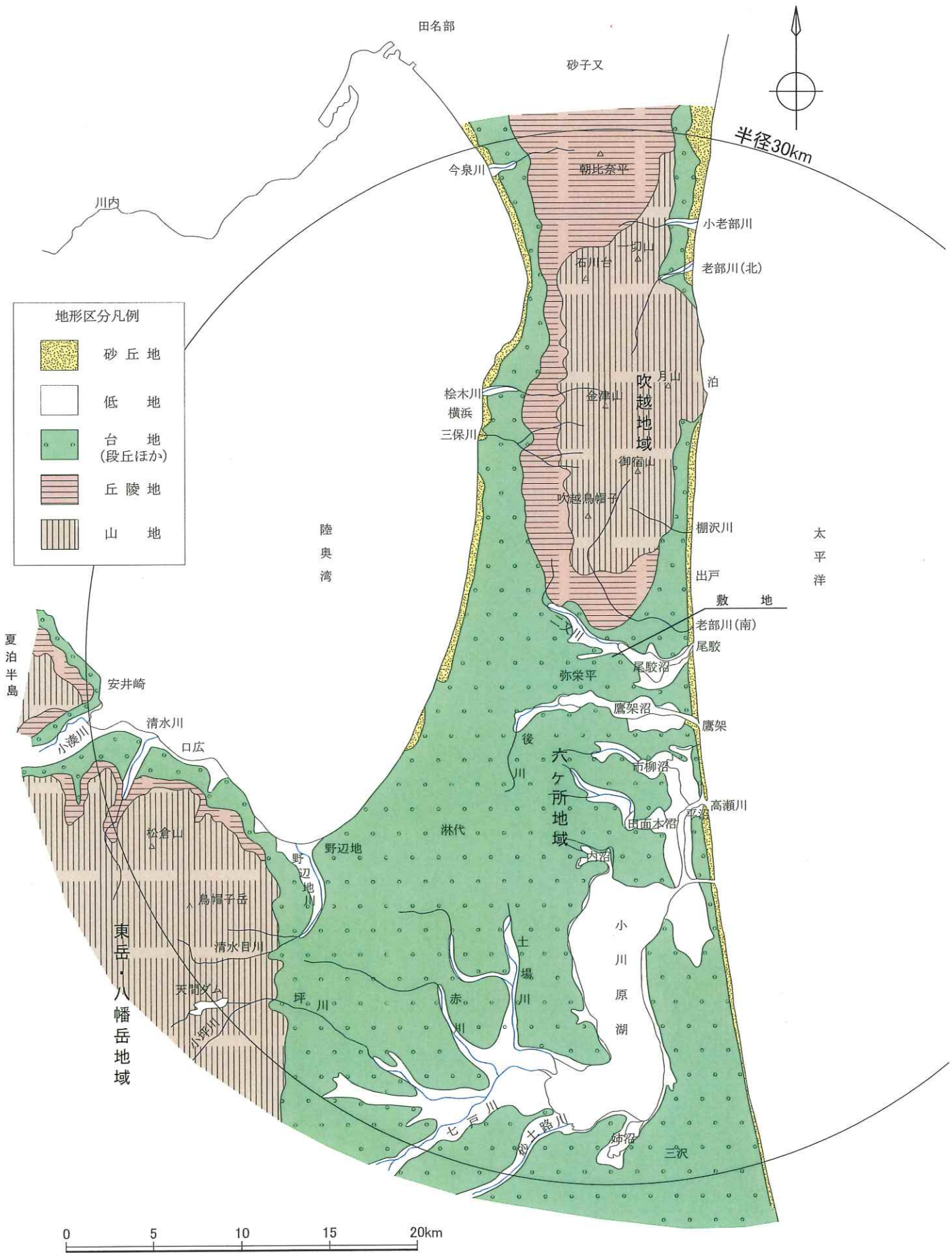
第4.2-2図 敷地周辺陸域の地形区分図
