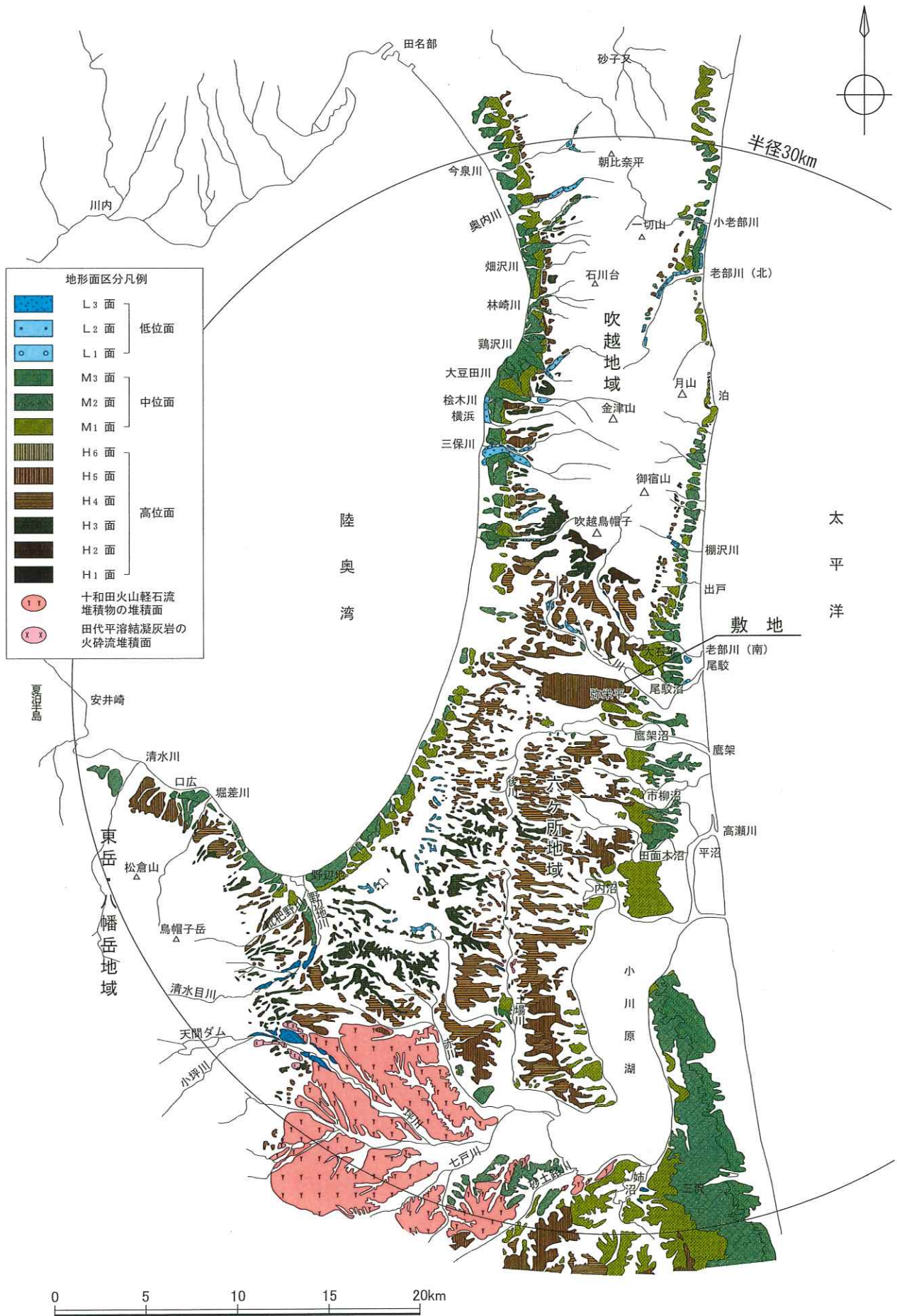
第4.2-6図 敷地周辺陸域の地形面区分図
