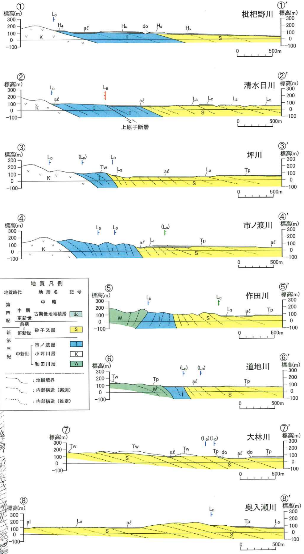
第4.2-47図(1) 野辺地断層から七戸西方断層にかけての地質構造詳細図
