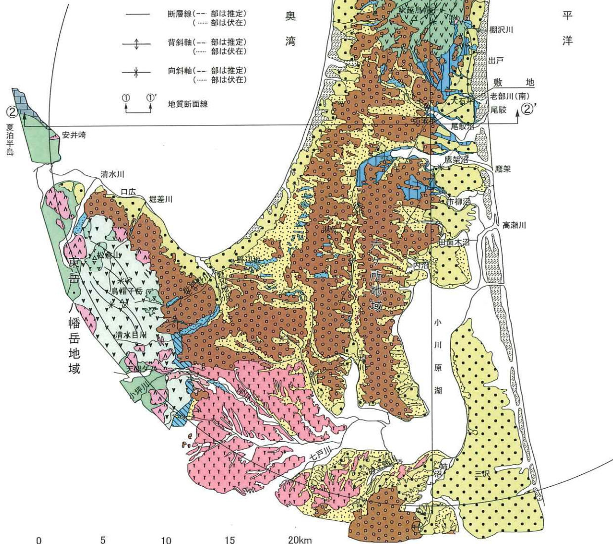
第4.2-3図 敷地周辺陸域の地質平面図
