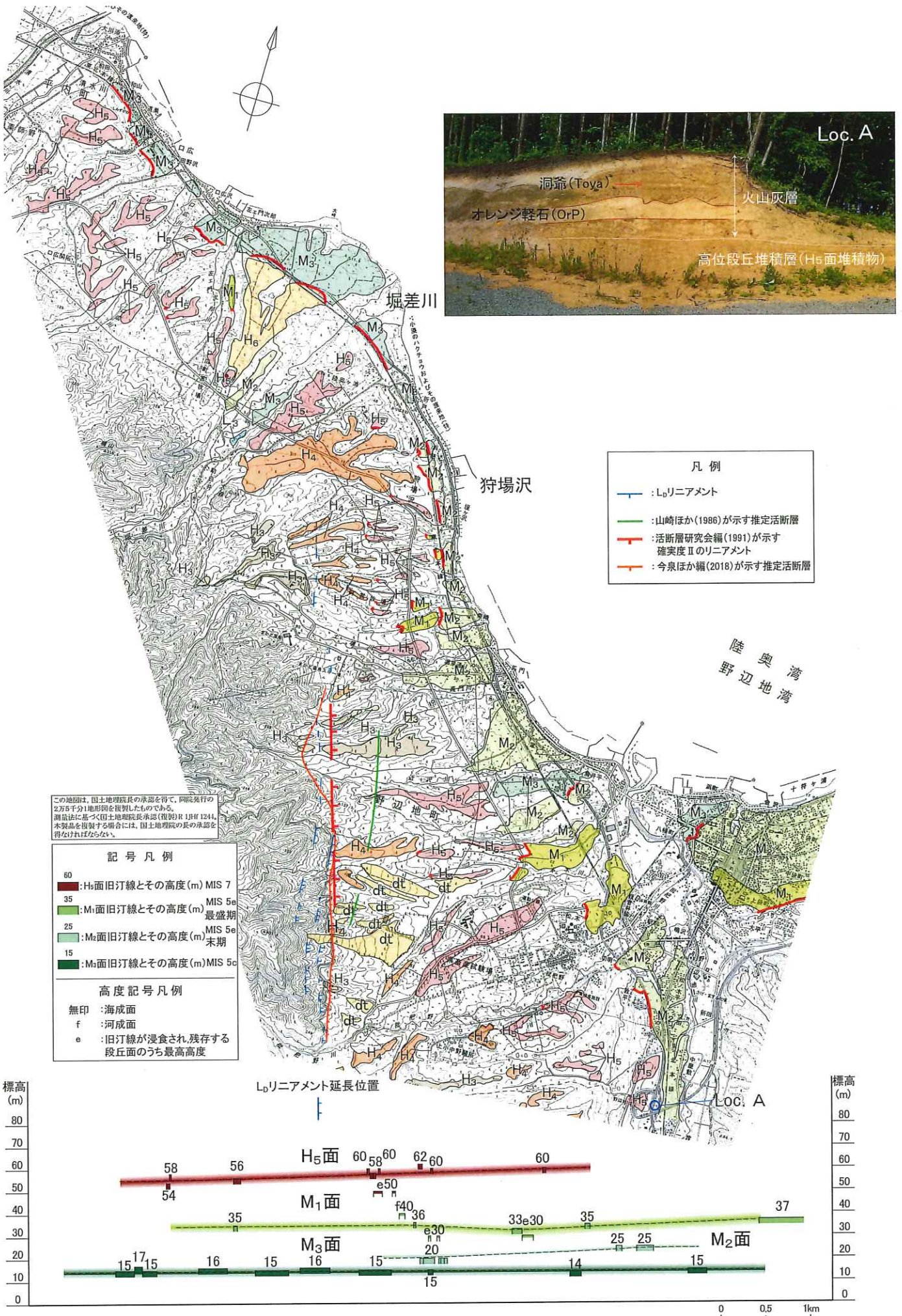
第4.2-30図 野辺地断層北方延長位置の旧汀線高度分布図
