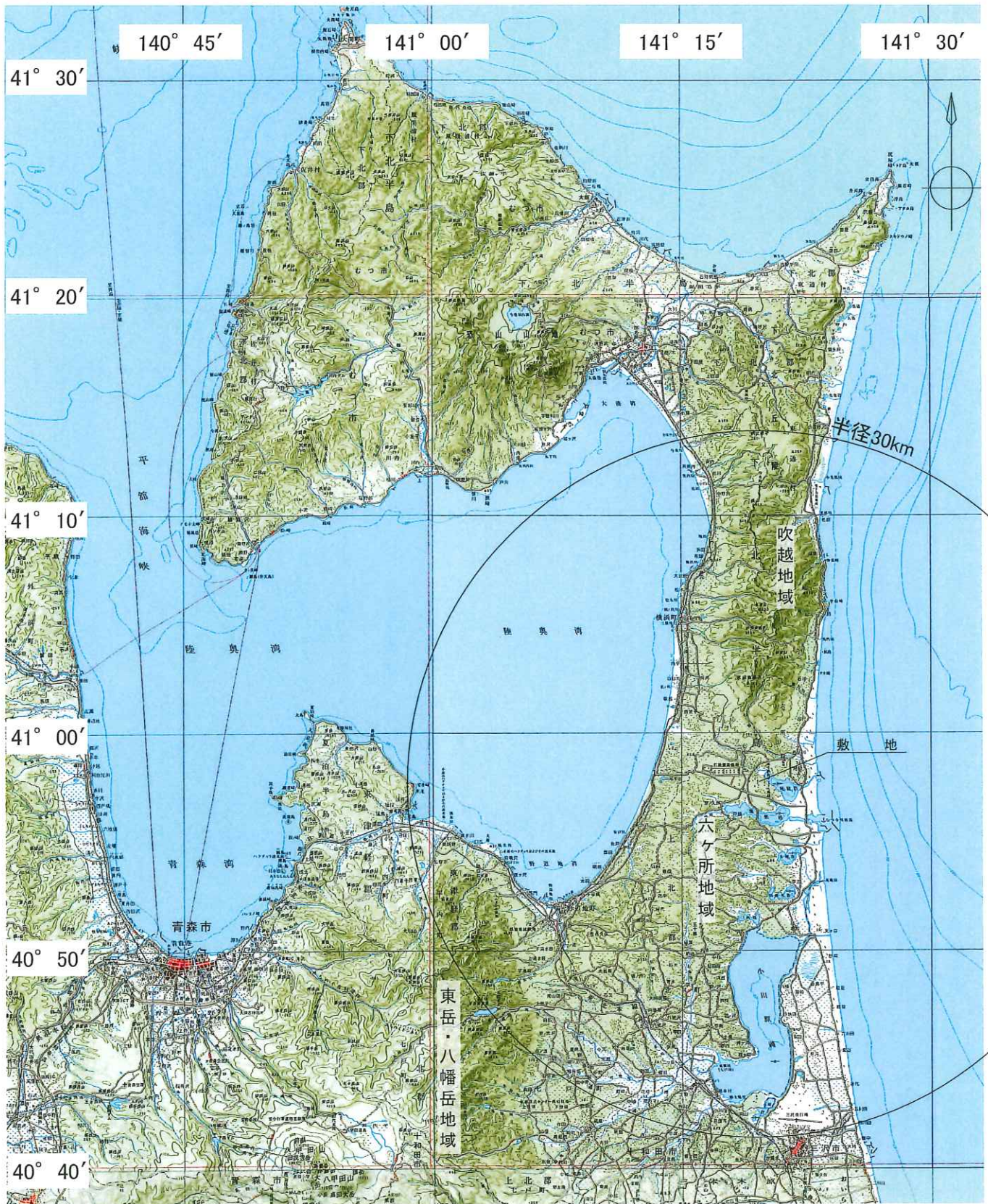
第4.2-1図 敷地周辺陸域の地形図
