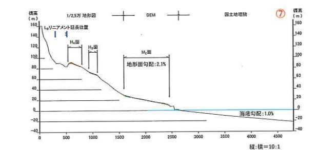
第4.2-31図 野辺地断層北方の地形断面図
