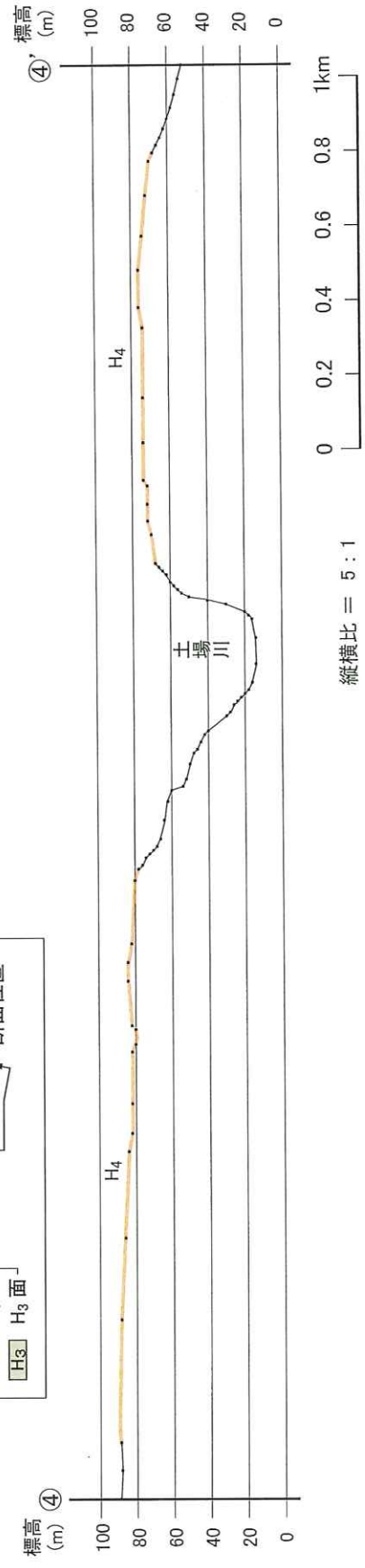
第4.2-51図(3) 後川-土場川断層周辺の地形断面図 (④測線) 4-4-296
