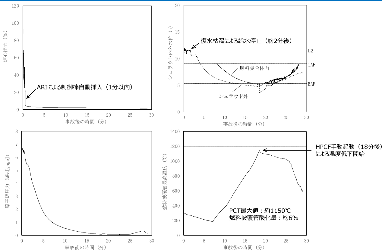
図 TRACGによるRHR出口配管破断（給水継続）+デジタル安全保護系CCF解析例（18分後HPCF手動起動を想定）
