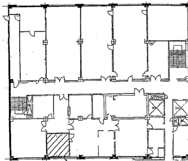
事務本館 3階
