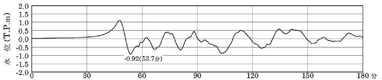
西山断層帯
