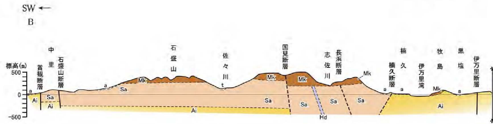
【B-B'断面図】
