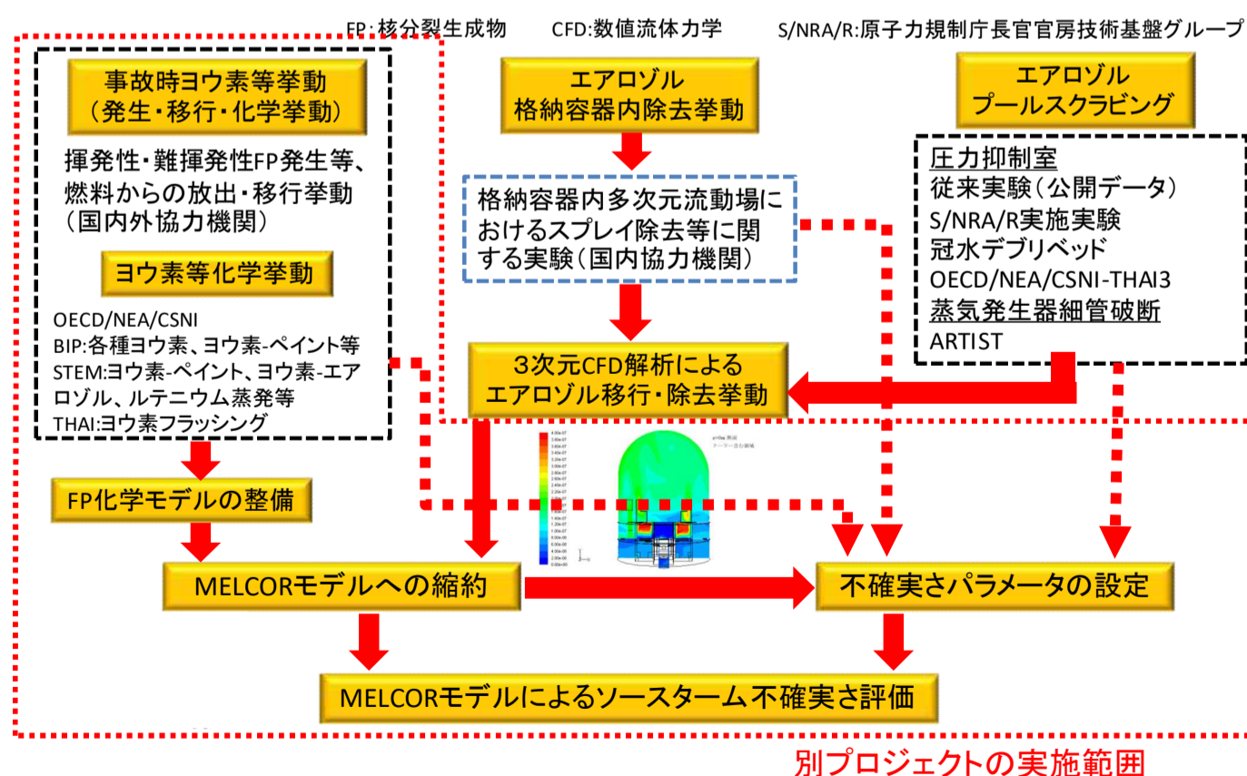
図4 放射性物質生成・移行・除去モデル開発
