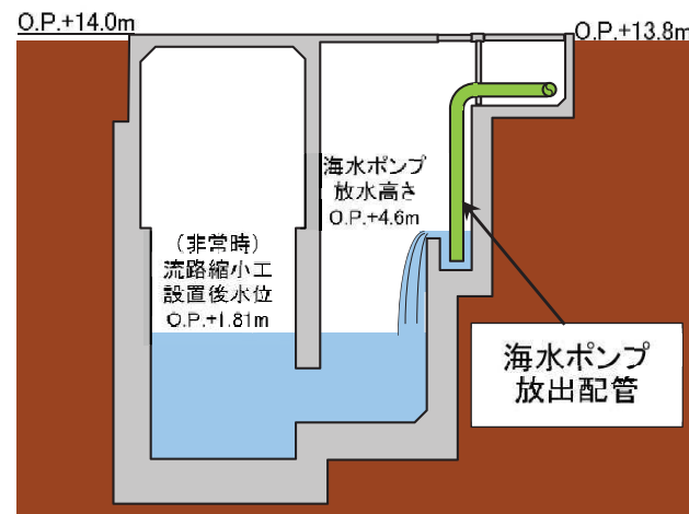
B-B断面図
